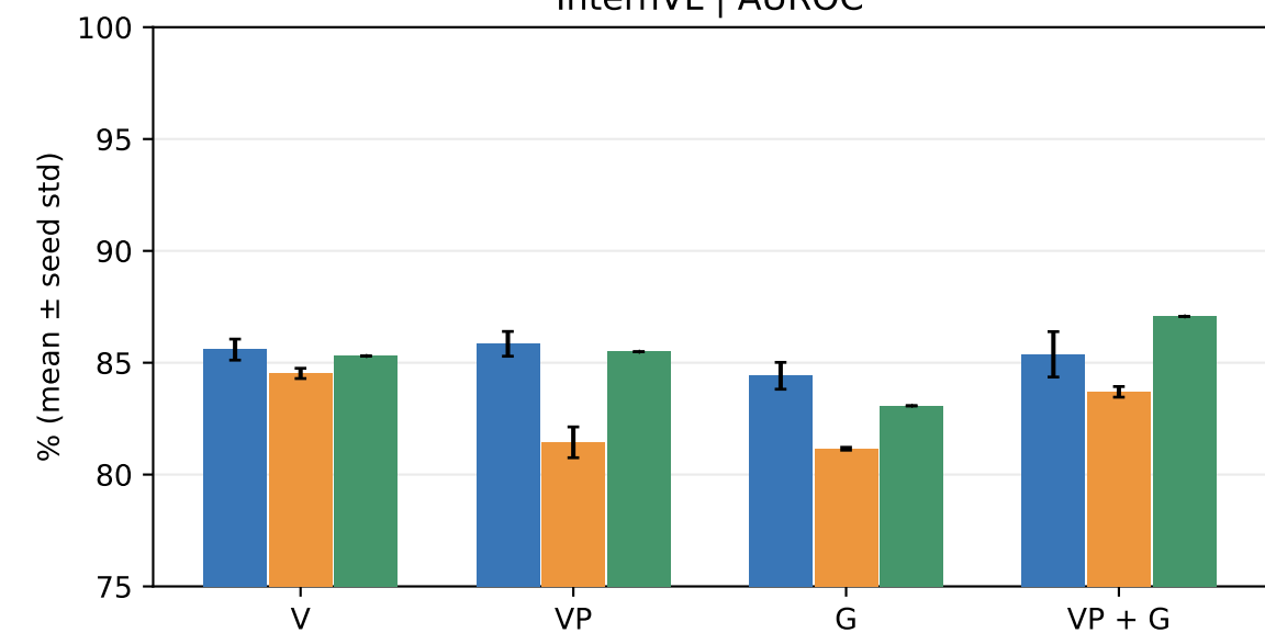
InternVL | AUROC
