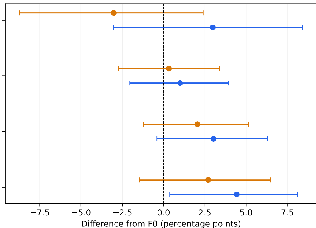
HALL-AUPR
