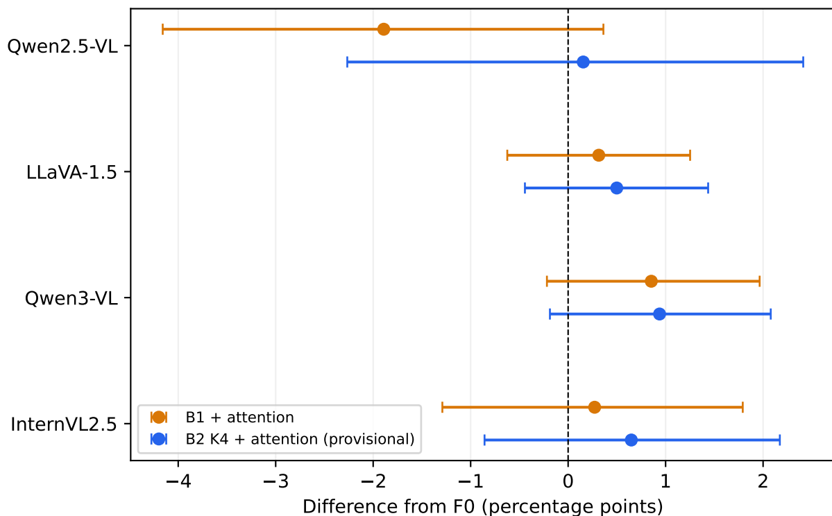
AUROC
