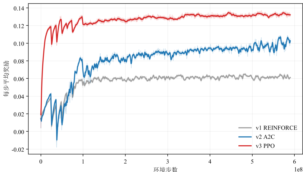
图 17: 同一个任务、同一份预算，三个算法的学习曲线。横轴用环境步数而不是墙钟——墙钟依赖当时跑在哪张卡上、有没有别的任务在抢，换台机器数字就变；环境步数是算法本身消耗的经验量，跨机器可比。浅色是逐迭代原始值，深色是滑动平均。 纵轴是训练时记的平均奖励。 v2/v3 那两条含一项 v1 没有的超时价值补偿（实测 +7.3%），所以三条线之间比的是形状与收敛快慢，绝对高低看上面那张评测表。
