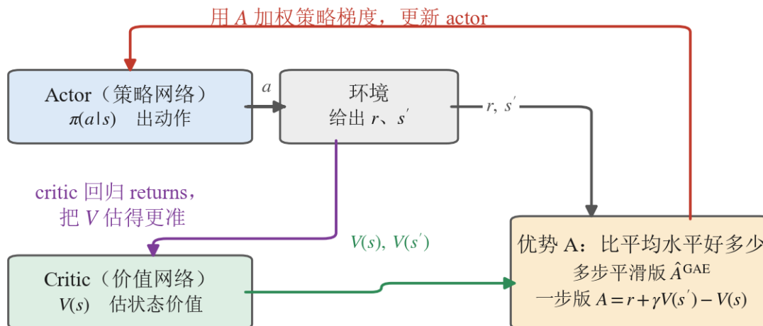
图 12: actor 与 critic 各自在做什么。critic 回归 returns 把 V 估准，两个 V 相减得到优势 A （一步版 A = r + \gamma V(s') - V(s) ，本篇用的是多步平滑的 GAE），再拿 A 去加权策略梯度更新 actor。
