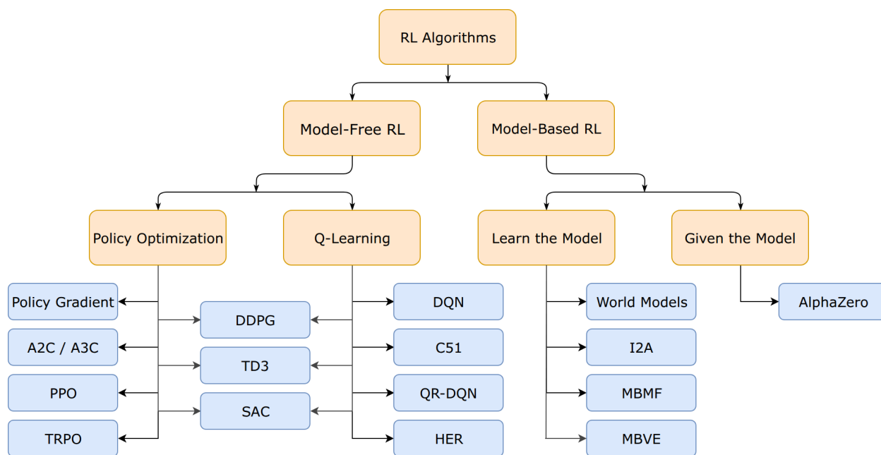
图 7: 方法分类地图 (取自 OpenAI Spinning Up)。它画出了本节前两个划分: 先分「学不学环境模型」, 无模型那一支再分「基于策略」与「基于价值」。本讲走的是左下角那条——无模型·基于策略, 图里的 Policy Gradient → A2C/A3C → PPO 正好是第 5-7 节的三级阶梯。第三个划分 (on-policy / off-policy) 不在这张图上, 见 3.4 节。
