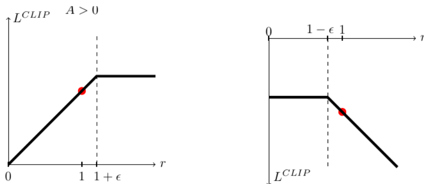
图 15: clip 目标的形状（PPO 原论文图 1）。横轴是概率比值 r ，纵轴是单个样本的目标值。左：优势为正时， r 涨过 1 + \epsilon 之后曲线变平——再往那个方向推没有额外收益。右：优势为负时， r 跌破 1 - \epsilon 之后同样变平。红点是 r = 1 （新旧策略相同）的位置。
