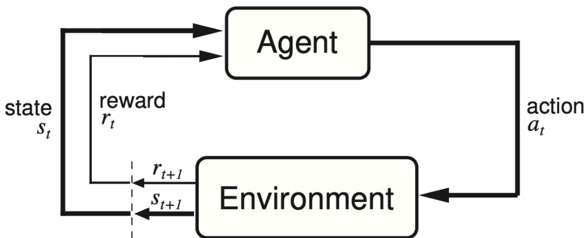
图 4: 智能体与环境的闭环：环境给出状态 s_t ，智能体出动作 a_t ，环境回一个新状态 s_{t+1} 和一个奖励 r_{t+1} 。强化学习与模仿学习的全部差别，就在多出来的那条奖励线上。（图取自 LeRobot 的强化学习教程）
