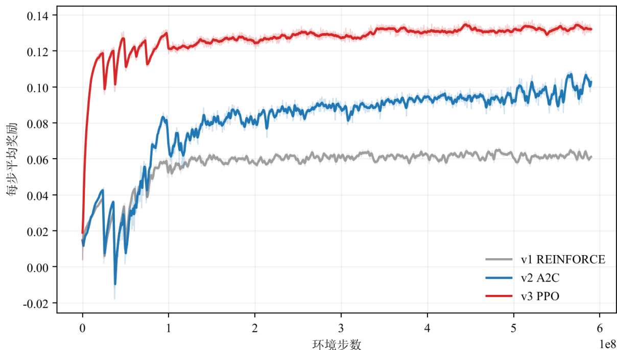
图 16: 同一个任务、同一份预算，三个算法的学习曲线。横轴用环境步数而不是墙钟——墙钟依赖当时跑在哪张卡上、有没有别的任务在抢，换台机器数字就变；环境步数是算法本身消耗的经验量，跨机器可比。浅色是逐迭代原始值，深色是滑动平均。 纵轴是训练时记的平均奖励。 v2/v3 那两条含一项 v1 没有的超时价值补偿（实测 +7.3%），所以三条线之间比的是形状与收敛快慢，绝对高低看上面那张评测表。
