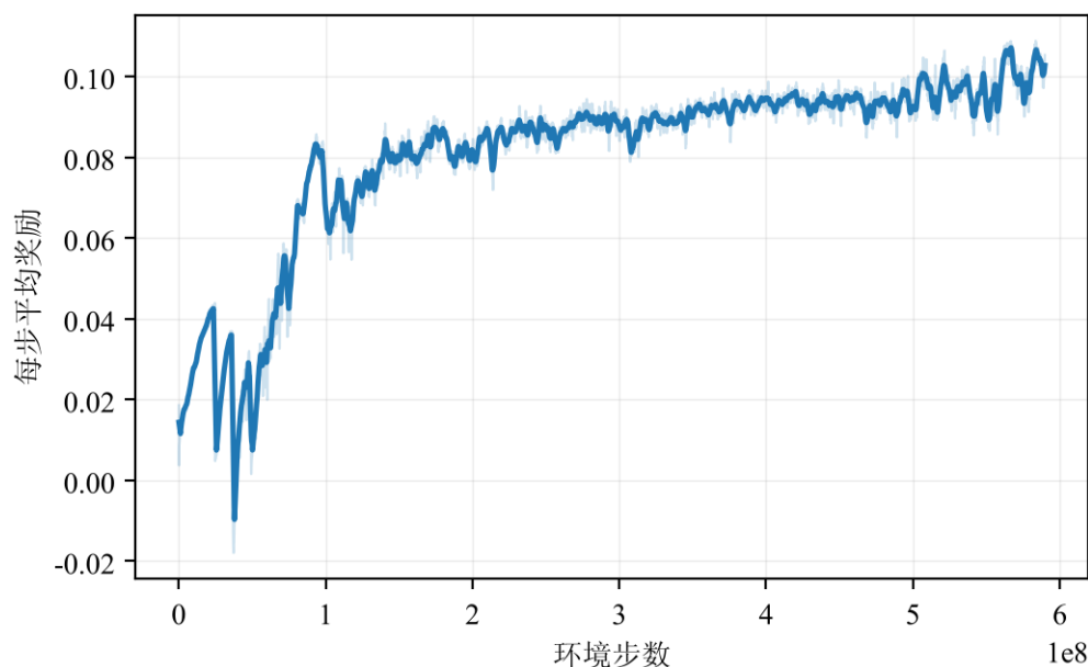
图 13: v2 A2C 的学习曲线。它一路爬到 0.10 以上还没走平，而 v1 在 0.06 就停住了。
