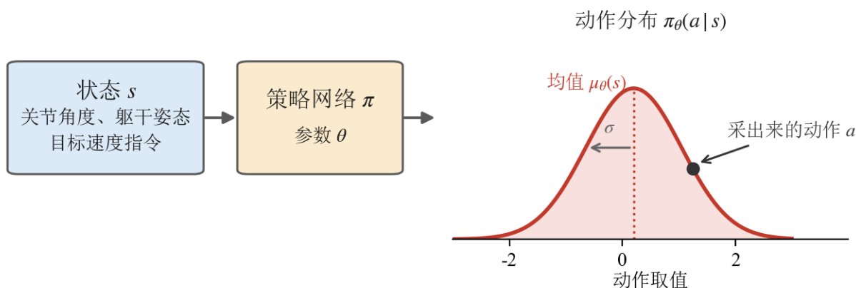
图 5: 策略在连续动作上输出的不是一个数，是一个 分布 ：网络给出均值 \mu_\theta(s) 与标准差 \sigma ，真正执行的 动作 是从这个高斯里采出来的。 \sigma 就是探索的幅度——第 5 节那个熵奖励调的正是它。
