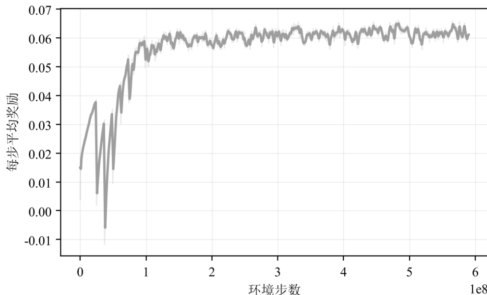
图 10: v1 REINFORCE 的学习曲线。浅色是逐迭代原始值，深色是滑动平均。它确实在学，但爬到 0.06 附近就走平了，而且是彻底走平，不是放慢。
