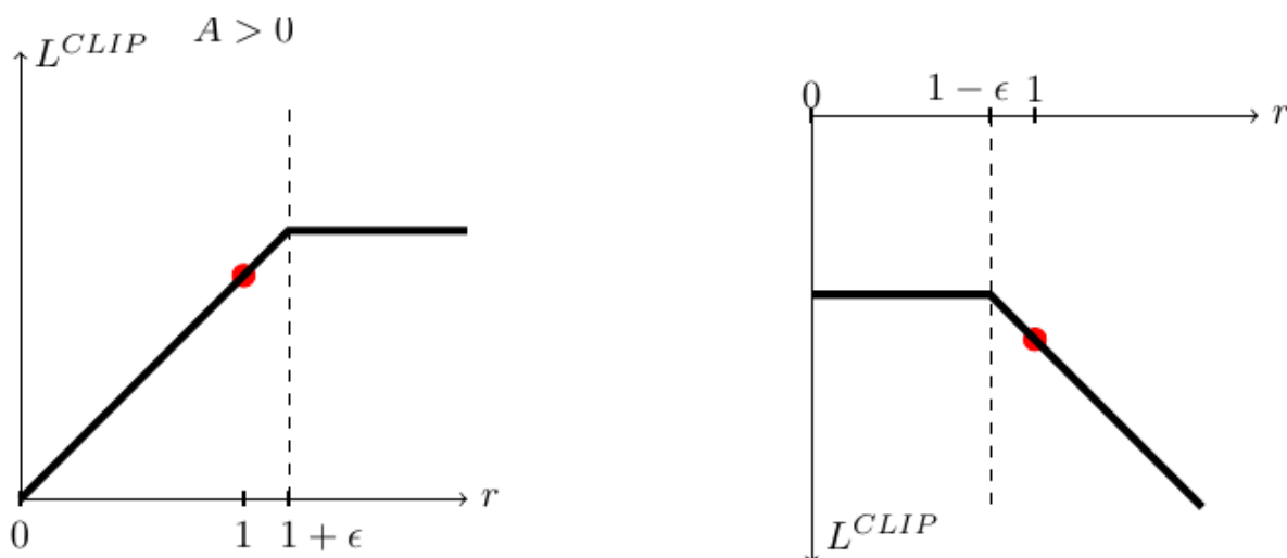
图 17: clip 目标的形状（PPO 原论文图 1）。横轴是概率比值 r ，纵轴是单个样本的目标值。左：优势为正时， r 涨过 1 + \epsilon 之后曲线变平——再往那个方向推没有额外收益。右：优势为负时， r 跌破 1 - \epsilon 之后同样变平。红点是 r = 1 （新旧策略相同）的位置。
