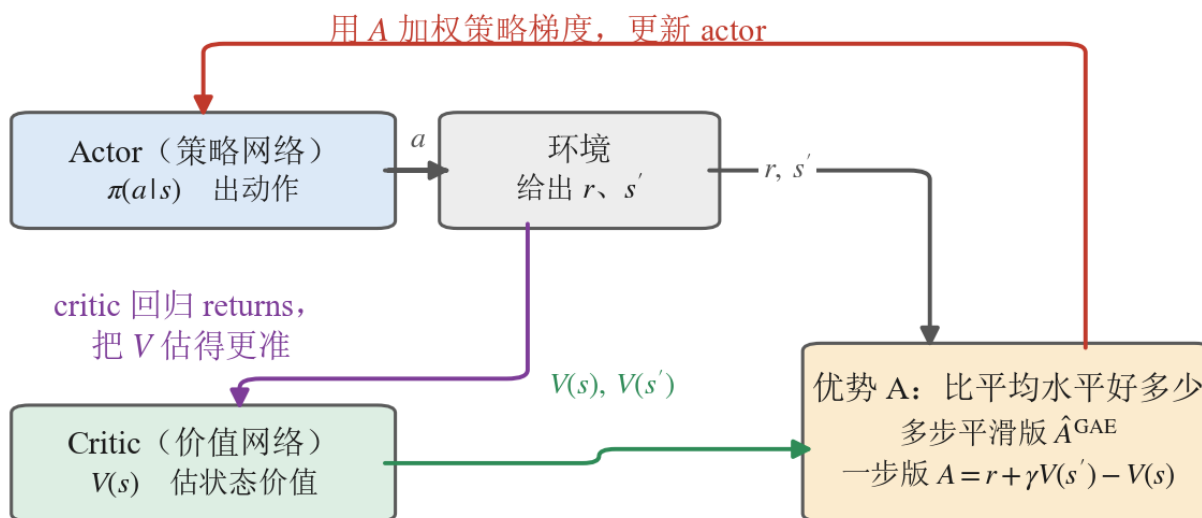
图 14: actor 与 critic 各自在做什么。critic 回归 returns 把 V 估准，两个 V 相减得到优势 A （一步版 A = r + \gamma V(s') - V(s) ，本篇用的是多步平滑的 GAE），再拿 A 去加权策略梯度更新 actor。
