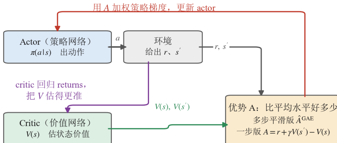
图 11: actor 与 critic 各自在做什么。critic 回归 returns 把 V 估准，两个 V 相减得到优势 A （一步版 A = r + \gamma V(s') - V(s) ，本篇用的是多步平滑的 GAE），再拿 A 去加权策略梯度更新 actor。
