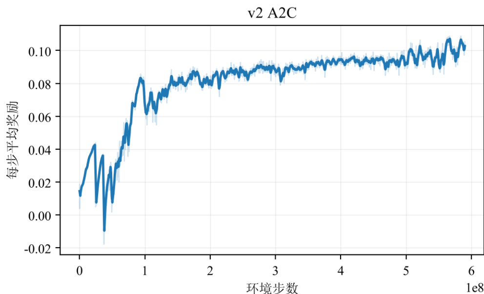
图 12: v2 A2C 的学习曲线。它一路爬到 0.10 以上还没走平，而 v1 在 0.06 就停住了。
