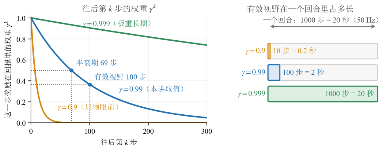
图 5: 折扣因子 \gamma 决定它看多远。左：往后第 k 步的奖励在回报里的权重 \gamma^k ；右：换算成”有效视野在一个回合里占多长”。本篇取 \gamma = 0.99 —— 半衰期 69 步、有效视野约 100 步，而走路一个回合是 1000 步（20 秒 / 50 赫兹）。取 0.9 就只顾眼前 0.2 秒，取 0.999 则把整个回合都算进来。
