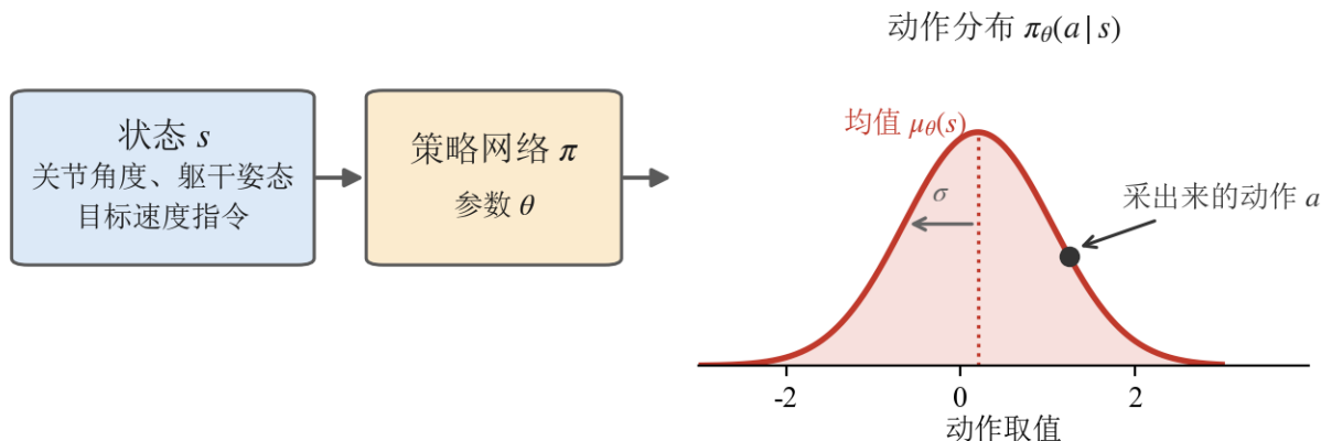
图 4: 策略在连续动作上输出的不是一个数，是一个分布：网络给出均值 \mu_\theta(s) 与标准差 \sigma ，真正执行的动作是从这个高斯里采出来的。 \sigma 就是探索的幅度——第 5 节那个熵奖励调的正是它。
