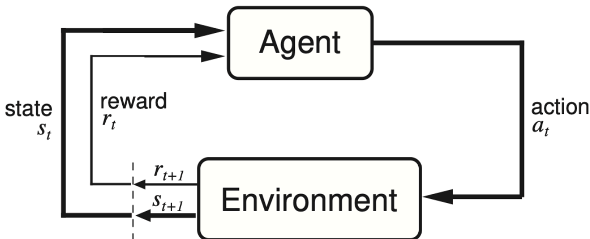
图 3: 智能体与环境的闭环：环境给出状态 s_t ，智能体出动作 a_t ，环境回一个新状态 s_{t+1} 和一个奖励 r_{t+1} 。强化学习与模仿学习的全部差别，就在多出来的那条奖励线上。（图取自 LeRobot 的强化学习教程）
