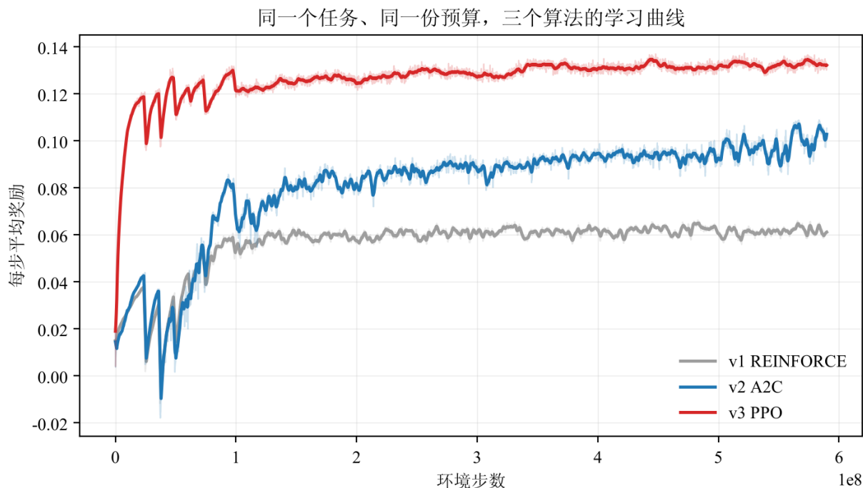
图 14: 同一个任务、同一份预算，三个算法的学习曲线。横轴用环境步数而不是墙钟——墙钟依赖当时跑在哪张卡上、有没有别的任务在抢，换台机器数字就变；环境步数是算法本身消耗的经验量，跨机器可比。浅色是逐迭代原始值，深色是滑动平均。 纵轴是训练时记的平均奖励。 v2/v3 那两条含一项 v1 没有的超时价值补偿（实测 +7.3%），所以三条线之间比的是形状与收敛快慢，绝对高低看上面那张评测表。
