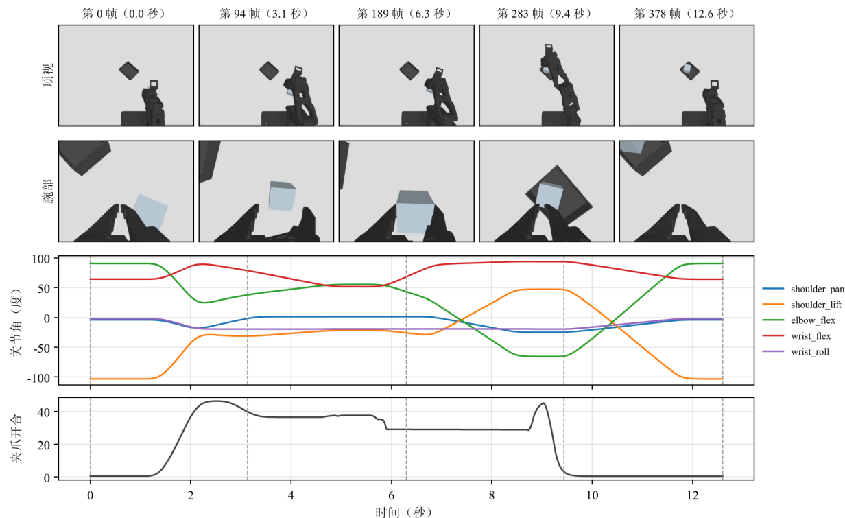
图 11: 仿真 4 cm 方块第 0 集：五个时刻的两路画面，以及同一集逐帧的关节角和夹爪开合
