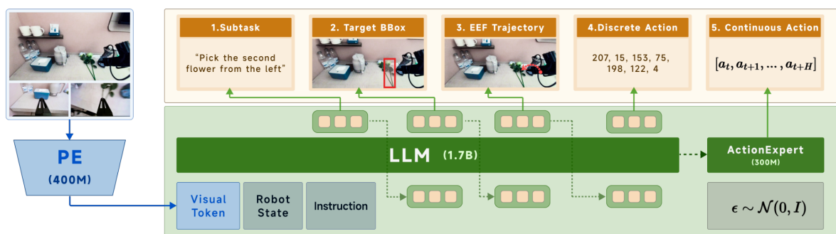
图 6: DM0 的结构: 左侧视觉编码器把多路画面变成视觉 token, 与机器人状态、指令一起送进大语言模型; 右侧动作专家从噪声出发生成连续动作。上方五格是论文里辅助训练用的输出: 子任务、目标框、夹爪轨迹、离散动作与连续动作 (图取自 DM0 论文 [8] 图 2)
