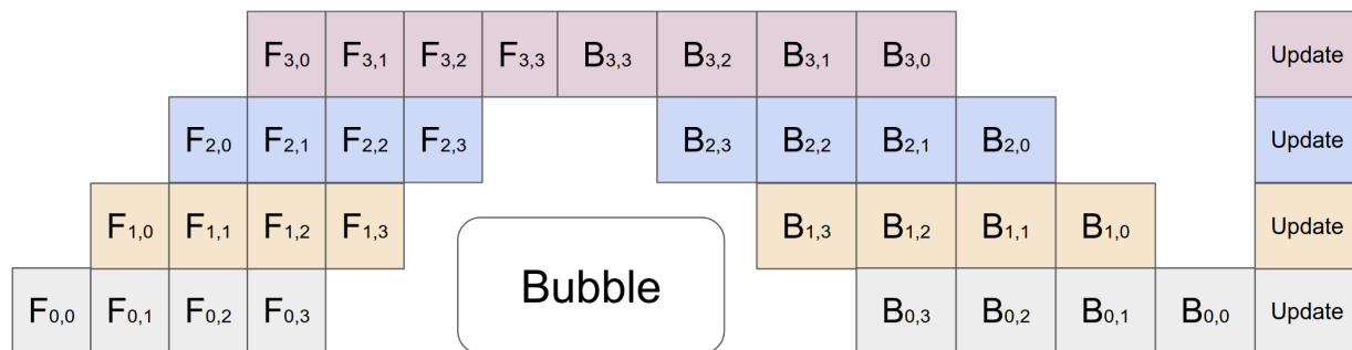
图 28: micro-batch 把流水线填满的调度。一个 batch 被切成 4 个 micro-batch, F_{i,j} 表示第 i 张卡 (行) 算第 j 个 micro-batch 的前向, B_{i,j} 是对应反向。多个 micro-batch 错峰连续喂入, 中间那段每张卡都在同时处理不同的 micro-batch (流水线被填满); 只有最左侧填充阶段和最右侧排空阶段存在空转, 即中间那个 “Bubble” (气泡)。micro-batch 切得越多, 气泡占比越小
