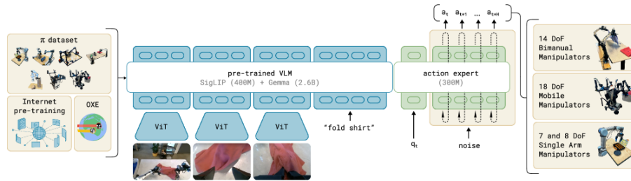
图 34: \pi_0 的框架。左端是训练数据来源—— \pi 自采数据集、互联网预训练语料与 OXE (Open X-Embodiment)；中间是预训练 VLM，标注为 SigLIP (400M) + Gemma (2.6B)，多路相机图各过一个 ViT，与指令“fold shirt”一起进入；右接一个 300M 的动作专家，输入当前关节状态 q_t 和噪声，输出动作块 a_t, a_{t+1}, \dots, a_{t+H} ；最右列出三类目标本体——14 自由度双臂、18 自由度移动操作、7 与 8 自由度单臂。(图取自参考文献 [8])
