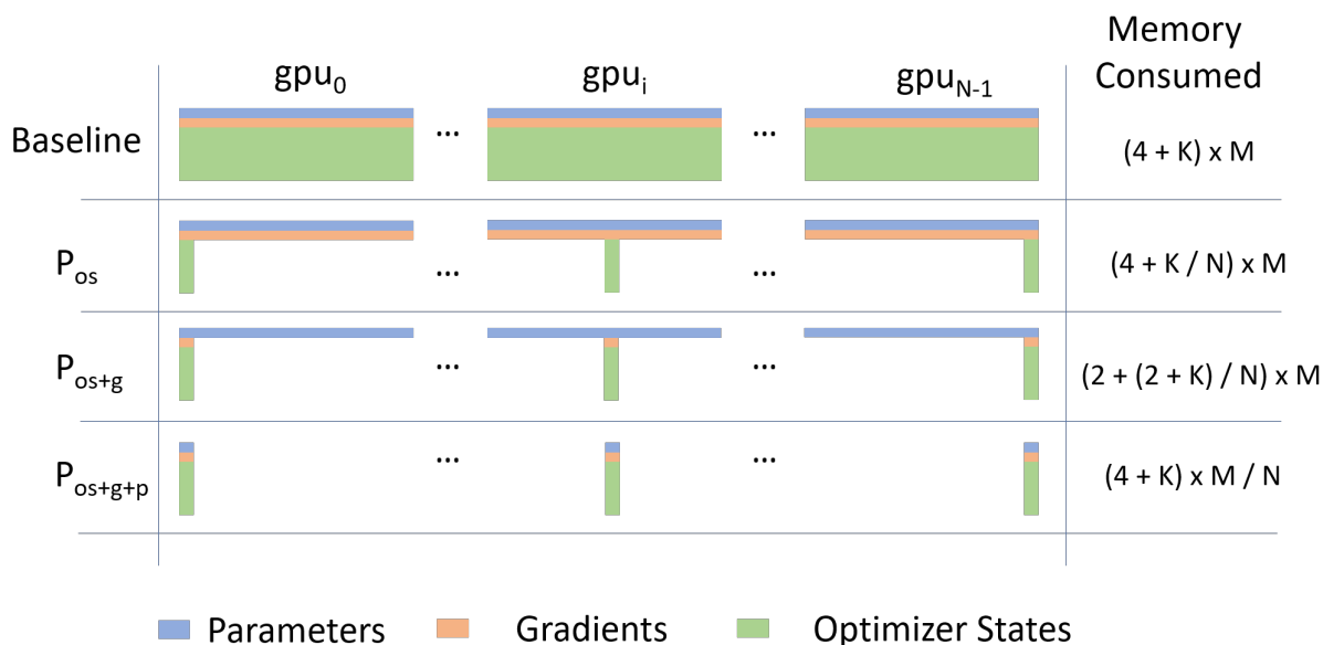
图 23: ZeRO 三阶段分片对比。每一行是一种方案，横向从 gpu_0 到 gpu_{N-1} 是各张卡，柱子里蓝 = 参数、橙 = 梯度、绿 = 优化器状态。最上 Baseline（即 DDP）每张卡存满整份 (4 + K)\Psi ； P_{os} （Stage 1）只把绿色优化器状态沿各卡切开，每卡降到 (4 + K/N)\Psi ； P_{os+g} （Stage 2）再切橙色梯度，降到 (2 + (2 + K)/N)\Psi ； P_{os+g+p} （Stage 3）连蓝色参数也切，每卡只剩 (4 + K)\Psi/N 。图中 K 为优化器状态系数（混合精度 Adam K=12 ）， N 为数据并行度（正文写作 N_d ）；图上把参数量记成 M ，就是正文的 \Psi
