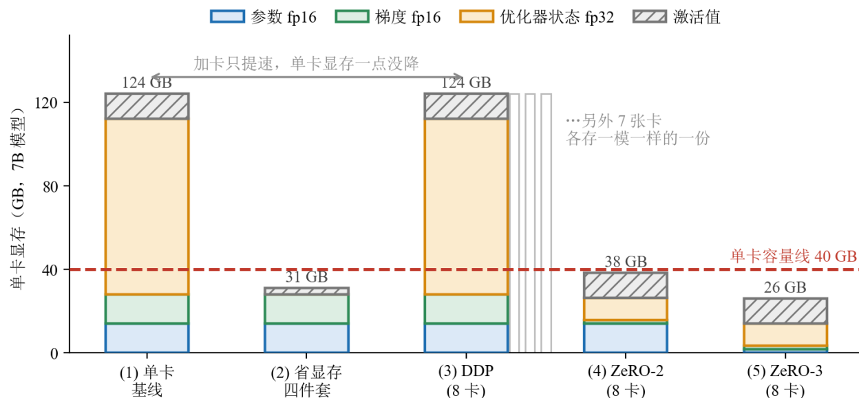
图 29: 一根 7B 模型的单卡显存柱，在五种方案下怎么变。柱子按 4.1.2 节四类吃货分段：参数 fp16 (蓝)、梯度 fp16 (绿)、优化器状态 fp32 (橙)、激活值 (斜纹灰)；红色虚线是标着 40 GB 的单卡容量线。(1) 单卡基线 124 GB，高高在线上；(2) 开省显存四件套后橙色的优化器状态整段消失 (搬到卡外)、斜纹的激活段被梯度检查点压扁，落到 31 GB；(3)DDP 那根柱子仍标着 124 GB，一条双向箭头从 (1) 拉到 (3)、上面写着“加卡只提速，单卡显存一点没降”，右侧几根灰柱注着“另外 7 张卡各存一模一样的一份”；(4)ZeRO-2 把梯度段和优化器段各切成 1/8，降到 38 GB；(5)ZeRO-3 把三段全部切成 1/8，降到 26 GB。图下一行注明：斜纹那段是激活值，随批量与序列长度变，图上只画一个示意高度，其余三段按 16 字节/参数精确折算 (分片按 8 卡算，与 4.4.6 节表里的公式一致)
