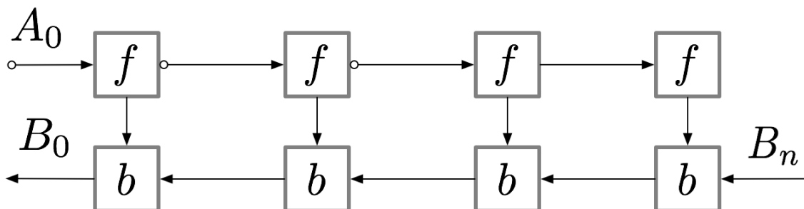
图 21: 梯度检查点下反向传播的执行： f 是前向（重算）、 b 是反向。反向是分段走的：每要算一段的梯度，就先从上游检查点重做一次局部前向 f 补出该段激活，紧接着做这一段的反向 b 。算力上多花了若干次前向重算，换来的是中间激活不必全程驻留显存
