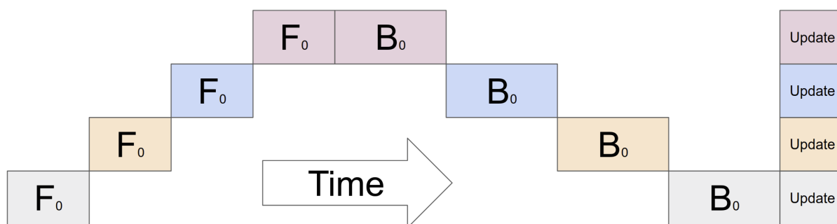
图 27: 朴素按层切的严重空转。横轴是时间，四行是四张卡。一个 batch 进来，前向 F_0 从卡 0（最下行）逐段往上传，同一时刻只有一张卡在算、其余三张闲着；前向走到顶后反向 B_0 再逐段往下回传，依旧一次只有一张卡工作；最后各卡 Update。绝大部分时间各卡都在空转，多卡几乎没换来加速
