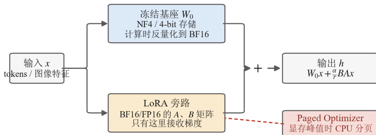
图 12: 输入 x 分成两条支路：上支是冻结基座 W_0 ，标注为 NF4 / 4-bit 存储、计算时反量化到 BF16；下支是 LoRA 旁路，标注为 BF16/FP16 的 A 、 B 矩阵，并注明“只有这里接收梯度”；两支输出相加得到 h = W_0x + \frac{\alpha}{r}BAx 。右下角另有一个分页优化器方框，用虚线指向 LoRA 旁路，标注“显存峰值时 CPU 分页”
