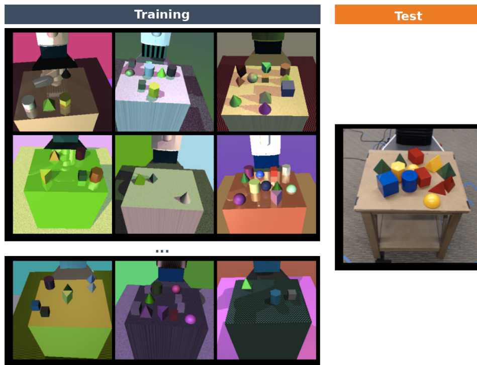
图 30: 左侧“训练”栏是九张仿真渲染图，同一张桌子和同一批几何体在每张里换了一套颜色、纹理、光照和相机角度，桌面从粉到绿到紫无所不有；右侧“测试”栏只有一张真机照片——普通木桌上摆着彩色积木。（图取自参考文献 [27]）
