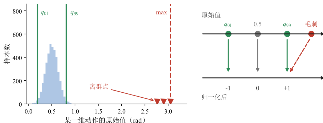
图 11: 左: 直方图里几个离群点把 max 拉得很远, 而 q_{01} / q_{99} 紧贴数据主体; 右: 把 [q_{01}, q_{99}] 线性映射到 [-1, +1] , 超出 q_{99} 的毛刺被截断到 +1
