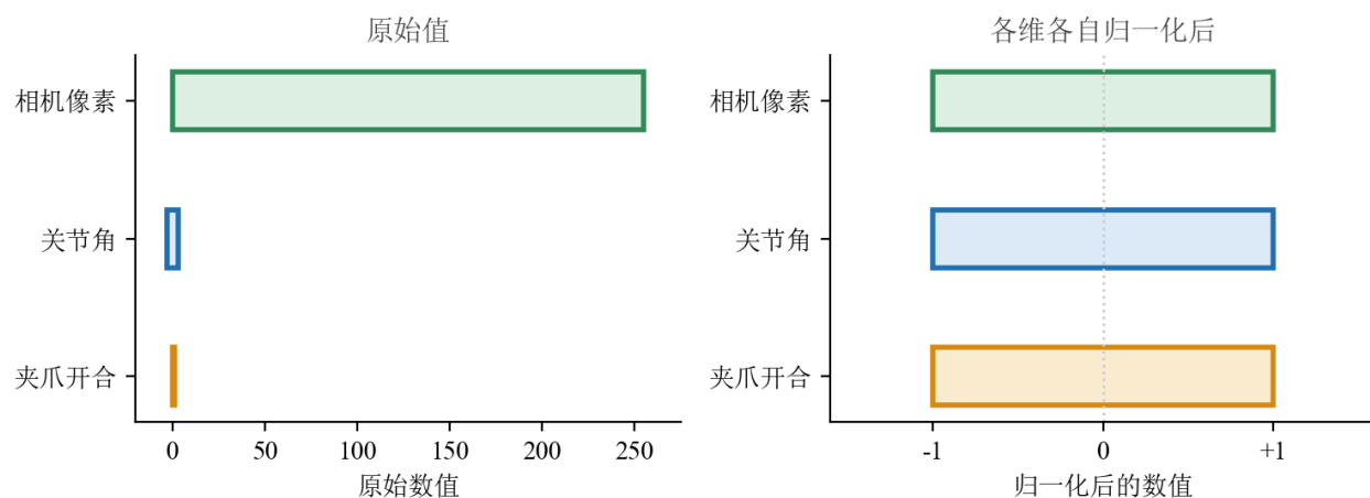
图 10: 左：相机像素、关节角、夹爪开合三种量的原始数值范围相差悬殊；右：各维各自归一化后，统一落到 [-1, +1]
