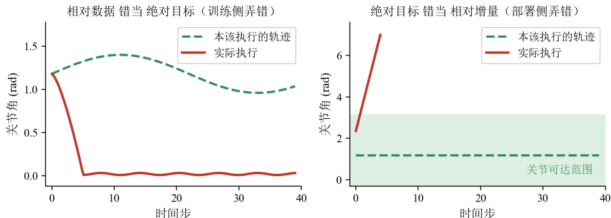
图 9: 左：相对数据被错当成绝对目标训练，网络学会输出“绝对目标约等于 0”，机械臂扎向零位后几乎不动；右：绝对目标被错当成相对增量部署，每步都在当前位置上再累加，关节角一路冲出可达范围
