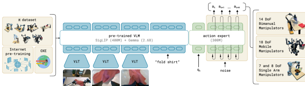
图 13: \pi_0 框架总览：视觉-语言骨干处理图像与语言指令，较小的动作专家以连续方式输出机器人动作
