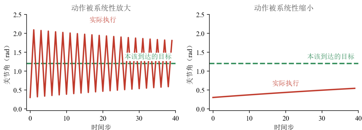
图 12: 左: 动作被系统性放大, 每步都迈过头、围绕目标来回过冲, 看起来在“抖”; 右: 动作被系统性缩小, 每步只挪一点点、迟迟够不到目标, 看起来“不动”。两图里绿色虚线都是本该到达的目标
