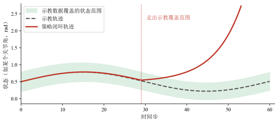
图 7: 绿色带是示教数据覆盖过的状态范围；策略的闭环轨迹起初只比示教偏一点点，一旦走出绿色带、进入模型没见过的状态，预测越来越不可靠，误差加速放大
