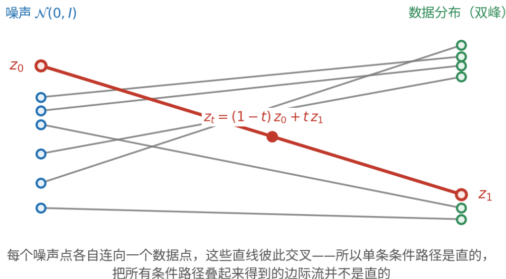
图 12: 左列是采到的噪声样本，右列是数据集里的样本（画成双峰）。同一下标的两个点配成一条 条件路径 ，图里画了 7 条：每个噪声点各自连向一个数据点，端点是独立采样再配对的，所以这些直线彼此交叉。红色那条被高亮出来，标出 z_0 、 z_1 与它们之间的插值点 z_t （本书自绘）
