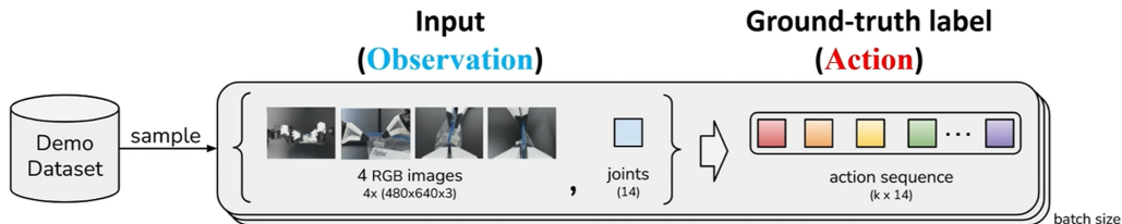
图 5: 训练过程 Step 1: VAE Encoder
