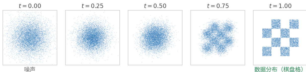
图 11: 五格从左到右是 t = 0, 0.25, 0.5, 0.75, 1 。 t = 0 是标准正态噪声, t = 1 是棋盘格数据分布, 中间三格是 z_t = (1-t)z_0 + tz_1 的边际分布——注意结构不是最后一步突然出现的, t = 0.75 时格子的轮廓已经显形 (本书自绘: 直接按插值式采样画出解析的概率路径, 未训练模型)
