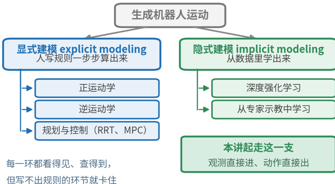
图 1: 生成机器人运动分成两支：左支显式建模，下挂正运动学、逆运动学、规划与控制（RRT、MPC）三类人写规则的方法；右支隐式建模，下挂深度强化学习与从专家示教中学习。右支底下那个加粗的绿框标出了本讲的落点——观测直接进、动作直接出（本书自绘）
