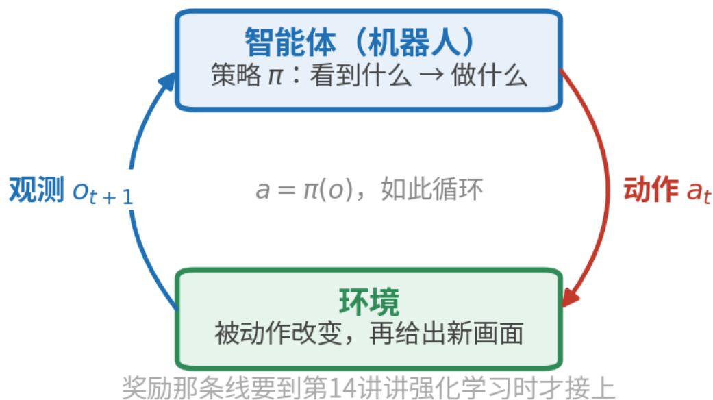
图 4: 智能体与环境只有两条边的闭环：智能体（策略 \pi ）看到观测就给出动作 a_t ，动作作用到环境上，环境被改变后返回新的观测 o_{t+1} ，如此循环（本书自绘）
