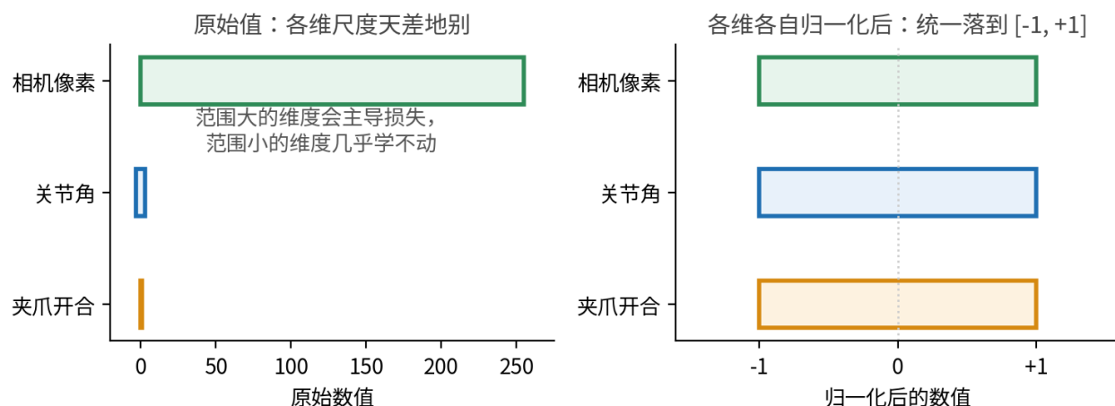
图 11: 左：相机像素、关节角、夹爪开合三种量的原始数值范围相差悬殊；右：各维各自归一化后，统一落到 [-1, +1] （本书自绘）
