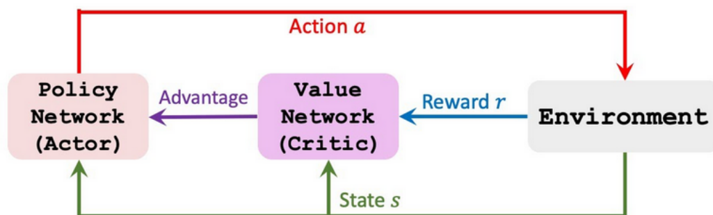
图 11: 占位图 (出处: https://www.paddlepaddle.org.cn/documentation/practices/reinforcement_learning/advantage_actor_critic.html , 许可未确认), 待按此重画。A2C 的骨架是一个环: 环境给出状态 s (下方绿线, 同时进两个网络), 策略网络 (Actor) 据此出动作 a (上方红线) 作用回环境, 环境给出的奖励 r (蓝线) 进价值网络 (Critic), Critic 算出的优势 (Advantage, 紫线) 再回到 Actor 手里。图上写的是 Value Network (价值网络) 而不是 Q 网络, 与本讲 critic 估 V(s) 的口径一致
