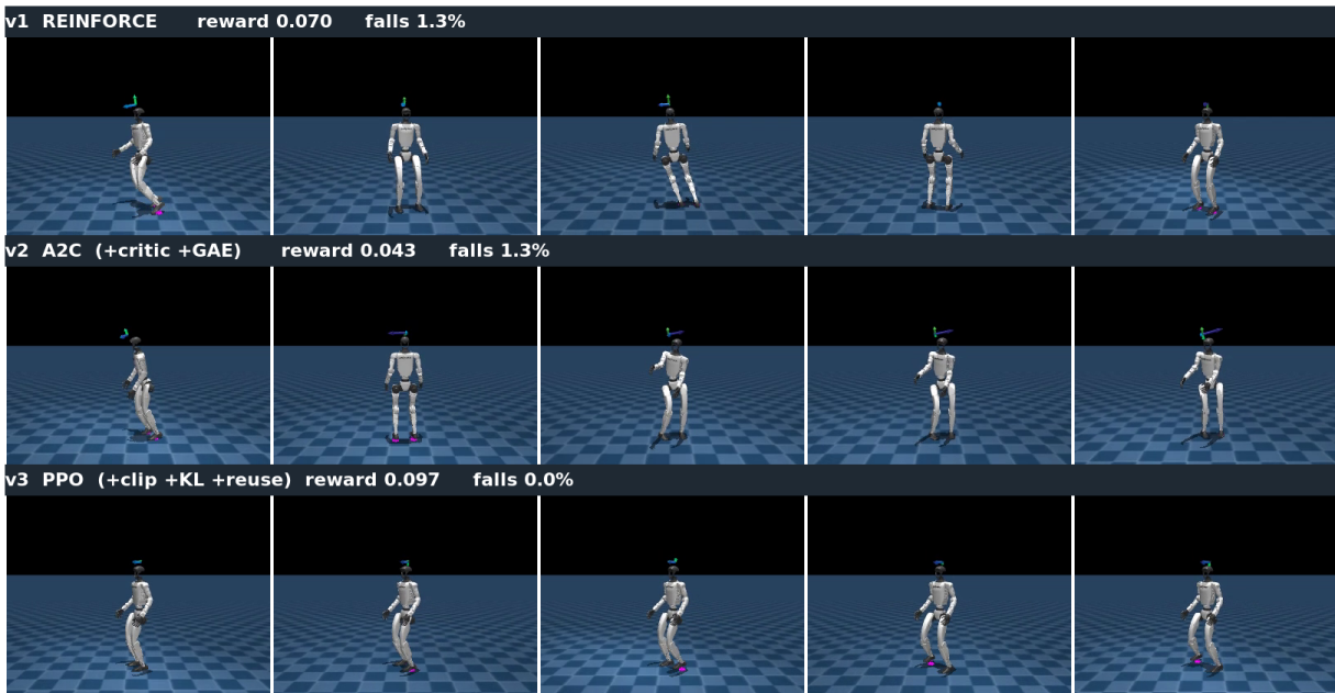
图 15: G1 行走三算法 rollout 对照，每行从左到右是同一段时间内的关键帧，从上到下依次为 v1 REINFORCE、v2 A2C、v3 PPO；各行标题上印着该版本的评测奖励与摔倒率。v3 全程直立稳定，6400 个评测步里一次都没倒
