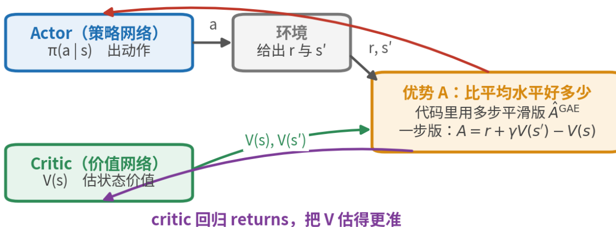
图 12: A2C 的 Actor-Critic 分工: actor (策略网络) 出动作, critic (价值网络) 估状态价值、帮 actor 算优势。图里按通路性质分了三色——灰色是前向的数据流, 绿色是 critic 把 V 供给优势计算, 红色与紫色是两条各自独立的训练回流 (红的更新 actor, 紫的更新 critic)。优化主体仍是策略, critic 只当参照物
