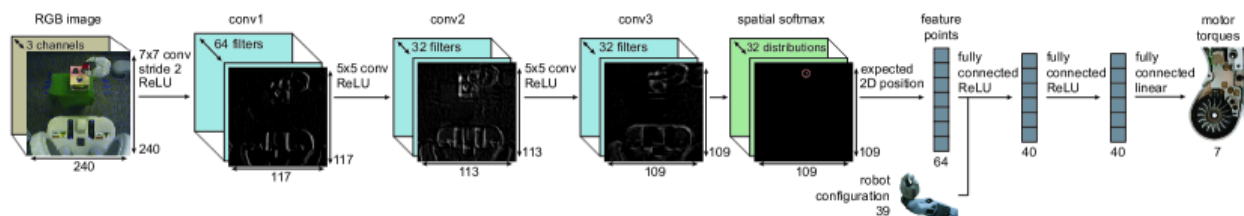
图 3: Levine 视觉运动策略：RGB 图像经卷积与空间特征点提取，直接映射到电机扭矩
