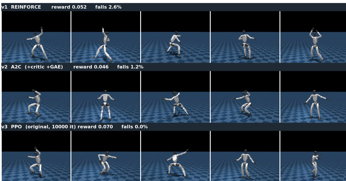
图 16: G1 动作跟随三算法 rollout 对照，每行从左到右是同一段时间内的关键帧，从上到下依次为 v1 REINFORCE、v2 A2C、v3 PPO: v3 做出干净协调的武术姿态（宽马步、抬臂出击）且从不摔倒，v1/v2 明显跟不住参考、东倒西歪
