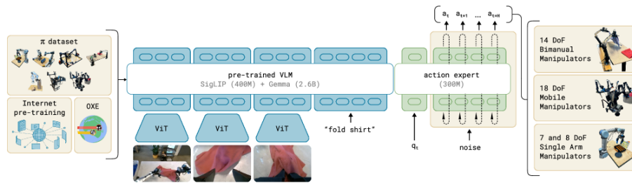
图 37: \pi_0 的框架。左端是训练数据来源—— \pi 自采数据集、互联网预训练语料与 OXE (Open X-Embodiment)；中间是预训练 VLM，标注为 SigLIP (400M) + Gemma (2.6B)，多路相机图各过一个 ViT，与指令“fold shirt”一起进入；右接一个 300M 的动作专家，输入当前关节状态 q_t 和噪声，输出动作块 a_t, a_{t+1}, \dots, a_{t+H} ；最右列出三类目标本体——14 自由度双臂、18 自由度移动操作、7 与 8 自由度单臂。(图取自参考文献 [8])
