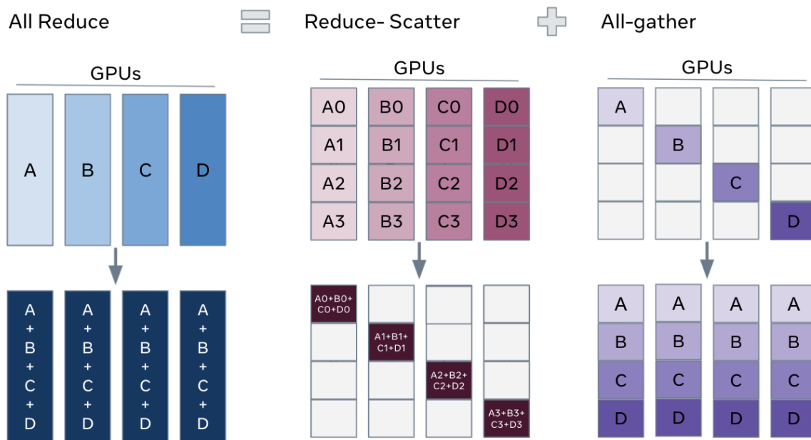
图 25: 同一批要在各卡间对齐的数据, 三种集合通信的差别: 左边 All-Reduce 把各卡的整份数据规约 (求和) 后让人手一份相同结果, 是 DDP 同步梯度用的; 中间 Reduce-Scatter 先按分片求和、但每张卡只收下自己负责的那一片求和结果 (每卡只留 1/N 的规约梯度); 右边 All-Gather 把各卡手里的分片拼接起来, 让每张卡集齐完整的一份。ZeRO/FSDP 正是用 all-gather 临时拼回完整参数、用 reduce-scatter 把梯度规约后直接切片落到各卡
