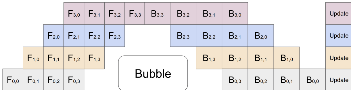
图 31: micro-batch 把流水线填满的调度。一个 batch 被切成 4 个 micro-batch, F_{i,j} 表示第 i 张卡 (行) 算第 j 个 micro-batch 的前向, B_{i,j} 是对应反向。多个 micro-batch 错峰连续喂入, 中间那段每张卡都在同时处理不同的 micro-batch (流水线被填满); 只有最左侧填充阶段和最右侧排空阶段存在空转, 即中间那个 “Bubble” (气泡)。micro-batch 切得越多, 气泡占比越小
