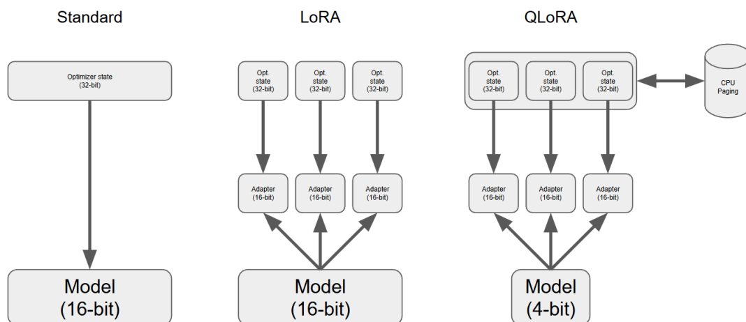
图 17: 标准微调、LoRA、QLoRA 三种方式的显存构成对照：基座权重、适配器与优化器状态各占多少、各处是什么精度
