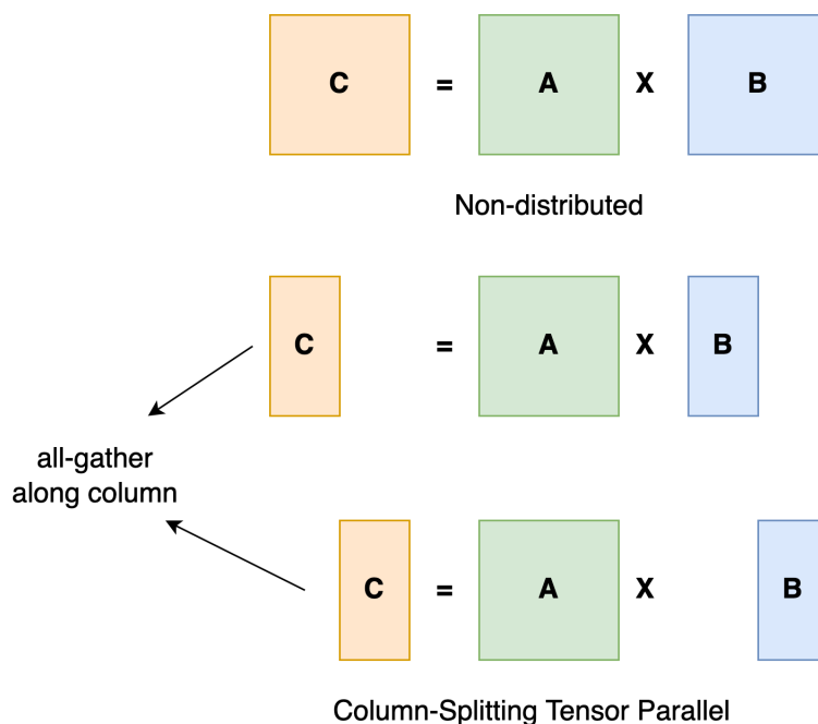
图 19: 模型并行 (张量并行) 示意: 上方是非分布式的整块矩阵乘 C = A \times B ; 下方是按列切分 (Column-Splitting) 后, 每张卡只算结果的一部分列, 再通过 all-gather 沿列方向把各卡的局部结果拼成完整的 C
