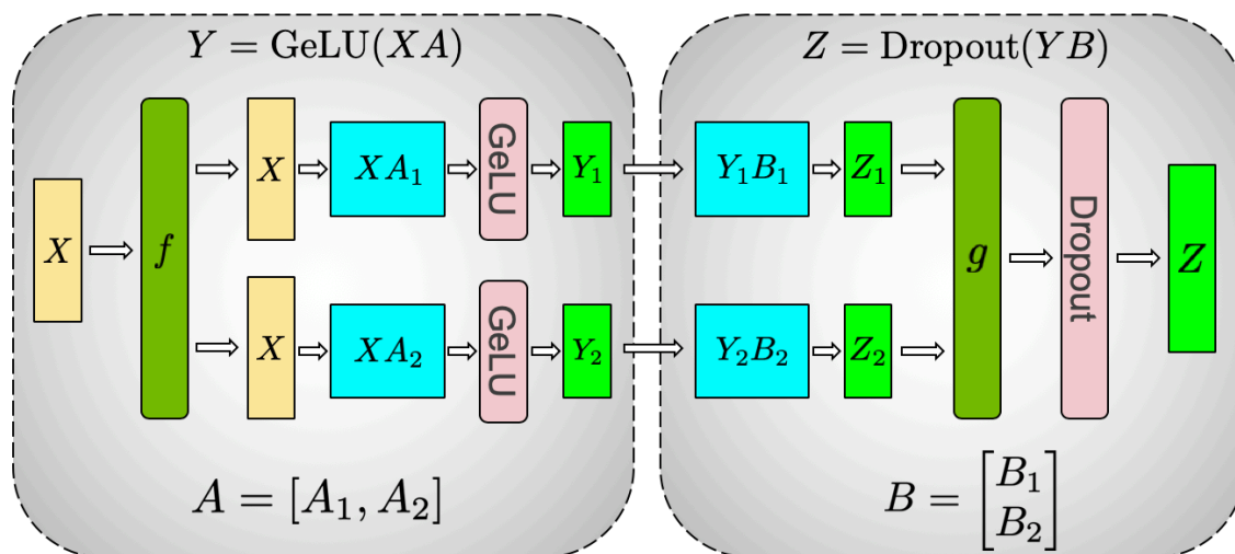
图 28: Megatron 把 MLP 子层做张量并行的切法。第一个权重矩阵 A 按列切成 A_1 、 A_2 ，输入 X 完整复制给两条支路，各算 XA_1 、 XA_2 并各过一个 GeLU（逐元素激活，无需通信）；第二个权重矩阵 B 按行切成 B_1 、 B_2 ，两条支路各算 Y_1B_1 、 Y_2B_2 得到部分和，最后那个 g 把两个部分和规约（求和）成完整输出。整层只在末尾汇总处发生一次跨卡通信
