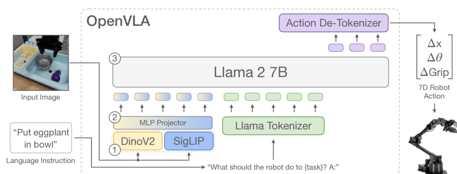
图 36: OpenVLA 的数据通路。左侧输入是一张相机图和一句语言指令“Put eggplant in bowl”；图像经 DinoV2 与 SigLIP 两个编码器并联，再过 MLP 投影成视觉 token，指令经 Llama Tokenizer 成文本 token，两串 token 拼在一起送进 Llama 2 7B；输出端的动作 token 经 Action De-Tokenizer 还原成 [\Delta x, \Delta \theta, \Delta \text{Grip}] 这样一个 7 维机器人动作。（图取自参考文献 [7]）
