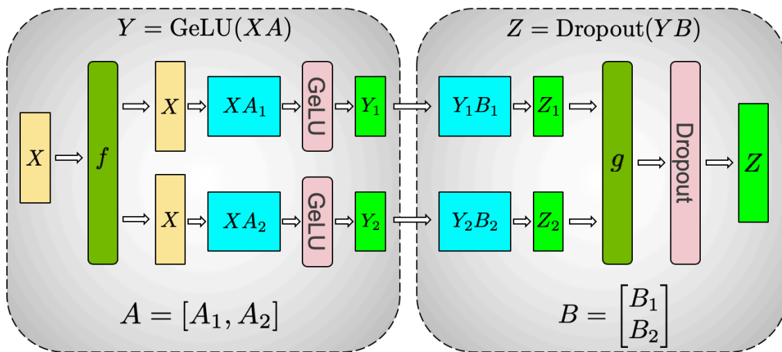
图 26: 图：Megatron 把 MLP 子层做张量并行的切法。第一个权重矩阵 A 按列切成 A_1 、 A_2 ，输入 X 完整复制给两条支路，各算 XA_1 、 XA_2 并各过一个 GeLU（逐元素激活，无需通信）；第二个权重矩阵 B 按行切成 B_1 、 B_2 ，两条支路各算 Y_1B_1 、 Y_2B_2 得到部分和，最后那个 g 把两个部分和规约（求和）成完整输出。整层只在末尾汇总处发生一次跨卡通信
