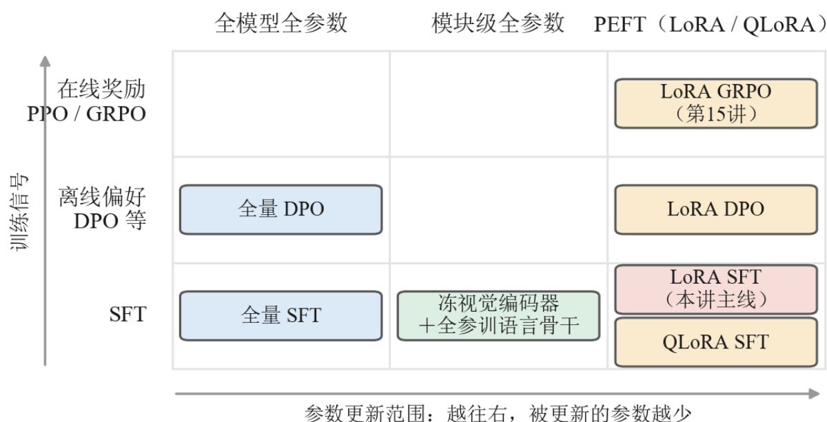
图 3: 一张三行三列的方法地图。列是参数更新范围：全模型全参数 / 模块级全参数 / PEFT (LoRA、QLoRA)，图下注明越往右被更新的参数越少；行是训练信号：自下而上为 SFT、离线偏好 DPO 等、在线奖励 PPO / GRPO。九个格子里有六格填着本讲提到的组合：左列是全量 SFT 与全量 DPO，中列只有“冻视觉编码器 + 全参训语言骨干”一格，右列自下而上是 LoRA SFT 与 QLoRA SFT (上下叠在同一格)、LoRA DPO、标着第 15 讲的 LoRA GRPO；红框那格 LoRA SFT 标着“本讲主线”。三个空格不是不能组合，只是本讲没走那条路
