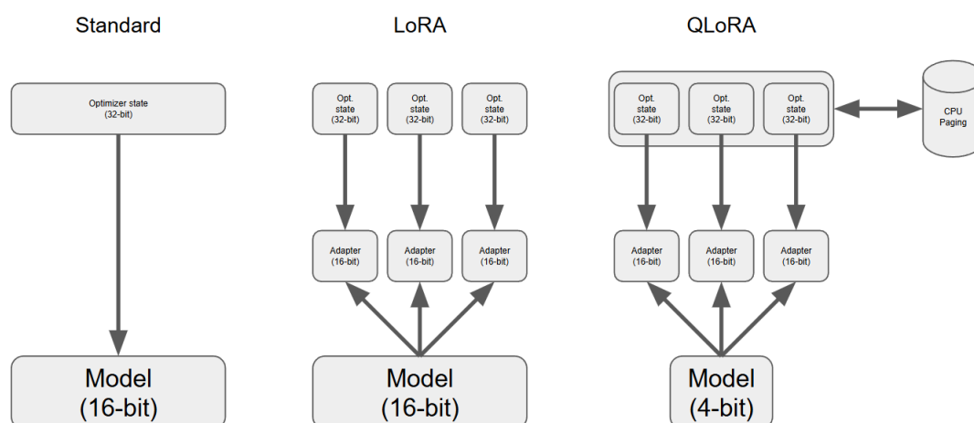
图 15: 图：标准微调、LoRA、QLoRA 三种方式的显存构成对照——基座权重、适配器与优化器状态各占多少、各处是什么精度
