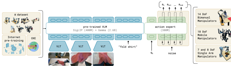
图 35: 图: \pi_0 的框架。左端是训练数据来源—— \pi 自采数据集、互联网预训练语料与 OXE (Open X-Embodiment); 中间是预训练 VLM, 标注为 SigLIP (400M) + Gemma (2.6B), 多路相机图各过一个 ViT, 与指令 “fold shirt” 一起进入; 右接一个 300M 的动作专家, 输入当前关节状态 q_t 和噪声, 输出动作块 a_t, a_{t+1}, \dots, a_{t+H} ; 最右列出三类目标本体——14 自由度双臂、18 自由度移动操作、7 与 8 自由度单臂。(图取自参考文献 [8])
