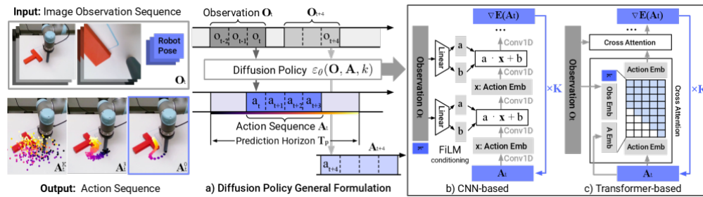
图 33: 图: 论文的方法总览, 分三格。左格是输入输出示例——上排是机械臂的图像观测序列, 下排三张图叠着彩色散点, 画的是同一个观测下采出的多条候选动作序列。中格是通用形式: 观测 O_t 送进去噪声网络 \epsilon_\theta(O, A, k) , 一次吐出预测时域 T_p 内的一整段动作 A_t , 只执行开头几步再重新预测。右两格是两种网络实现: CNN 版用 FiLM 把观测条件注入一维卷积, Transformer 版用交叉注意力。(图取自参考文献 [36])
