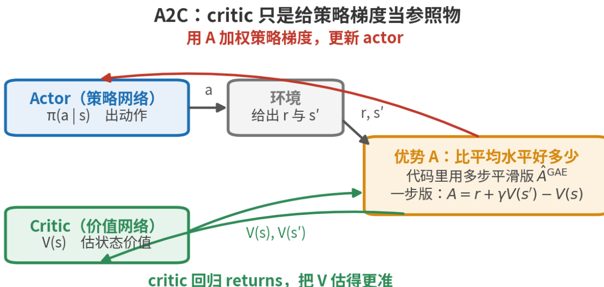
图 11: A2C 的 Actor-Critic 分工：actor（策略网络）出动作，critic（价值网络）估状态价值、帮 actor 算优势。优化主体仍是策略，critic 只当参照物
