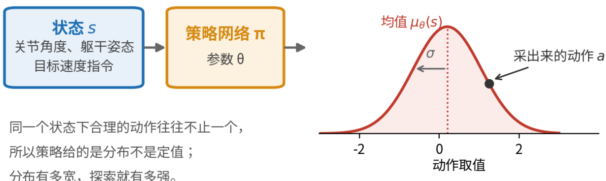
图 4: 策略把状态映射成的是一个 动作分布 ，不是一个定值：左边是输入（关节角度、躯干姿态、目标速度指令），中间是参数为 \theta 的网络，右边是它吐出来的高斯密度——峰值处的均值 \mu_{\theta}(s) 是“最想做的动作”，从均值往外量出去的那一段 \sigma 就是探索强度，黑点是这一步真正采出来去执行的那个 a 。 \sigma 越宽，采到离均值远的动作的机会越大
