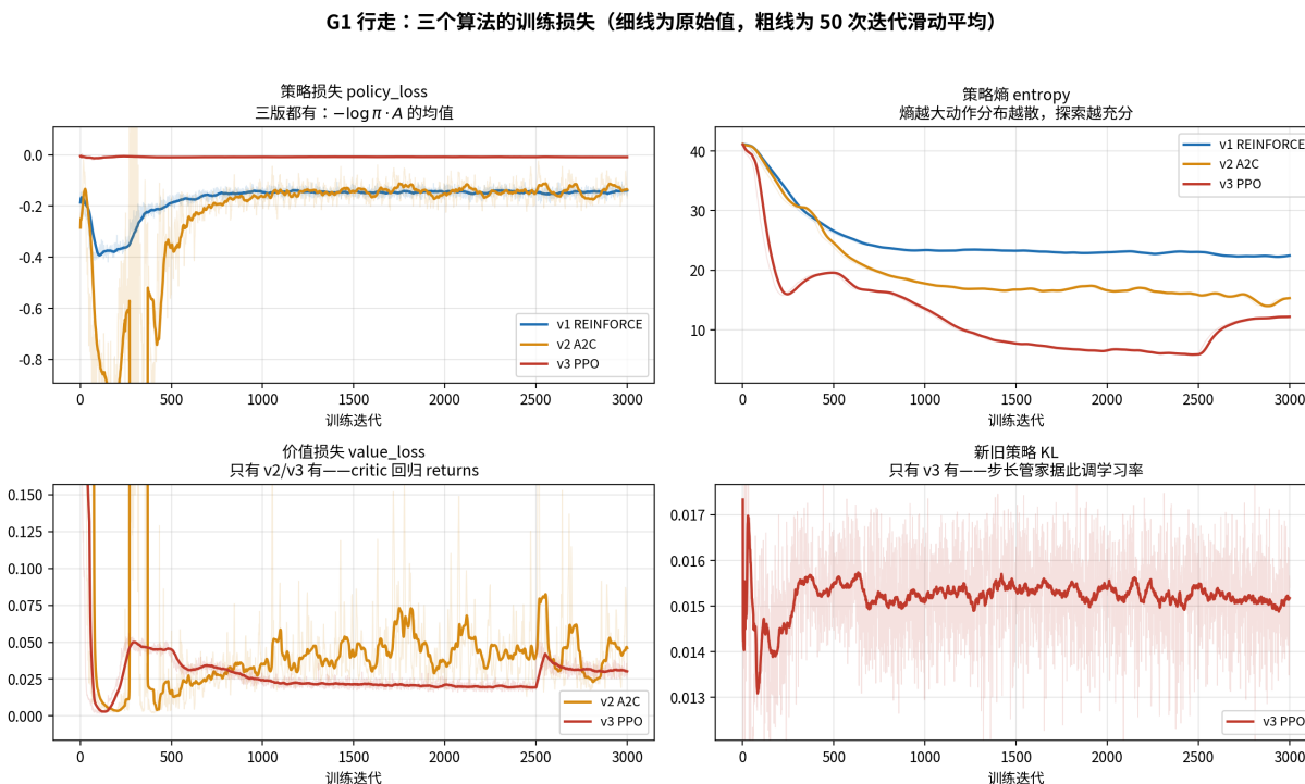
图 16: G1 行走三算法的训练损失（细线为每次迭代原始值，粗线为 50 次迭代滑动平均）：左上策略损失三版都有；右上策略熵反映探索强度；左下价值损失只有 v2/v3 有；右下新旧策略 KL 只有 v3 记录。数据来源：code/rl/1_rl_basics/result/1_1_g1_walk_rl/train-loss-curves.json
