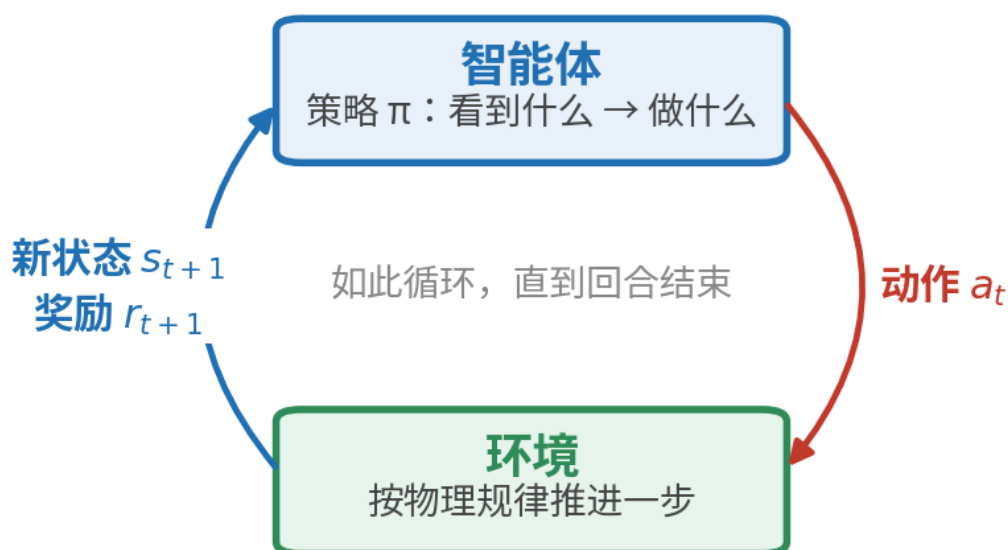
图 1: 智能体与环境的交互闭环: 智能体在状态 s_t 下输出动作 a_t , 环境返回新的状态 s_{t+1} 和奖励 r_{t+1} (“做完 a_t 之后拿到的那一份”), 如此循环
