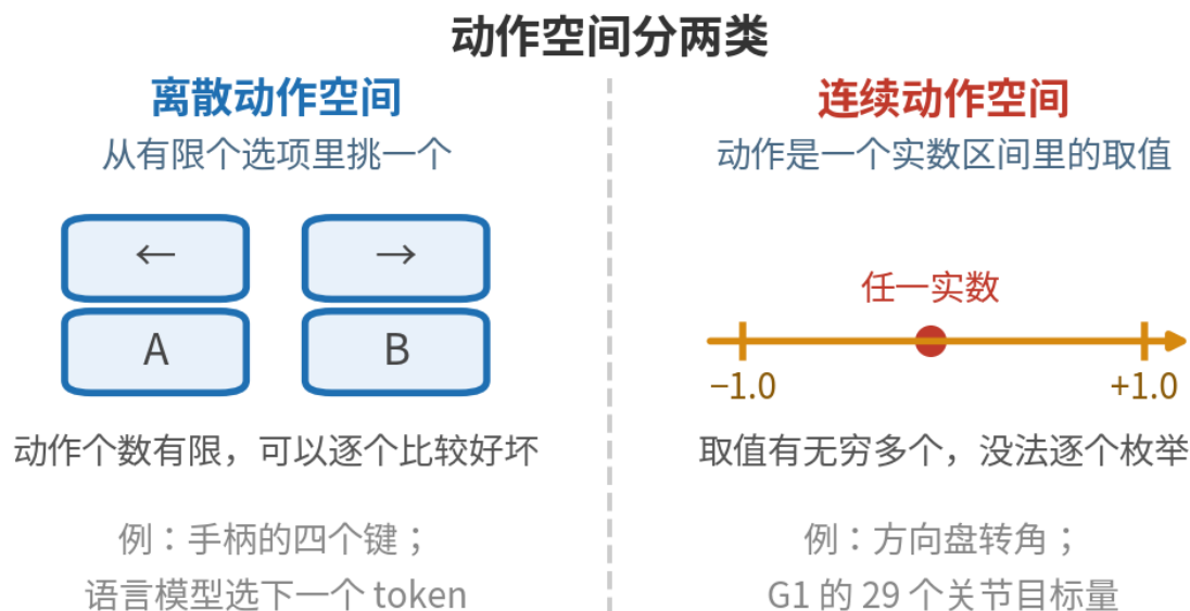
图 2: 动作空间分两类。左边是离散：动作是几个方框里挑一个（图上画的是手柄的四个键），数得清，所以可以逐个比较好坏。右边是连续：动作是一根实数轴上的任意一点（图上画的是 -1 到 +1 这段），取值有无穷多个，没法逐个枚举
