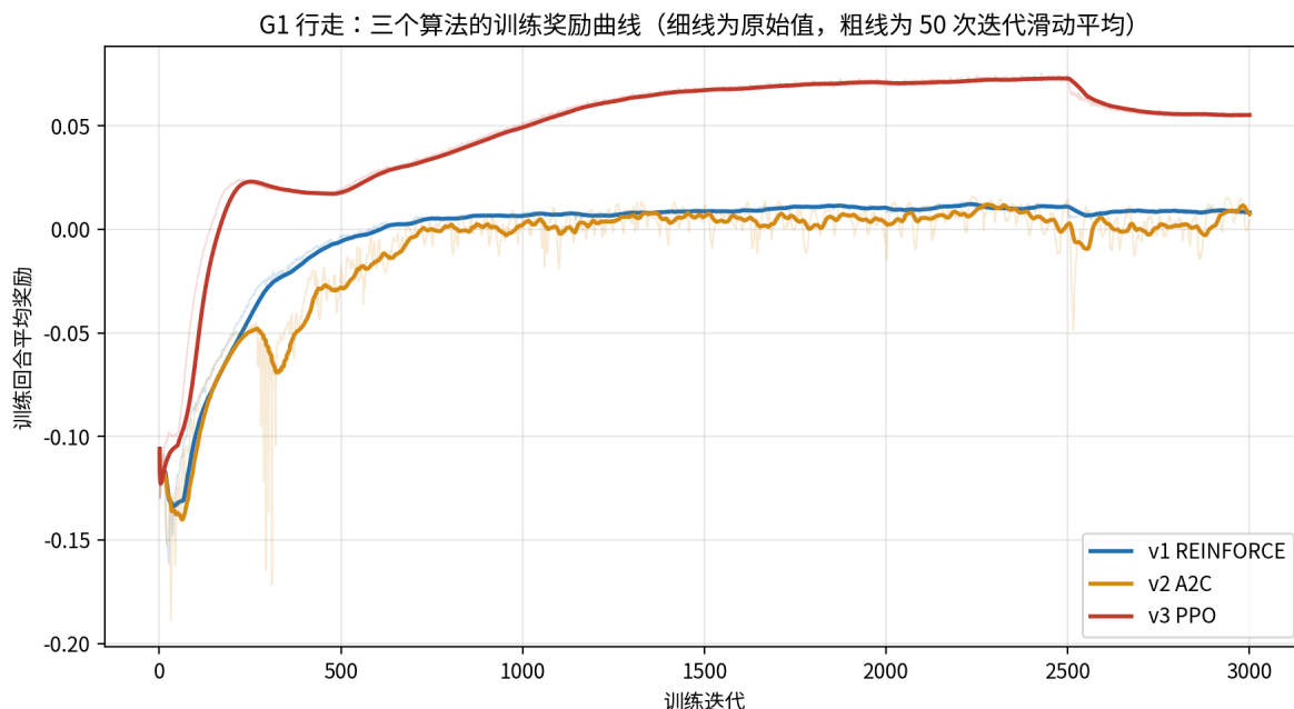
图 15: G1 行走三算法的训练奖励曲线（同为 3000 次迭代，细线为每次迭代的原始值，粗线为 50 次迭代的滑动平均）：v3 PPO 爬到 0.073 附近，在约 2500 迭代处掉了一级、余下区间稳在 0.055；v1 与 v2 大约 700 迭代后就压在 0 附近再没上去，v2 的原始曲线抖动幅度最大。数据来源：code/r1/1_rl_basics/result/1_1_g1_walk_rl/train-reward-curves.json
