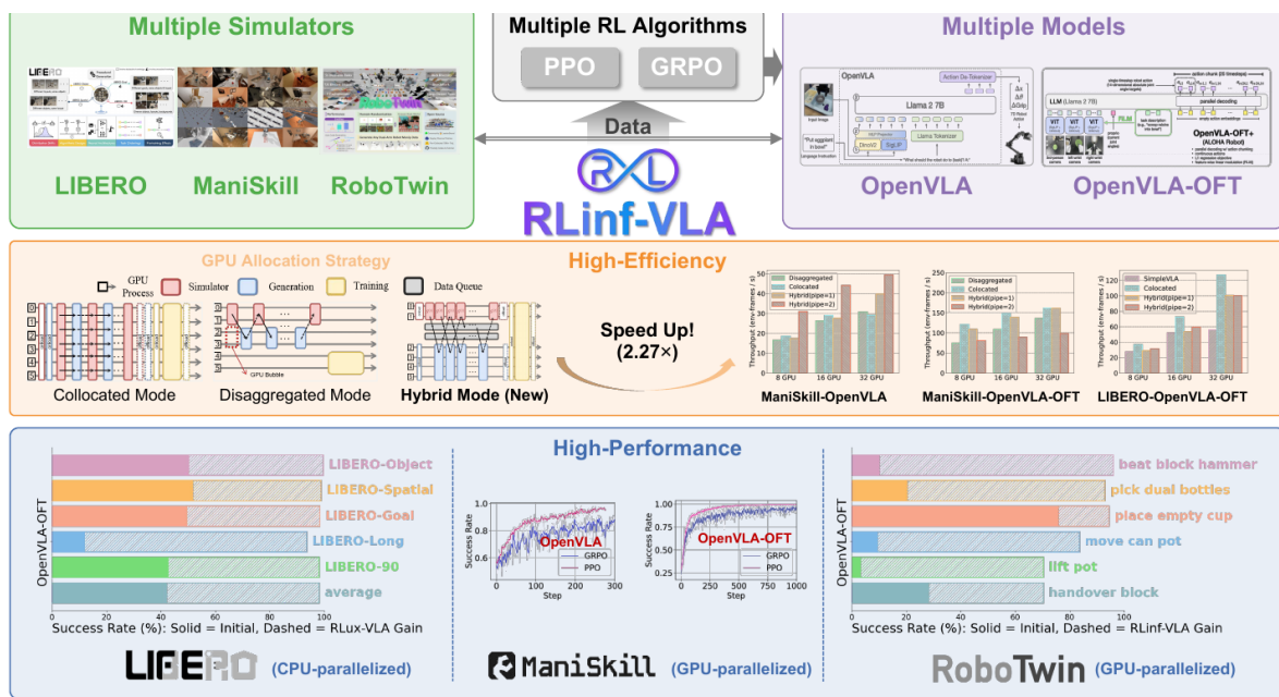
图 11: RLinf-VLA 总览，自上而下三层：统一接口层把仿真器、VLA 模型、RL 算法三个维度都做成可插拔的；中间一层并排比较三种 GPU 分配编排；最下一层是三个基准上的成功率面板
