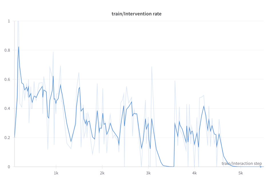
图 19: 一次健康训练的干预率曲线：从 0.5 上下的高位总体下行，3.3k 步附近一度归零；随后有一段回升到 0.3 左右并持续约一千步，4.7k 步后才稳定归零（截图自 LeRobot 官方文档）
