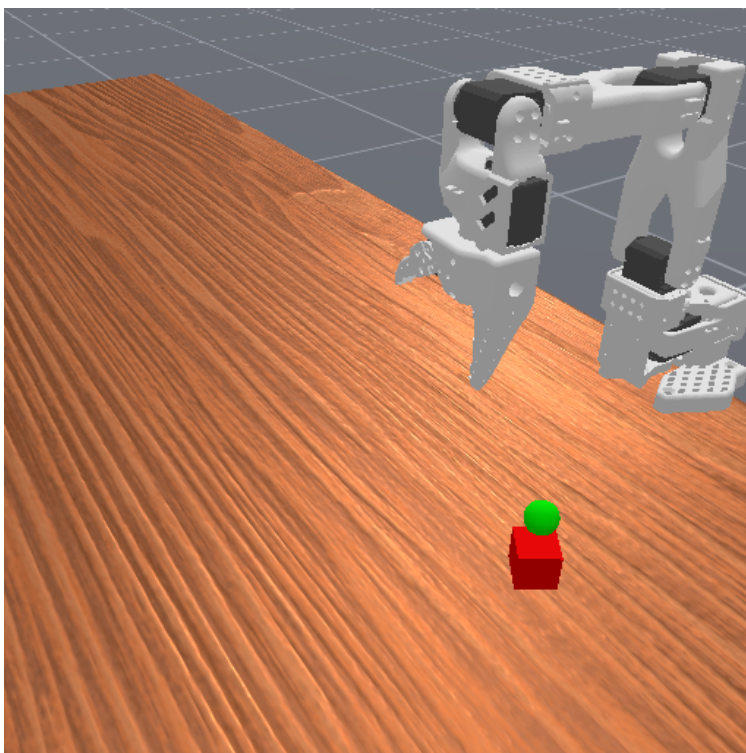
图 4: SO-101 机械臂与 ReachCube 任务：低成本的 SO-101 臂要把末端够到桌面上的方块，红块顶端的绿色小球是目标标记
