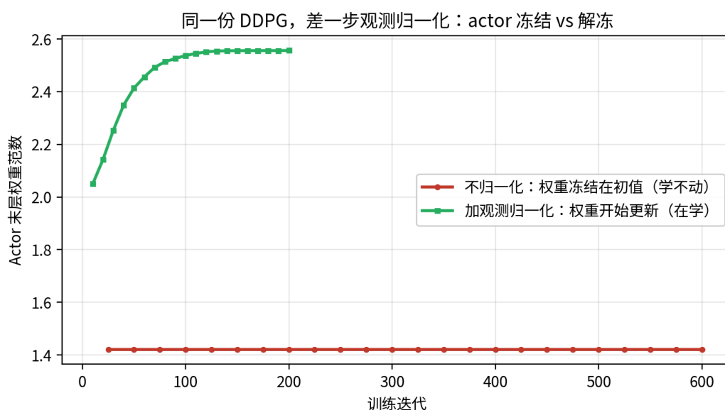
图 6: 同一份 DDPG，只差一步观测归一化。纵轴是 Actor 末层的权重范数 ，不是奖励：不归一化那次（红）600 次迭代死死钉在 1.42，一位小数都没动过；加上在线观测归一化那次（绿）从 2.05 一路涨到 2.55 才收住——网络在改自己的参数，梯度是通的（数据来源：3.1 节说明的那次单相机 ReachCube 实验的训练记录）
