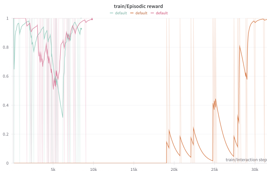
图 18: 人工干预对学习速度的影响：三条 episodic reward 曲线里，无干预那次（橙）到约 3 万交互步才追上最高回报，有人干预的两次（粉、绿）在 1 万步以内就到顶。图例三条都写作 default ，哪条是哪次取自 LeRobot 官方文档的说明
