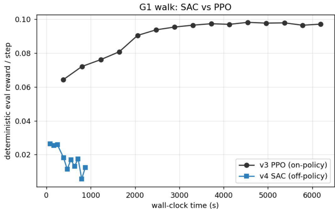
图 13: 按墙钟时间对齐的同两条曲线：3000 次迭代 SAC 约 875 秒、PPO 约 6190 秒；SAC 那条在头四分钟里就走完了全部涨幅，剩下的 11 分钟在往下走
