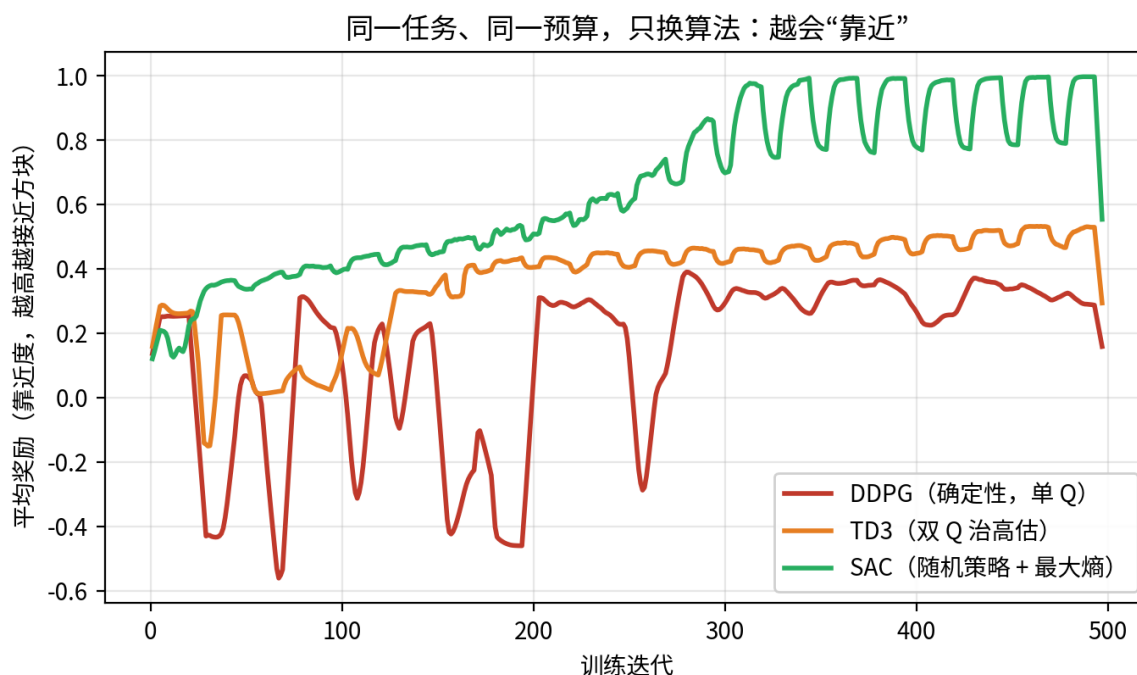
图 7: 同一任务、同一预算（500 次迭代），只换算法。纵轴平均奖励是“靠近度”的代理——越高表示末端越接近方块。DDPG（红）在正负之间大起大落，最后一次探到 -0.29 在两百五十次前后，此后在 0.3 上下（ 0.23 \sim 0.37 ）走完；TD3（橙）头一百三十次也在晃，此后平滑爬升并停在 0.42 \sim 0.53 的平台；SAC（绿）从头到尾稳步上行，三百次之后八成时间在 0.8 \sim 1.0 ，锯齿谷底探到 0.7 （数据来源：3.1 节说明的那次单相机 ReachCube 实验的训练记录）
