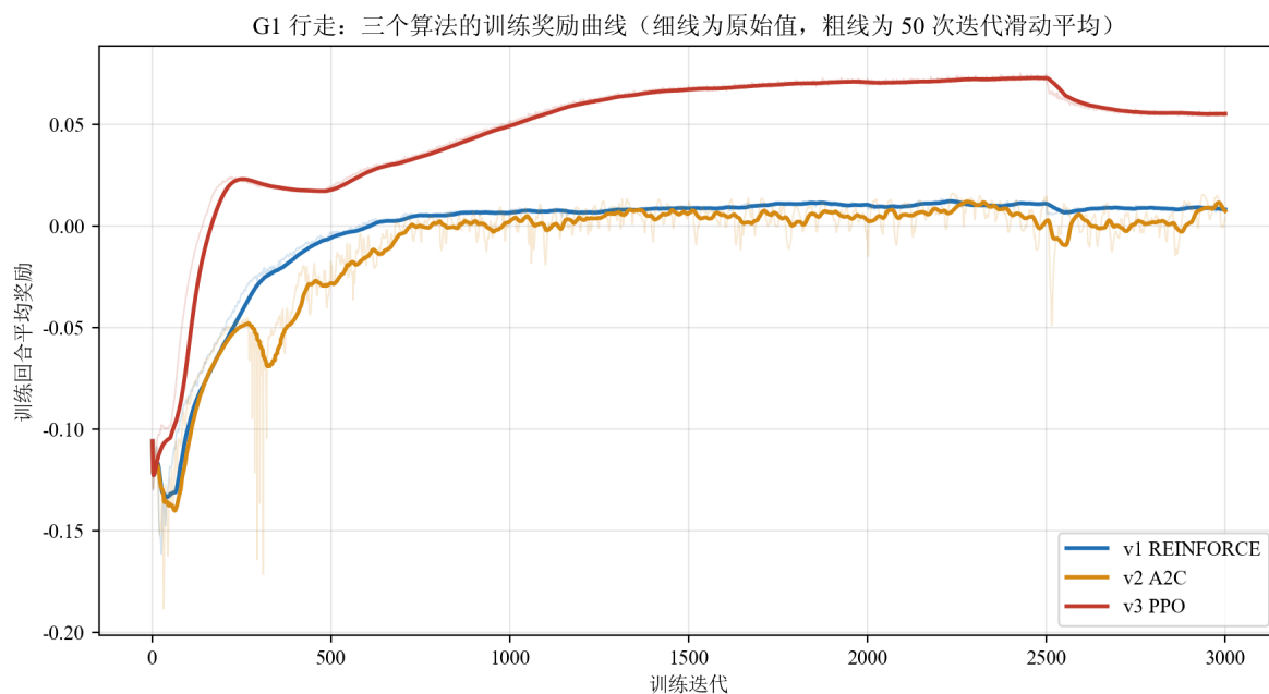
图 16: G1 行走三算法的训练奖励曲线 (同为 3000 次迭代, 细线为每次迭代的原始值, 粗线为 50 次迭代的滑动平均): v3 PPO 爬到 0.073 附近, 在约 2500 迭代处掉了一级、余下区间稳在 0.055; v1 与 v2 大约 700 迭代后就压在 0 附近再没上去, v2 的原始曲线抖动幅度最大。数据来源: code/r1/1_rl_basics/result/1_1_g1_walk_rl/train-reward-curves.json
