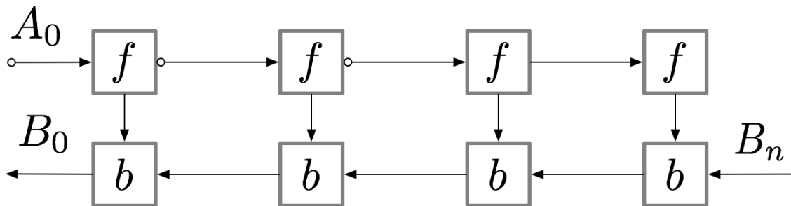
图 25: 梯度检查点下反向传播的执行： f 是前向（重算）、 b 是反向。反向是分段走的：每要算一段的梯度，就先从上游检查点重做一次局部前向 f 补出该段激活，紧接着做这一段的反向 b 。算力上多花了若干次前向重算，换来的是中间激活不必全程驻留显存
