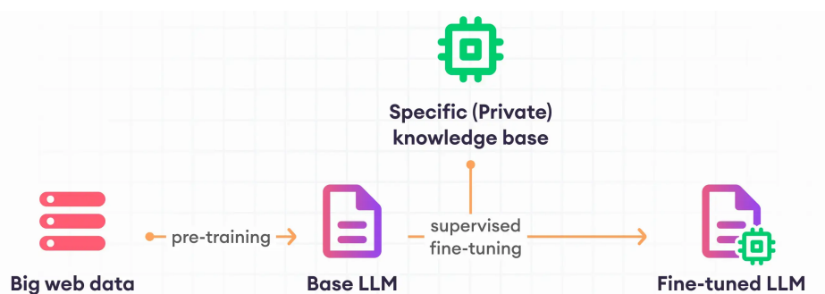
图 1：一条从左到右的链：大规模 Web 数据经预训练得到 Base LLM，再经监督微调得到 fine-tuned LLM；微调那一步上方另有一支箭头，把特定的（私有）知识库喂进来
