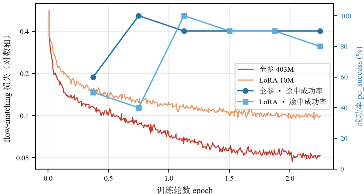
图 18: 两条 flow-matching 损失曲线（对数轴）与两组途中成功率：红色是全参 403M、橙色是 LoRA 10M，LoRA 的损失全程高一截、末点 0.099 对 0.052；深浅两色的方点与圆点是每 5000 步一次的途中成功率，两者最后都落在 80~90% 一带
