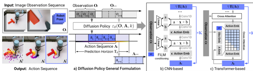
图 36: 论文的方法总览，分三格。左格是输入输出示例——上排是机械臂的图像观测序列，下排三张图叠着彩色散点，画的是同一个观测下采出的多条候选动作序列。中格是通用形式：观测 O_t 送进去噪声网络 \varepsilon_\theta(O, A, k) ，一次吐出预测时域 T_p 内的一整段动作 A_t ，只执行开头几步再重新预测。右两格是两种网络实现：CNN 版用 FiLM 把观测条件注入一维卷积，Transformer 版用交叉注意力。（图取自参考文献 [36]）
