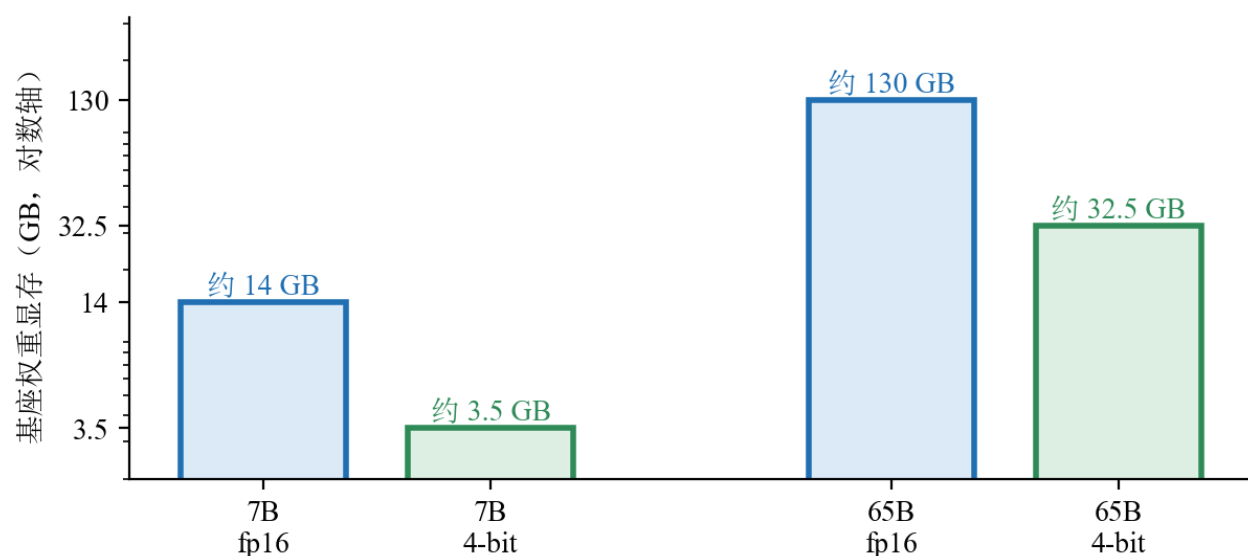
图 16: 基座模型权重显存的粗略对比, 四根柱子分两组, 纵轴取对数: 7B 在 fp16 下约 14 GB、压到 4-bit 后约 3.5 GB; 65B 在 fp16 下约 130 GB、压到 4-bit 后约 32.5 GB (四个数按 fp16 每参数 2 字节、4-bit 每参数 0.5 字节直接折算)
