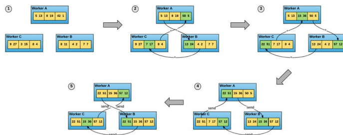
图 21: ring-allreduce 把各卡排成一个环，每张卡只与相邻两张卡通信：先把自己的梯度切成与卡数相同的若干块，在环上一轮轮地“收下左邻传来的块、累加上自己对应的块、再发给右邻”，转一圈后每个块都集齐了所有卡的贡献；随后再沿环传一圈把已经规约好的块分发到每张卡。整个过程没有中心节点，通信均摊在每条相邻链路上
