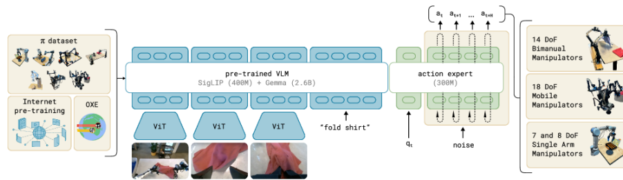
图 38: \pi_0 的框架。左端是训练数据来源—— \pi 自采数据集、互联网预训练语料与 OXE (Open X-Embodiment)；中间是预训练 VLM，标注为 SigLIP (400M) + Gemma (2.6B)，多路相机图各过一个 ViT，与指令“fold shirt”一起进入；右接一个 300M 的动作专家，输入当前关节状态 q_t 和噪声，输出动作块 a_t, a_{t+1}, \dots, a_{t+H} ；最右列出三类目标本体——14 自由度双臂、18 自由度移动操作、7 与 8 自由度单臂。(图取自参考文献 [8])
