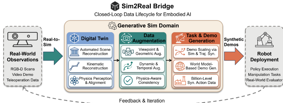
图 40: 中间橙色框是生成式仿真域，内含三列——数字孪生列（自动场景重建 / 运动学重建 / 物理感知与对齐）、数据增强列（视角与几何增强 / 动态与时序增强 / 物理一致性）、任务与示教生成列；左端真实观测（RGB-D 扫描、视频示教、遥操数据）经一支粗箭头进入，右端合成示教喂给真实机器人部署，底部一条虚线箭头从部署折返回真实观测。（图出自参考文献 [39] 图 9）
