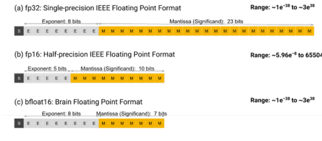
图 23: fp32 / fp16 / bf16 三种浮点格式的位宽与数值范围对比。fp32 用 8 位指数 + 23 位尾数，范围极宽、精度高；fp16 把指数压到 5 位，能表示的最小正数只到约 6 \times 10^{-8} ，范围窄得多；bfloat16 保留 8 位指数（范围和 fp32 一样宽）、只砍尾数到 7 位，用精度换范围
