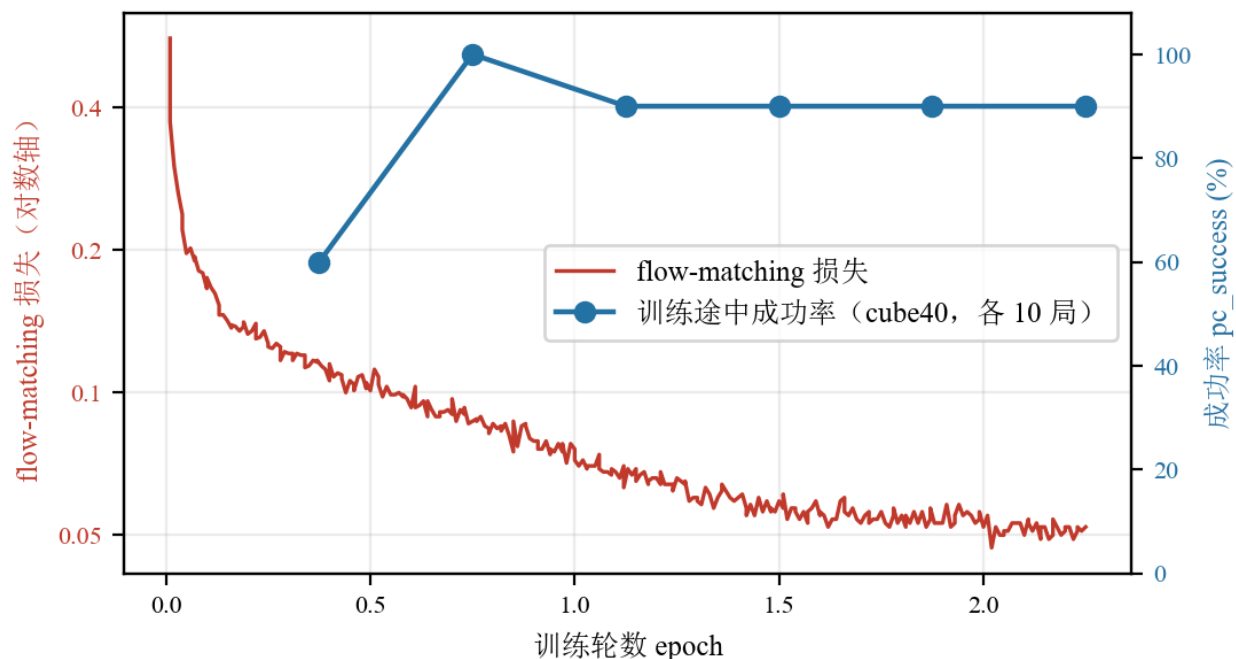
图 11: 左轴红线是 flow-matching 损失 (对数轴), 从 0.56 降到 0.05; 右轴蓝线是训练途中每 5000 步一次的成功率, 六个点依次为 60%、100%、90%、90%、90%、90%
