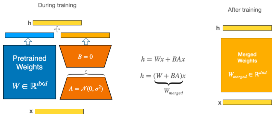
图 13: 左半标注“训练中”: 输入 x 兵分两路, 一路过冻结的 W \in \mathbb{R}^{d \times d} , 一路经下投影 A (图上标 \mathcal{N}(0, \sigma^2) ) 压到 r 维、再由上投影 B (图上标 B = 0 ) 抬回原维度, 两路输出相加; 右半标注“训练后”: W 与 BA 已合并成单块 W_{merged} , 旁路不再出现
