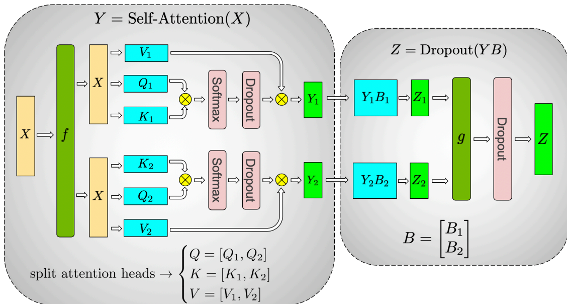
图 30: 注意力子层的张量并行: 多头注意力按头切到两张卡, 卡 1 负责一组头的 Q_1, K_1, V_1 、卡 2 负责另一组 Q_2, K_2, V_2 , 各自独立完成 Softmax 与加权 (图中两条并行支路互不通信), 输出投影矩阵 B 按行切, 末尾 g 把两路部分和规约成完整输出。和 MLP 一样, 整层前向只在出口通信一次
