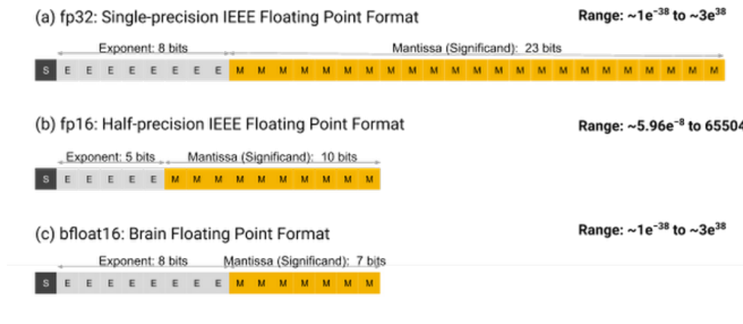
图 19: fp32 / fp16 / bf16 三种浮点格式的位宽与数值范围对比。fp32 用 8 位指数 + 23 位尾数，范围极宽、精度高；fp16 把指数压到 5 位，能表示的最小正数只到约 6 \times 10^{-8} ，范围窄得多；bf16 保留 8 位指数（范围和 fp32 一样宽）、只砍尾数到 7 位，用精度换范围
