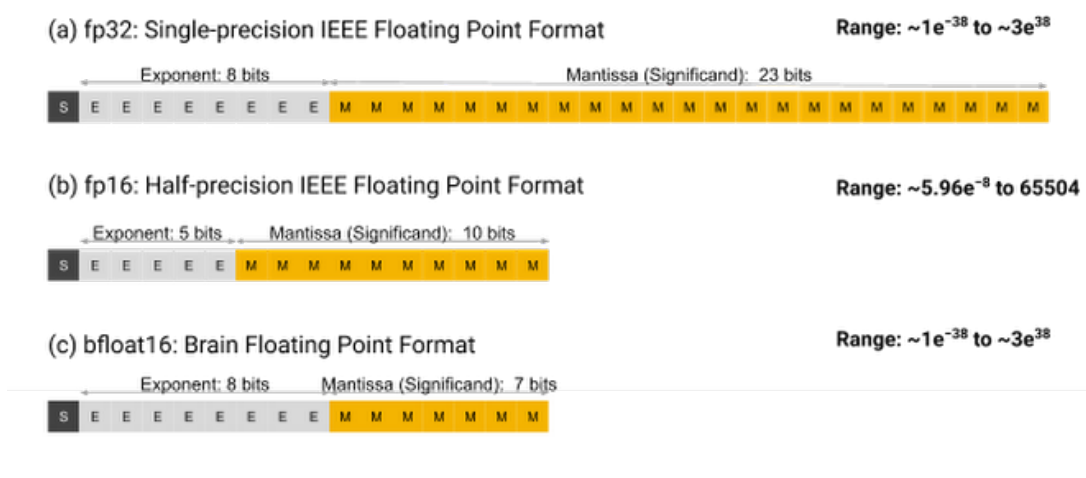
图 21: fp32 / fp16 / bf16 三种浮点格式的位宽与数值范围对比。fp32 用 8 位指数 + 23 位尾数，范围极宽、精度高；fp16 把指数压到 5 位，能表示的最小正数只到约 6 \times 10^{-8} ，范围窄得多；bf16 保留 8 位指数（范围和 fp32 一样宽）、只砍尾数到 7 位，用精度换范围
