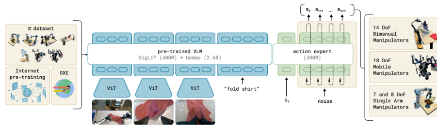
图 36: \pi_0 的框架。左端是训练数据来源—— \pi 自采数据集、互联网预训练语料与 OXE (Open X-Embodiment); 中间是预训练 VLM, 标注为 SigLIP (400M) + Gemma (2.6B), 多路相机图各过一个 ViT, 与指令 “fold shirt” 一起进入; 右接一个 300M 的动作专家, 输入当前关节状态 q_t 和噪声, 输出动作块 a_t, a_{t+1}, \dots, a_{t+H} ; 最右列出三类目标本体——14 自由度双臂、18 自由度移动操作、7 与 8 自由度单臂。(图取自参考文献 [8])
