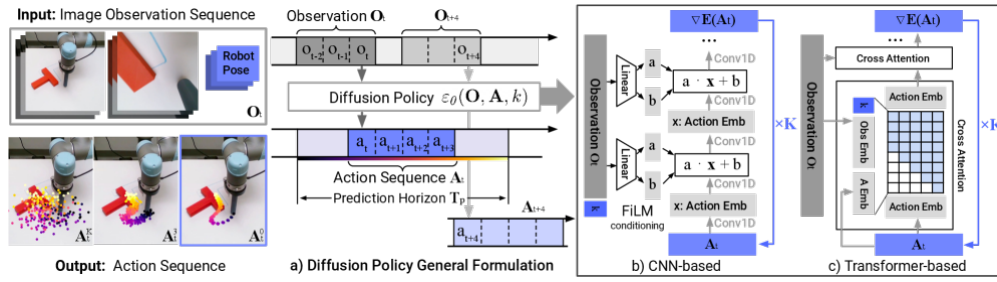
图 34: 论文的方法总览, 分三格。左格是输入输出示例——上排是机械臂的图像观测序列, 下排三张图叠着彩色散点, 画的是同一个观测下采出的多条候选动作序列。中格是通用形式: 观测 \mathbf{O}_t 送进去噪声网络 \varepsilon_\theta(\mathbf{O}, \mathbf{A}, k) , 一次吐出预测时域 T_p 内的一整段动作 \mathbf{A}_t , 只执行开头几步再重新预测。右两格是两种网络实现: CNN 版用 FiLM 把观测条件注入一维卷积, Transformer 版用交叉注意力。(图取自参考文献 [36])
