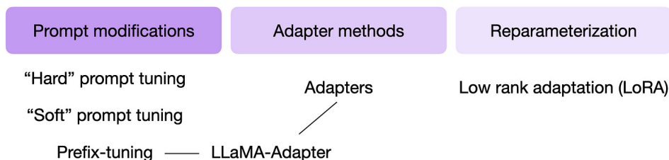
图 6: 三个并排的紫色标题条把常见 PEFT 方法分成三栏。Prompt modifications 栏下列着“Hard” prompt tuning、“Soft” prompt tuning 与 Prefix-tuning; Adapter methods 栏下列着 Adapters 与 LLaMA-Adapter, 并有一条连线把 Prefix-tuning 与 LLaMA-Adapter 连起来; Reparameterization 栏下只有一项 Low rank adaptation (LoRA)
