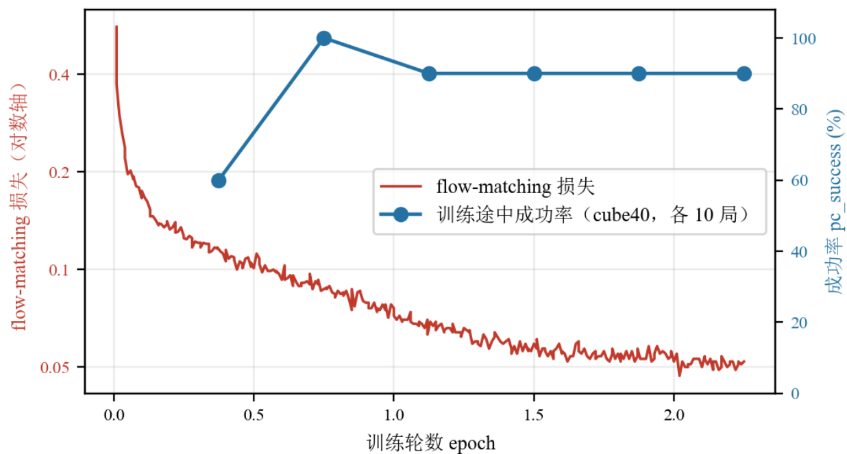
图 11: 左轴红线是 flow-matching 损失（对数轴），从 0.56 降到 0.05；右轴蓝线是训练途中每 5000 步一次的成功率，六个点依次为 60%、100%、90%、90%、90%、90%
