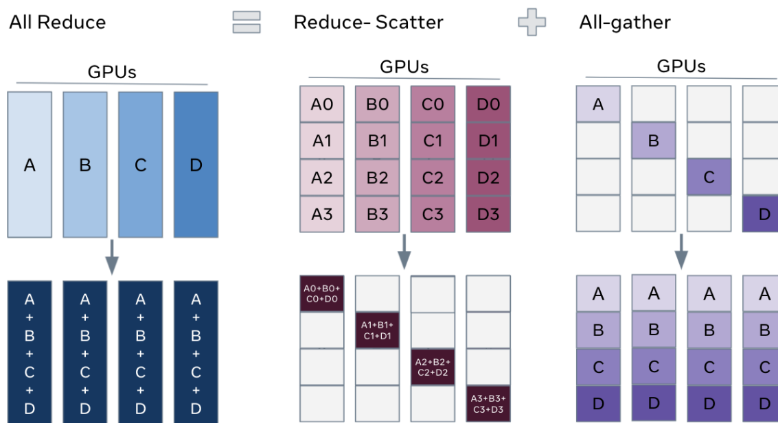
图 24: 同一批要在各卡间对齐的数据，三种集合通信的差别：左边 All-Reduce 把各卡的整份数据规约（求和）后让人手一份相同结果，是 DDP 同步梯度用的；中间 Reduce-Scatter 先按分片求和、但每张卡只收下自己负责的那一片求和结果（每卡只留 1/N 的规约梯度）；右边 All-Gather 把各卡手里的分片拼接起来，让每张卡集齐完整的一份。ZeRO/FSDP 正是用 all-gather 临时拼回完整参数、用 reduce-scatter 把梯度规约后直接切片落到各卡
