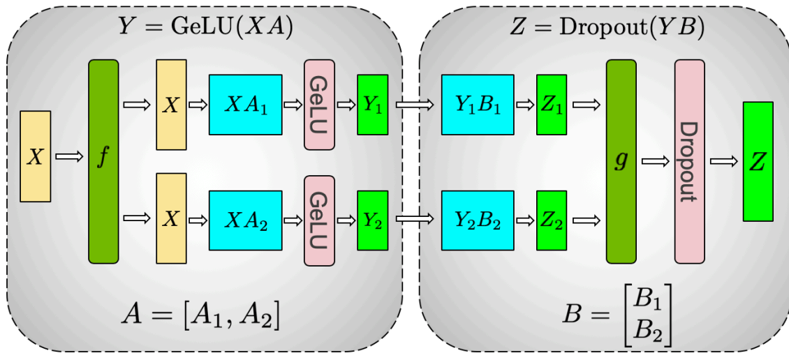
图 27: Megatron 把 MLP 子层做张量并行的切法。第一个权重矩阵 A 按列切成 A_1 、 A_2 ，输入 X 完整复制给两条支路，各算 XA_1 、 XA_2 并各过一个 GeLU（逐元素激活，无需通信）；第二个权重矩阵 B 按行切成 B_1 、 B_2 ，两条支路各算 Y_1B_1 、 Y_2B_2 得到部分和，最后那个 g 把两个部分和规约（求和）成完整输出。整层只在末尾汇总处发生一次跨卡通信
