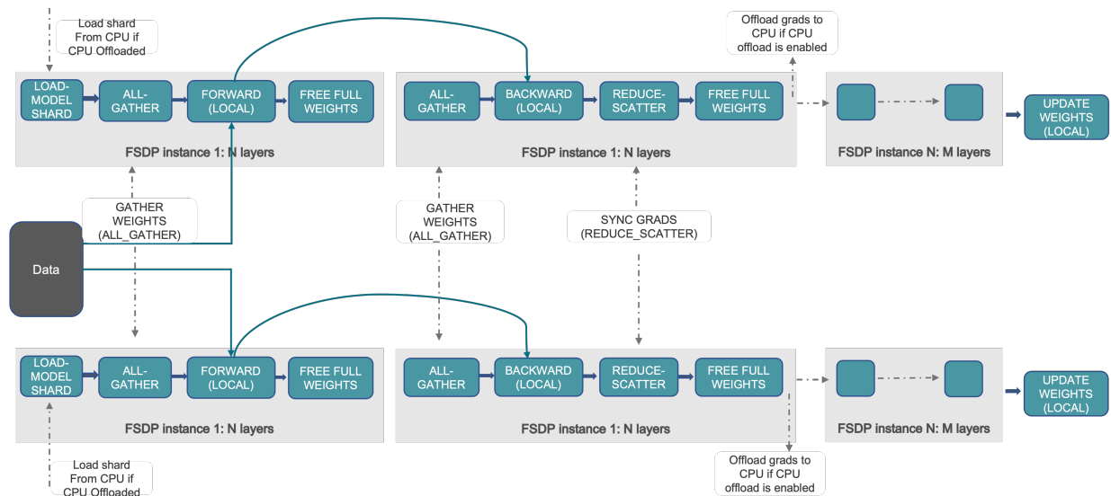
图 26: FSDP 的一步训练工作流。模型被切成若干 FSDP 单元（图中 FSDP Instance，通常按层/block 分组），每张卡只加载自己那份分片（load model shard）。前向时对当前单元 all-gather 出完整权重（gather weights）、算完该单元前向后释放掉非本地的那部分（free full weights）；反向同理先 all-gather 再算梯度，算完梯度用 reduce-scatter（sync grads）把规约后的梯度切片落到各卡；最后各卡只更新自己那一片参数（update weights）。若开启 offload，分片还能进一步搬到 CPU
