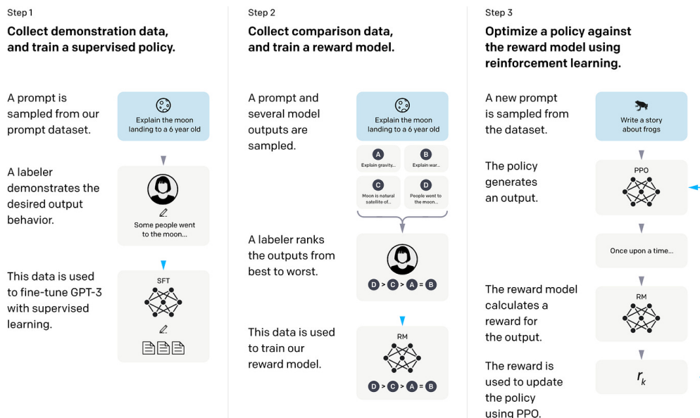
图 9: InstructGPT 的三步流程, 图上分三栏。第一栏: 从提示集抽一条提示 (“Explain the moon landing to a 6 year old”), 标注员写出期望回答, 用它监督微调出 SFT 模型。第二栏: 同一条提示采样出 A-D 四个模型输出, 标注员排出 D > C > A = B 的顺序, 用这批比较数据训练奖励模型。第三栏: 抽一条新提示 (“Write a story about frogs”), 策略生成输出, 奖励模型给出分数 r_k , 再用 PPO 回过头更新策略。(图取自参考文献 [4])
