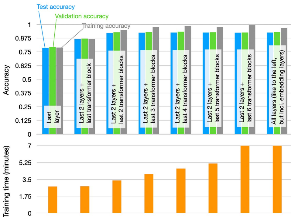
图 4: 不同层解冻方案的对照：上半部分是训练/验证/测试准确率，下半部分是训练时间，横轴从只训练最后一层排到解冻全部层
