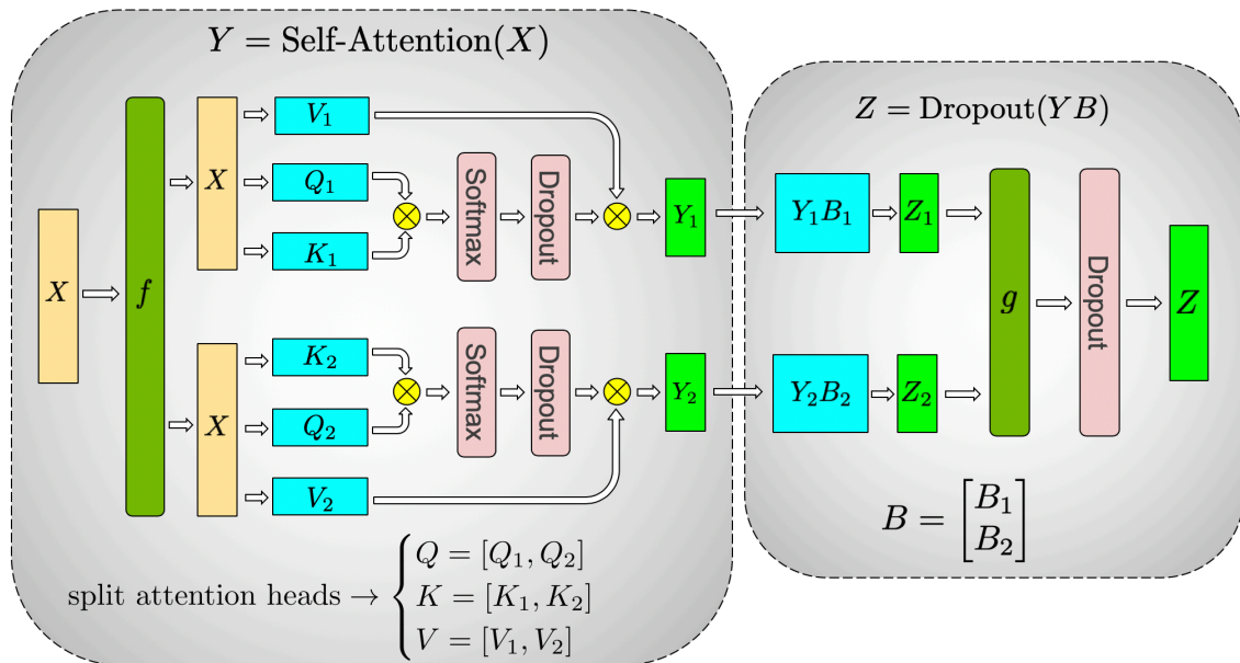
图 28: 注意力子层的张量并行：多头注意力按头切到两张卡，卡 1 负责一组头的 Q_1, K_1, V_1 、卡 2 负责另一组 Q_2, K_2, V_2 ，各自独立完成 \text{Softmax} 与加权（图中两条并行支路互不通信），输出投影矩阵 B 按行切，末尾 g 把两路部分和规约成完整输出。和 MLP 一样，整层前向只在出口通信一次
