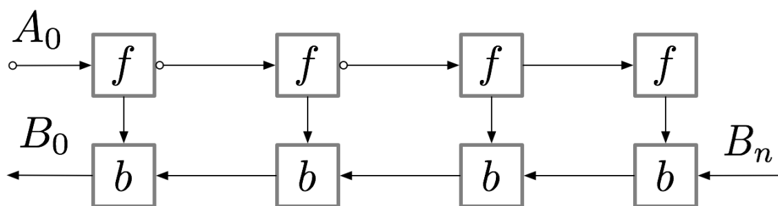
图 23: 梯度检查点下反向传播的执行: f 是前向 (重算)、 b 是反向。反向是分段走的: 每要算一段的梯度, 就先从上游检查点重做一次局部前向 f 补出该段激活, 紧接着做这一段的反向 b 。算力上多花了若干次前向重算, 换来的是中间激活不必全程驻留显存
