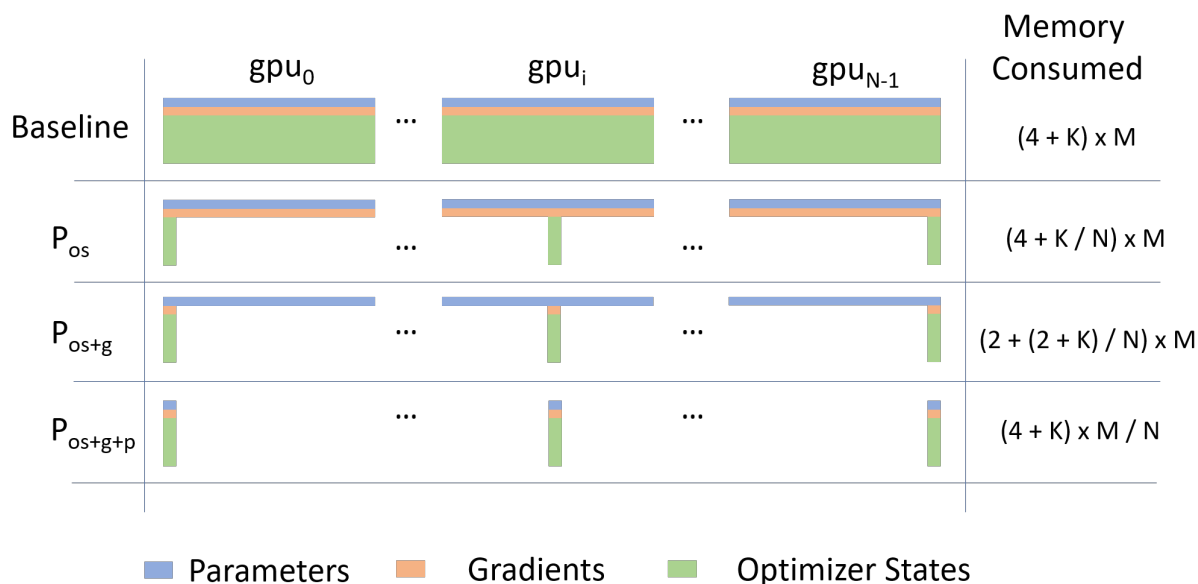
图 25: ZeRO 三阶段分片对比。每一行是一种方案，横向从 \text{gpu}_0 到 \text{gpu}_{N-1} 是各张卡，柱子里蓝 = 参数、橙 = 梯度、绿 = 优化器状态。最上 Baseline（即 DDP）每张卡存满整份 (4 + K)\Psi ； P_{os} （Stage 1）只把绿色优化器状态沿各卡切开，每卡降到 (4 + K/N)\Psi ； P_{os+g} （Stage 2）再切橙色梯度，降到 (2 + (2 + K)/N)\Psi ； P_{os+g+p} （Stage 3）连蓝色参数也切，每卡只剩 (4 + K)\Psi/N 。图中 K 为优化器状态系数（混合精度 Adam K=12 ）， N 为数据并行度（正文写作 N_d ）；图上把参数数量记成 M ，就是正文的 \Psi
