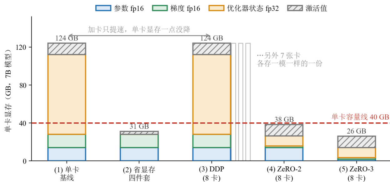
图 31: 一根 7B 模型的单卡显存柱，在五种方案下怎么变。柱子按 4.1.2 节四类吃货分段：参数 fp16（蓝）、梯度 fp16（绿）、优化器状态 fp32（橙）、激活值（斜纹灰）；红色虚线是标着 40 GB 的单卡容量线。(1) 单卡基线 124 GB，高高在线上；(2) 开省显存四件套后橙色的优化器状态整段消失（搬到卡外）、斜纹的激活段被梯度检查点压扁，落到 31 GB；(3) DDP 那根柱子仍标着 124 GB，一条双向箭头从 (1) 拉到 (3)、上面写着“加卡只提速，单卡显存一点没降”，右侧几根灰柱注着“另外 7 张卡各存一模一样的一份”；(4) ZeRO-2 把梯度段和优化器段各切成 1/8，降到 38 GB；(5) ZeRO-3 把三段全部切成 1/8，降到 26 GB。图下一行注明：斜纹那段是激活值，随批量与序列长度变，图上只画一个示意高度，其余三段按 16 字节/参数精确折算（分片按 8 卡算，与 4.4.6 节表里的公式一致）
