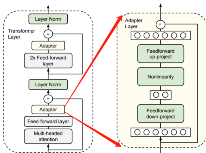
图 7: 左侧是一个 Transformer 层，两个 Adapter 分别插在多头注意力之后和前馈层之后，各自紧接一个 Layer Norm；右侧把其中一个 Adapter 放大：输入先经前馈下投影压到很窄的中间层（图上只画了两个圆点），过非线性，再经前馈上投影回到原宽度，并有一条跳连从入口直接加到出口。（图取自参考文献 [3]）
