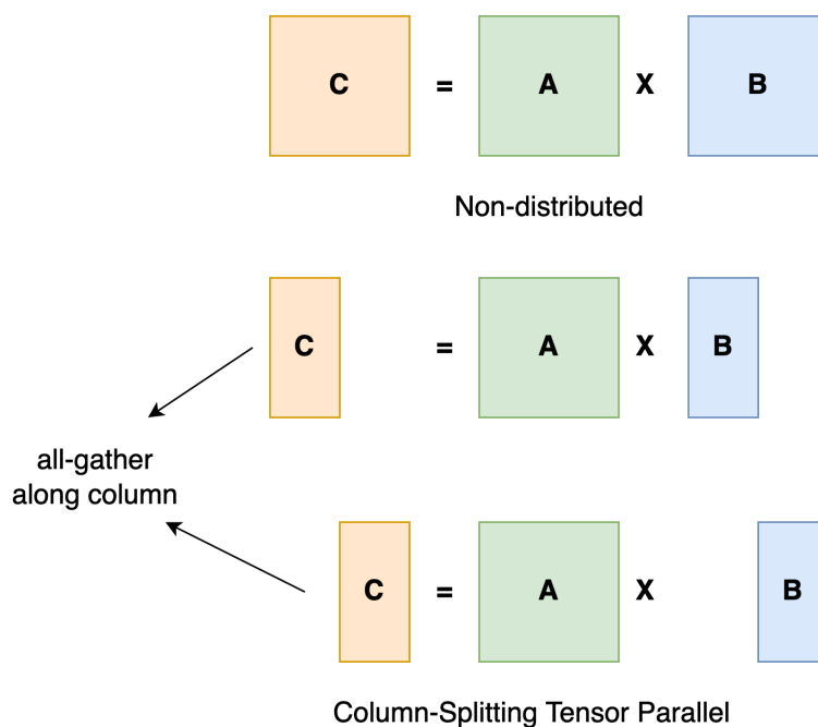
图 18: 模型并行 (张量并行) 示意: 上方是非分布式的整块矩阵乘 C = A \times B ; 下方是按列切分 (Column-Splitting) 后, 每张卡只算结果的一部分列, 再通过 all-gather 沿列方向把各卡的局部结果拼成完整的 C
