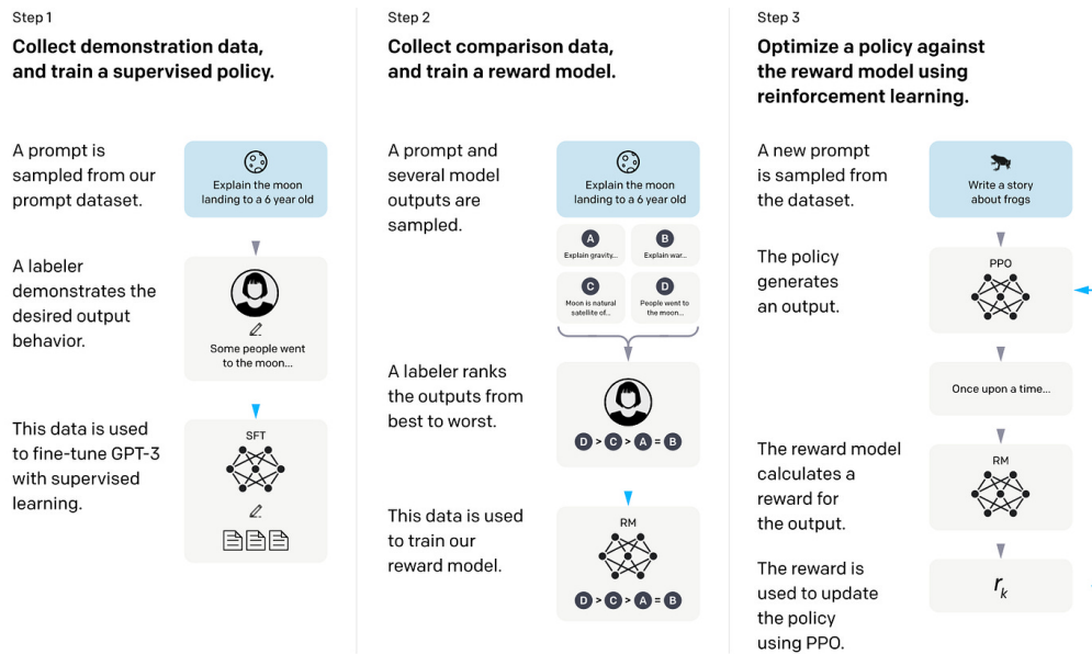
图 10: 图: InstructGPT 的三步流程, 图上分三栏。第一栏: 从提示集抽一条提示 (“Explain the moon landing to a 6 year old”), 标注员写出期望回答, 用它监督微调出 SFT 模型。第二栏: 同一条提示采样出 A-D 四个模型输出, 标注员排出 D > C > A = B 的顺序, 用这批比较数据训练奖励模型。第三栏: 抽一条新提示 (“Write a story about frogs”), 策略生成输出, 奖励模型给出分数 r_k , 再用 PPO 回过头更新策略。(图取自参考文献 [4])
