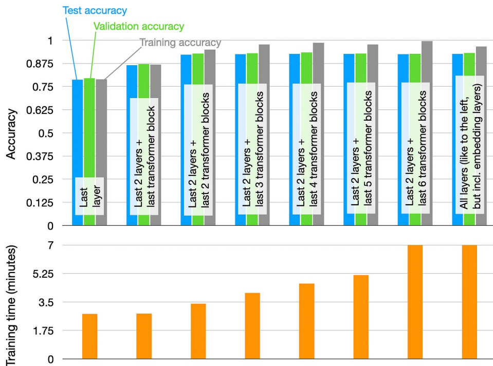
图 5: 图：不同层解冻方案的对照——上半部分是训练/验证/测试准确率，下半部分是训练时间，横轴从只训练最后一层排到解冻全部层
