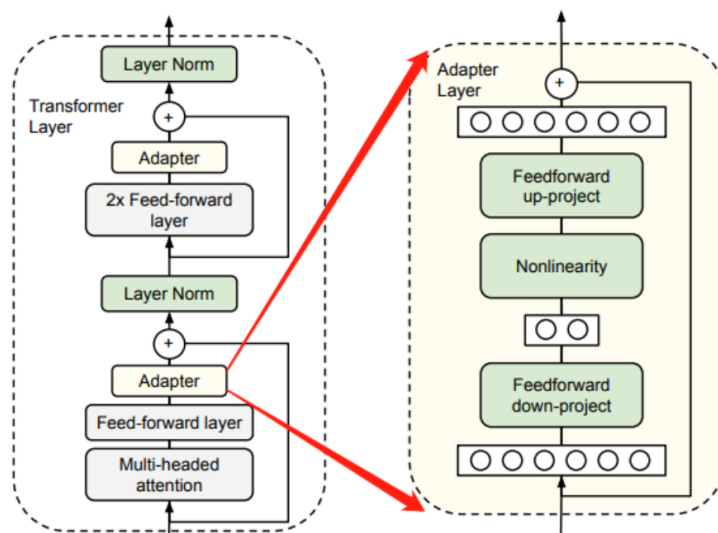
图 8: 图：左侧是一个 Transformer 层，两个 Adapter 分别插在多头注意力之后和前馈层之后，各自紧接一个 Layer Norm；右侧把其中一个 Adapter 放大——输入先经前馈下投影压到很窄的中间层（图上只画了两个圆点），过非线性，再经前馈上投影回到原宽度，并有一条跳连从入口直接加到出口。（图取自参考文献 [3]）
