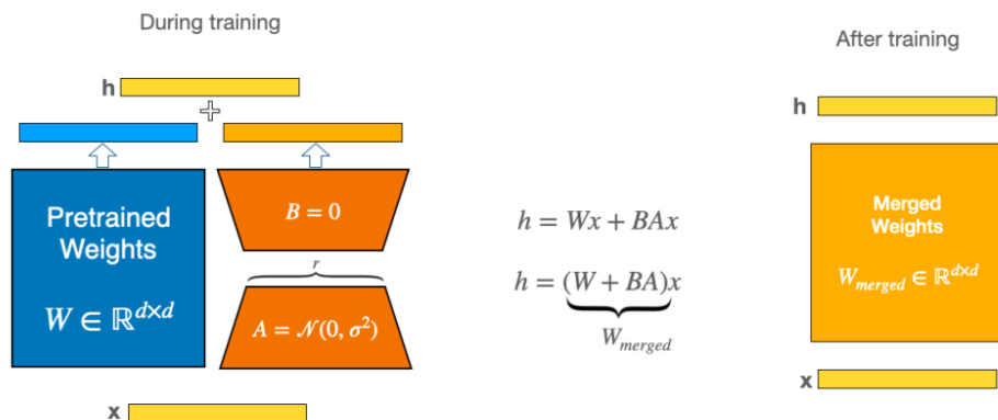
图 11: 图：左半标注”训练中”——输入 x 兵分两路，一路过冻结的 W \in \mathbb{R}^{d \times d} ，一路经下投影 A （图上标 \mathcal{N}(0, \sigma^2) ）压到 r 维、再由上投影 B （图上标 B = 0 ）抬回原维度，两路输出相加；右半标注”训练后”—— W 与 BA 已合并成单块 W_{merged} ，旁路不再出现
