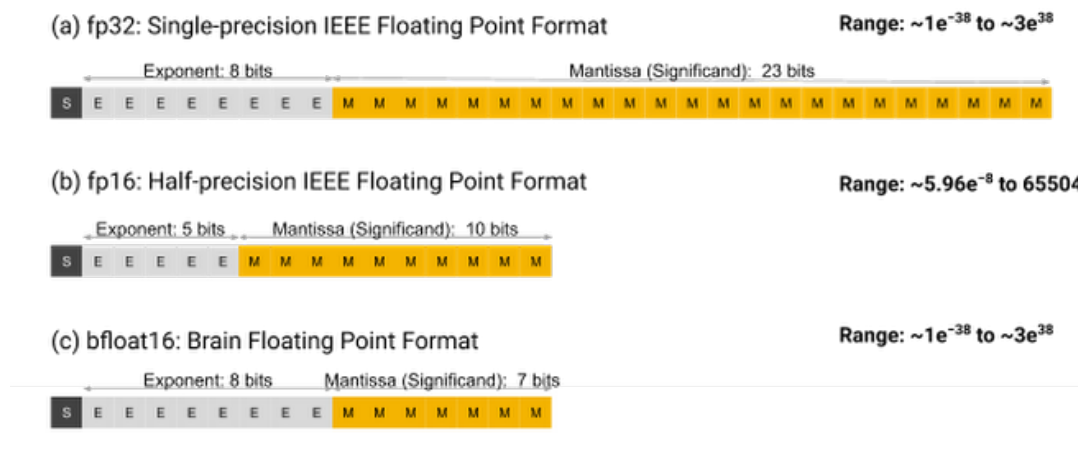
图 20: 图: fp32 / fp16 / bf16 三种浮点格式的位宽与数值范围对比。fp32 用 8 位指数 + 23 位尾数，范围极宽、精度高；fp16 把指数压到 5 位，能表示的最小正数只到约 6 \times 10^{-8} ，范围窄得多；bf16 保留 8 位指数（范围和 fp32 一样宽）、只砍尾数到 7 位，用精度换范围
