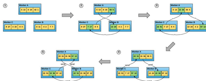
图 18: 图：ring-allreduce 把各卡排成一个环，每张卡只与相邻两张卡通信：先把自己的梯度切成与卡数相同的若干块，在环上一轮轮地”收下左邻传来的块、累加上自己对应的块、再发给右邻”，转一圈后每个块都集齐了所有卡的贡献；随后再沿环传一圈把已经规约好的块分发到每张卡。整个过程没有中心节点，通信均摊在每条相邻链路上
