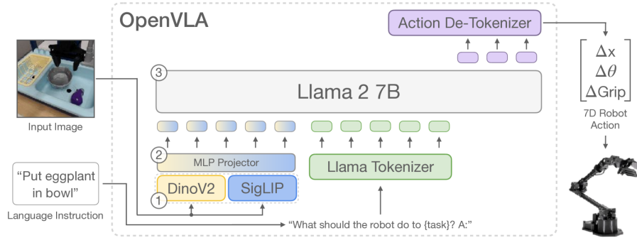
图 34: 图: OpenVLA 的数据通路。左侧输入是一张相机图和一句语言指令 “Put eggplant in bowl”；图像经 DinoV2 与 SigLIP 两个编码器并联，再过 MLP 投影成视觉 token，指令经 Llama Tokenizer 成文本 token，两串 token 拼在一起送进 Llama 2 7B；输出端的动作 token 经 Action De-Tokenizer 还原成 [\Delta x, \Delta \theta, \Delta Grip] 这样一个 7 维机器人动作。（图取自参考文献 [7]）
