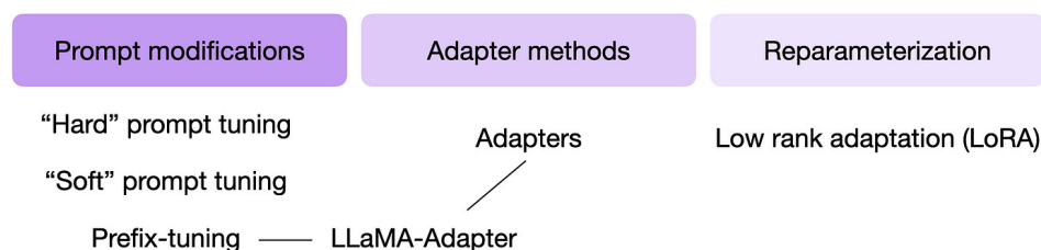
图 7: 图：三个并排的紫色标题条把常见 PEFT 方法分成三栏。Prompt modifications 栏下列着“Hard” prompt tuning、“Soft” prompt tuning 与 Prefix-tuning；Adapter methods 栏下列着 Adapters 与 LLaMA-Adapter，并有一条连线把 Prefix-tuning 与 LLaMA-Adapter 连起来；Reparameterization 栏下只有一项 Low rank adaptation (LoRA)
