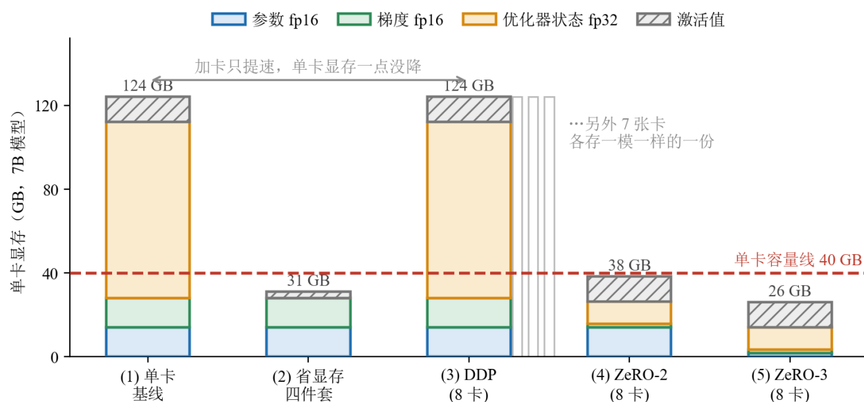
图 30: 图：一根 7B 模型的单卡显存柱，在五种方案下怎么变。柱子按 4.1.2 节四类吃货分段：参数 fp16 (蓝)、梯度 fp16 (绿)、优化器状态 fp32 (橙)、激活值 (斜纹灰)；红色虚线是标着 40 GB 的单卡容量线。(1) 单卡基线 124 GB，高高在线上；(2) 开省显存四件套后橙色的优化器状态整段消失 (搬到卡外)、斜纹的激活段被梯度检查点压扁，落到 31 GB；(3) DDP 那根柱子仍标着 124 GB，一条双向箭头从 (1) 拉到 (3)、上面写着“加卡只提速，单卡显存一点没降”，右侧几根灰柱注着“另外 7 张卡各存一模一样的一份”；(4) ZeRO-2 把梯度段和优化器段各切成 1/8，降到 38 GB；(5) ZeRO-3 把三段全部切成 1/8，降到 26 GB。图下一行注明：斜纹那段是激活值，随批量与序列长度变，图上只画一个示意高度，其余三段按 16 字节/参数精确折算 (本书自绘；分片按 8 卡算，与 4.4.6 节表里的公式一致)
