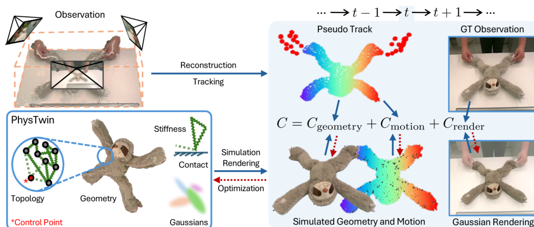
图 38: 图：左下角方框是 PhysTwin 的核心表示——一只软玩具，放大处画出连接质点的弹簧拓扑（红点为控制点），旁边挂着刚度、接触和三维高斯三组参数；左上角两台相机拍下真实视频，经重建与跟踪得到上排的伪轨迹，下排是仿真渲染出的几何与运动；两排之间的代价函数由几何项、运动项、渲染项三项相加，红色虚线箭头是回传的优化方向。（图出自参考文献 [41]）
