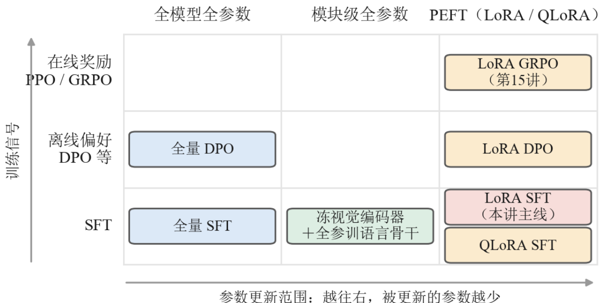
图 4: 图：一张三行三列的方法地图。列是参数更新范围——全模型全参数 / 模块级全参数 / PEFT (LoRA、QLoRA)，图下注明越往右被更新的参数越少；行是训练信号——自下而上为 SFT、离线偏好 DPO 等、在线奖励 PPO / GRPO。九个格子里有六格填着本讲提到的组合：左列是全量 SFT 与全量 DPO，中列只有“冻视觉编码器+全参训语言骨干”一格，右列自下而上是 LoRA SFT 与 QLoRA SFT (上下叠在同一格)、LoRA DPO、标着第 15 讲的 LoRA GRPO；红框那格 LoRA SFT 标着“本讲主线”。三个空格不是不能组合，只是本讲没走那条路（本书自绘）
