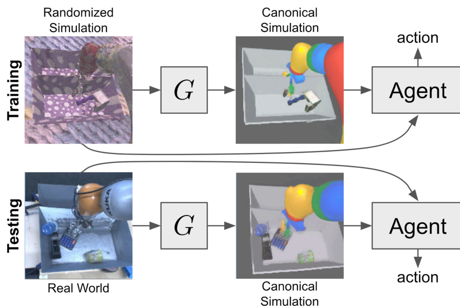
图 32: 图：上下两行结构完全相同，差别只在最左边那一格。上行“训练”从高度随机化的仿真图出发，下行“测试”从真机照片出发；两者都先过同一个生成器 G ，被翻译成同一套规范仿真外观（灰底、纯色积木、彩色机械臂），再送进同一个智能体输出动作。（图取自参考文献 [34]）
