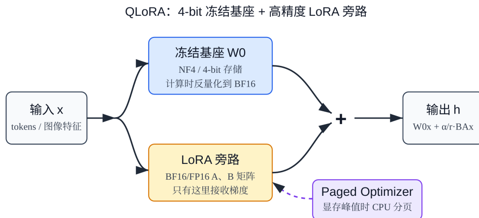
图 13: 图: 输入 x 分成两条支路——上支是冻结基座 W_0 , 标注为 NF4 / 4-bit 存储、计算时反量化到 BF16; 下支是 LoRA 旁路, 标注为 BF16/FP16 的 A 、 B 矩阵, 并注明“只有这里接收梯度”; 两支输出相加得到 h = W_0x + \frac{\alpha}{r}BAx 。右下角另有一个分页优化器方框, 用虚线指向 LoRA 旁路, 标注“显存峰值时 CPU 分页”
