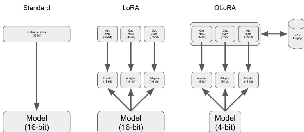
图 15: 图：标准微调、LoRA、QLoRA 三种方式的显存构成对照——基座权重、适配器与优化器状态各占多少、各处在什么精度
