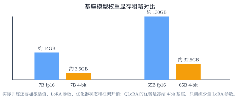
图 14: 图: 基座模型权重显存的粗略对比, 四根柱子分两组——7B 在 fp16 下约 14 GB、压到 4-bit 后约 3.5 GB; 65B 在 fp16 下约 130 GB、压到 4-bit 后约 32.5 GB (本书自绘; 四个数的来源是按 fp16 每参数 2 字节、4-bit 每参数 0.5 字节直接折算)
