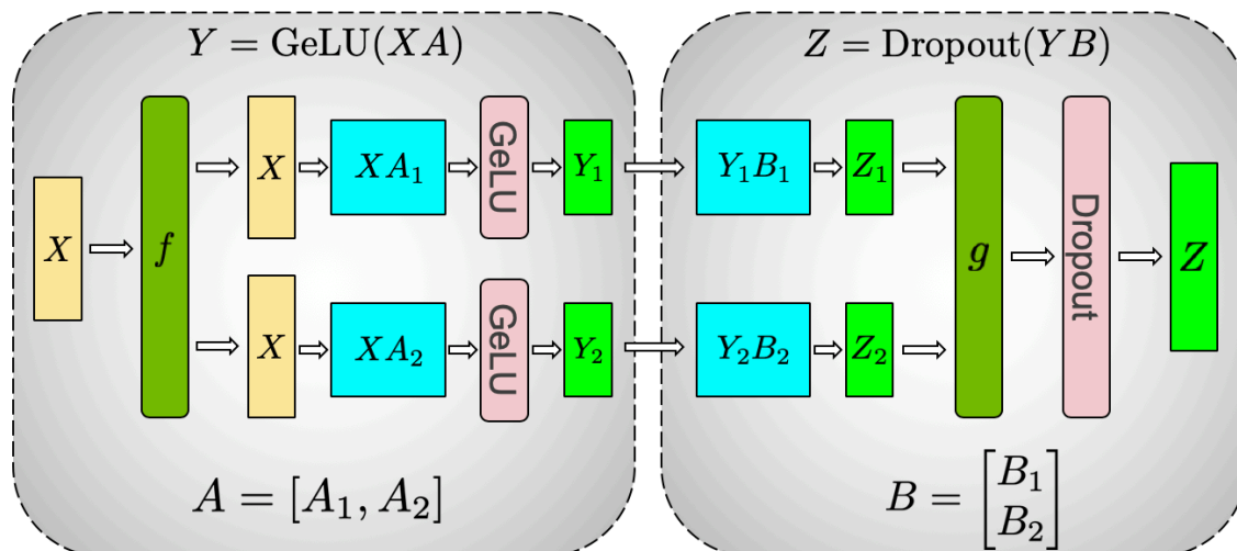
图 26: 图: Megatron 把 MLP 子层做张量并行的切法。第一个权重矩阵 A 按列切成 A_1 、 A_2 ，输入 X 完整复制给两条支路，各算 XA_1 、 XA_2 并各过一个 GeLU（逐元素激活，无需通信）；第二个权重矩阵 B 按行切成 B_1 、 B_2 ，两条支路各算 Y_1B_1 、 Y_2B_2 得到部分和，最后那个 g 把两个部分和规约（求和）成完整输出。整层只在末尾汇总处发生一次跨卡通信
