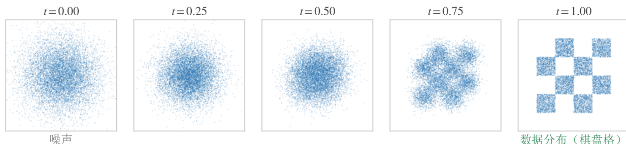
图 15: 五格从左到右是 t = 0, 0.25, 0.5, 0.75, 1 。 t = 0 是标准正态噪声， t = 1 是棋盘格数据分布，中间三格是 z_t = (1-t)z_0 + tz_1 的边际分布，注意结构不是最后一步突然出现的， t = 0.75 时格子的轮廓已经显形（直接按插值式采样画出解析的概率路径，未训练模型）
