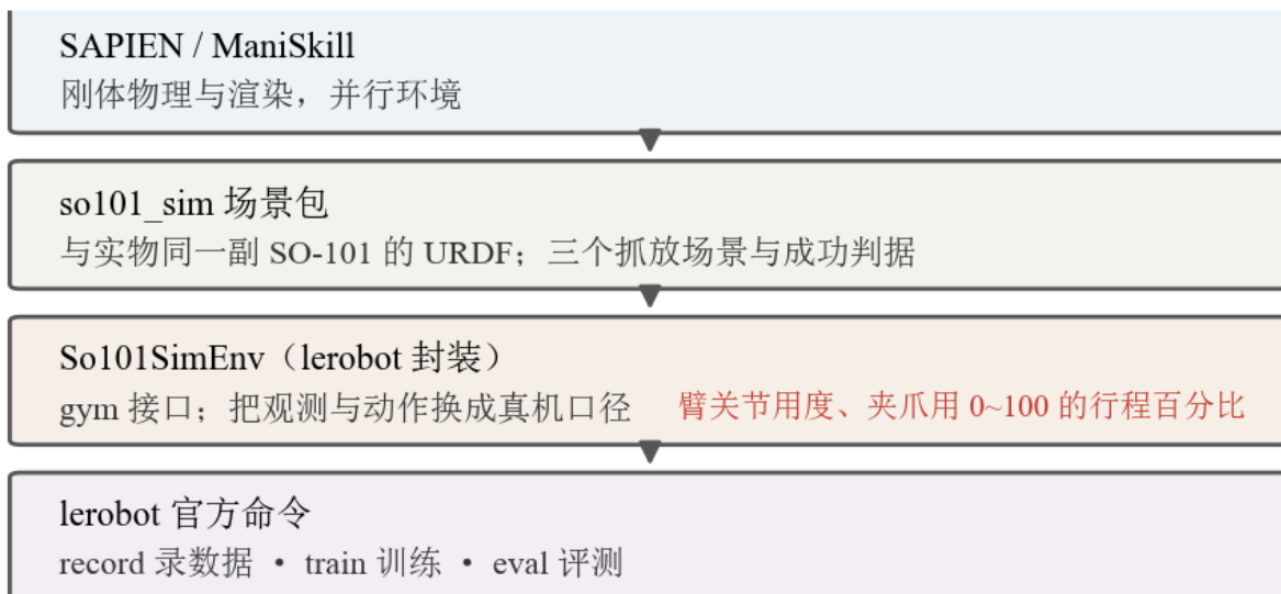
图 10: 四层自上而下：SAPIEN / ManiSkill 负责刚体物理与渲染、并行环境；so101_sim 场景包提供与实物同一副 SO-101 的 URDF、三个抓放场景与成功判据；So101SimEnv 是 lerobot 封装，给出 gym 接口并把观测与动作换成真机口径（臂关节用度、夹爪用 0~100 的行程百分比）；最下面是 lerobot 官方的 record / train / eval 三条命令
