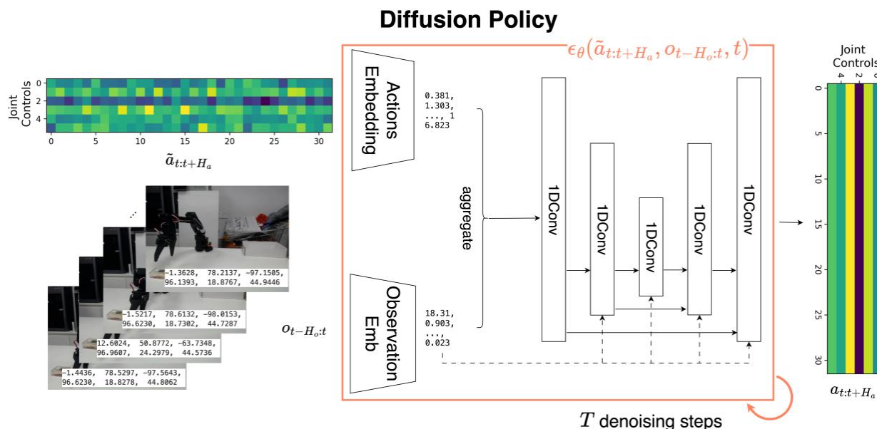
图 14: Diffusion Policy 的条件去噪架构示意
