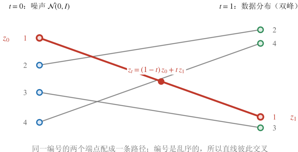
图 16: 左列是从噪声里采到的 4 个样本，右列是数据集里的 4 个样本（画成双峰）。 编号相同的两个端点配成一条条件路径 ，一共 4 条：每个噪声点各自连向一个数据点。编号是乱序的，所以这些直线彼此交叉，交叉正是「端点各自独立采样、随机配对」的后果。红色那条（编号 1）被高亮出来，标出 z_0 、 z_1 与它们之间的插值点 z_t
