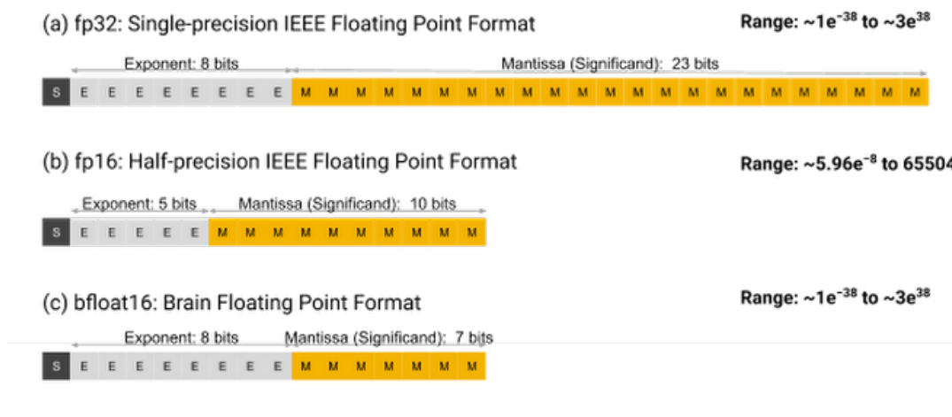
图 24: fp32 / fp16 / bf16 三种浮点格式的位宽与数值范围对比。fp32 用 8 位指数 + 23 位尾数，范围极宽、精度高；fp16 把指数压到 5 位，能表示的最小正数只到约 6 \times 10^{-8} ，范围窄得多；bfloat16 保留 8 位指数（范围和 fp32 一样宽）、只砍尾数到 7 位，用精度换范围
