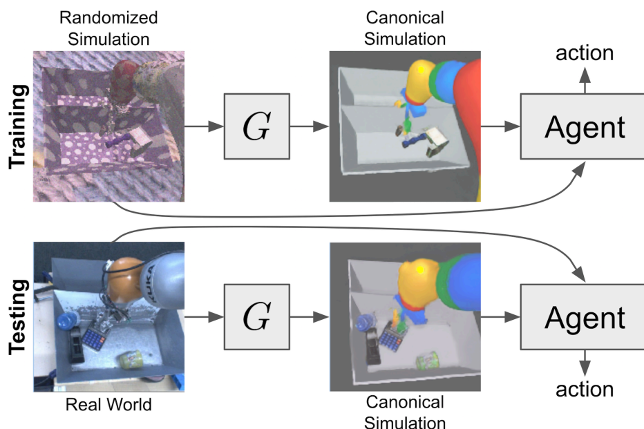
图 36: 上下两行结构完全相同，差别只在最左边那一格。上行“训练”从高度随机化的仿真图出发，下行“测试”从真机照片出发；两者都先过同一个生成器 G ，被翻译成同一套规范仿真外观（灰底、纯色积木、彩色机械臂），再送进同一个智能体输出动作。（图取自参考文献 [34]）
