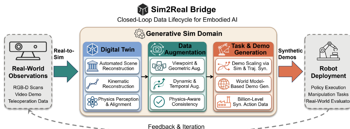
图 41: 中间橙色框是生成式仿真域，内含三列——数字孪生列（自动场景重建 / 运动学重建 / 物理感知与对齐）、数据增强列（视角与几何增强 / 动态与时序增强 / 物理一致性）、任务与示教生成列；左端真实观测（RGB-D 扫描、视频示教、遥操数据）经一支粗箭头进入，右端合成示教喂给真实机器人部署，底部一条虚线箭头从部署折返回真实观测。（图出自参考文献 [39] 图 9）
