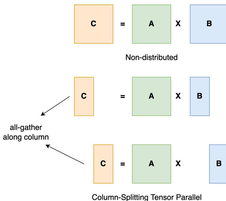
图 21: 模型并行 (张量并行) 示意: 上方是非分布式的整块矩阵乘 C = A \times B ; 下方是按列切分 (Column-Splitting) 后, 每张卡只算结果的一部分列, 再通过 all-gather 沿列方向把各卡的局部结果拼成完整的 C
