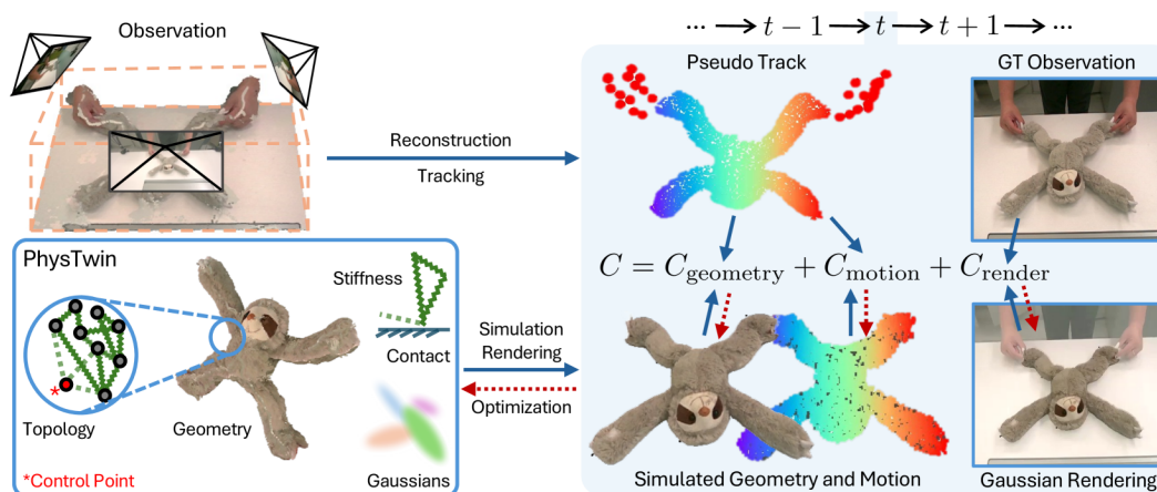
图 42: 左下角方框是 PhysTwin 的核心表示——一只软玩具，放大处画出连接质点的弹簧拓扑（红点为控制点），旁边挂着刚度、接触和三维高斯三组参数；左上角两台相机拍下真实视频，经重建与跟踪得到上排的伪轨迹，下排是仿真渲染出的几何与运动；两排之间的代价函数由几何项、运动项、渲染项三项相加，红色虚线箭头是回传的优化方向。（图出自参考文献 [41]）
