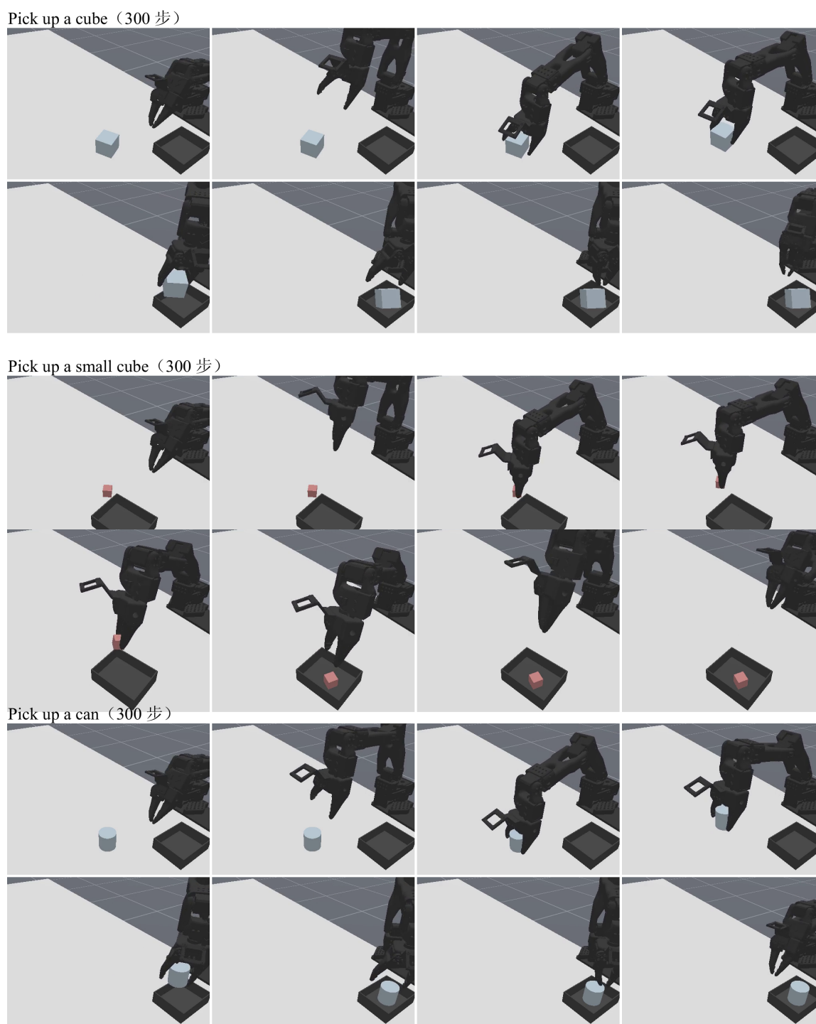
图 19: 三个任务各占两行（自上而下：方块、小方块、易拉罐），每个任务八帧走完一整个回合：初始位姿、夹爪降向物体、合拢夹住、抬起进入搬运、停在料箱上方、松手让物体落进箱、手臂退回、回到起始位姿
