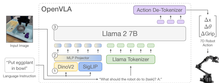
图 38: OpenVLA 的数据通路。左侧输入是一张相机图和一句语言指令“Put eggplant in bowl”；图像经 DinoV2 与 SigLIP 两个编码器并联，再过 MLP 投影成视觉 token，指令经 Llama Tokenizer 成文本 token，两串 token 拼在一起送进 Llama 2 7B；输出端的动作 token 经 Action De-Tokenizer 还原成 [\Delta x, \Delta \theta, \Delta \text{Grip}] 这样一个 7 维机器人动作。（图取自参考文献 [7]）
