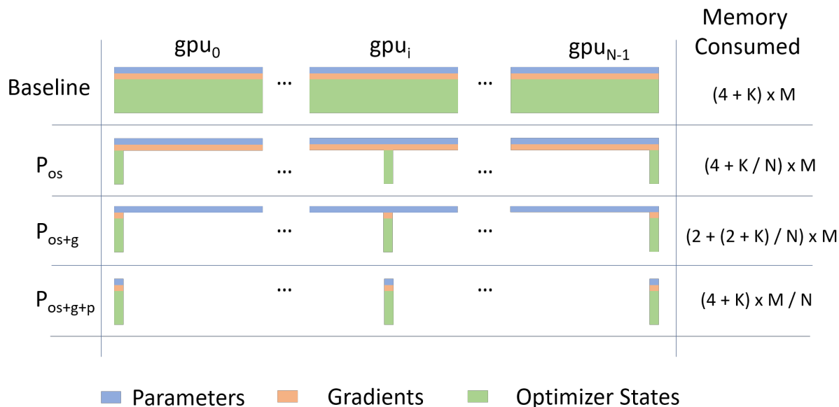
图 24: 图: ZeRO 三阶段分片对比。每一行是一种方案，横向从 gpu_0 到 gpu_{N-1} 是各张卡，柱子里蓝 = 参数、橙 = 梯度、绿 = 优化器状态。最上 Baseline（即 DDP）每张卡存满整份 (4 + K)\Psi ； P_{os} （Stage 1）只把绿色优化器状态沿各卡切开，每卡降到 (4 + K/N)\Psi ； P_{os+g} （Stage 2）再切橙色梯度，降到 (2 + (2 + K)/N)\Psi ； P_{os+g+p} （Stage 3）连蓝色参数也切，每卡只剩 (4 + K)\Psi/N 。图中 K 为优化器状态系数（混合精度 Adam K=12 ）， \Psi 为参数量， N 为数据并行度
