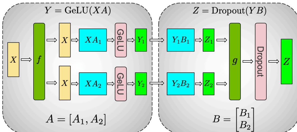
图 26: 图: Megatron 把 MLP 子层做张量并行的切法。第一个权重矩阵按列切成 A = [A_1, A_2] , 输入 X 完整复制给两条支路, 各算 XA_1 、 XA_2 并各过一个 \text{GeLU} (逐元素激活, 无需通信); 第二个权重矩阵按行切成 B = [B_1; B_2] , 两条支路各算 Y_1B_1 、 Y_2B_2 得到部分和, 最后那个 g 把两个部分和规约 (求和) 成完整输出。整层只在末尾汇总处发生一次跨卡通信
