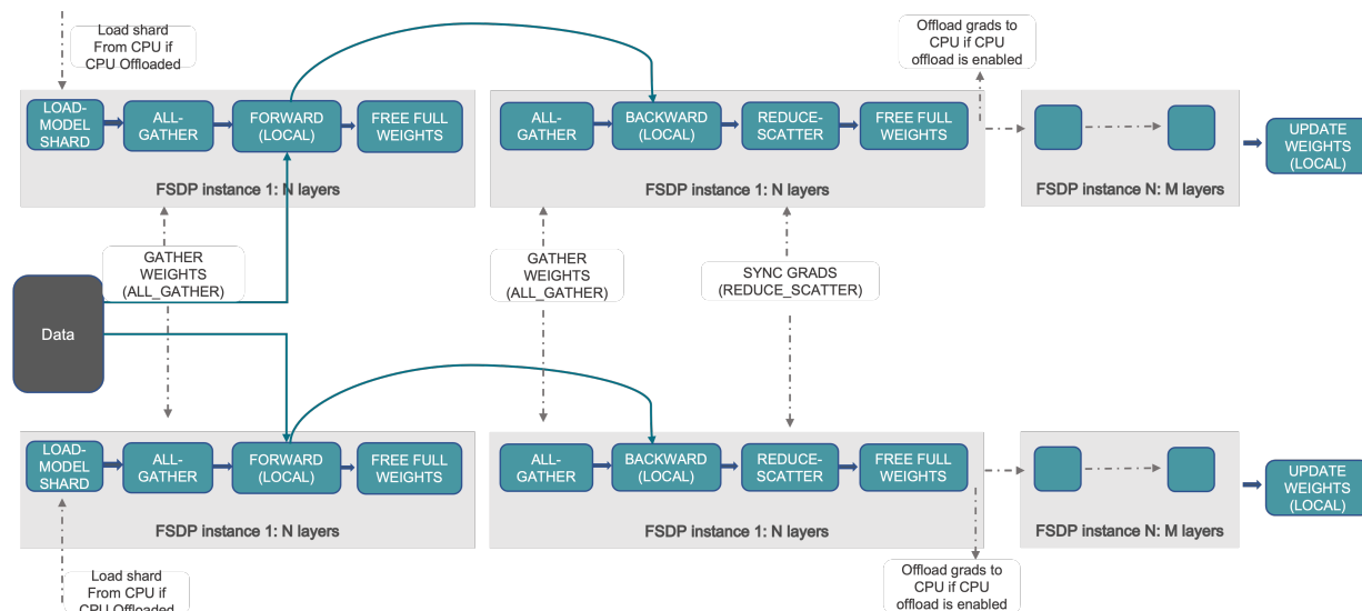
图 25: 图: FSDP 的一步训练 workflow。模型被切成若干 FSDP 单元（图中 FSDP Instance，通常按层/block 分组），每张卡只加载自己那份分片（load model shard）。前向时对当前单元 all-gather 出完整权重（gather weights）、算完该单元前向后释放掉非本地的那部分（free full weights）；反向同理先 all-gather 再算梯度，算完梯度用 reduce-scatter（sync grads）把规约后的梯度切片落到各卡；最后各卡只更新自己那一片参数（update weights）。若开启 offload，分片还能进一步搬到 CPU
