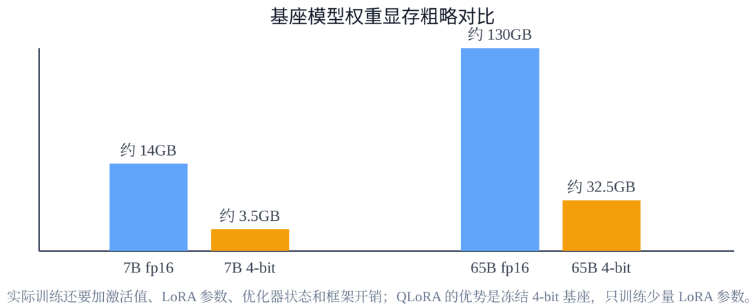
图 14: 图：QLoRA 显存对比
