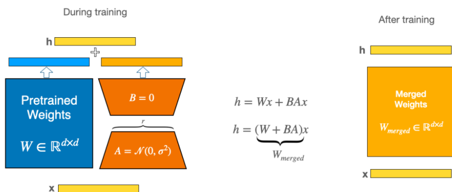
图 7: 图：LoRA 原理图
