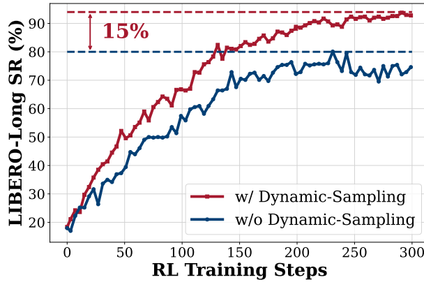
图 8: 三项探索增强策略的消融实验：动态采样、提高裁剪上界和提高 rollout 温度均带来显著提升
