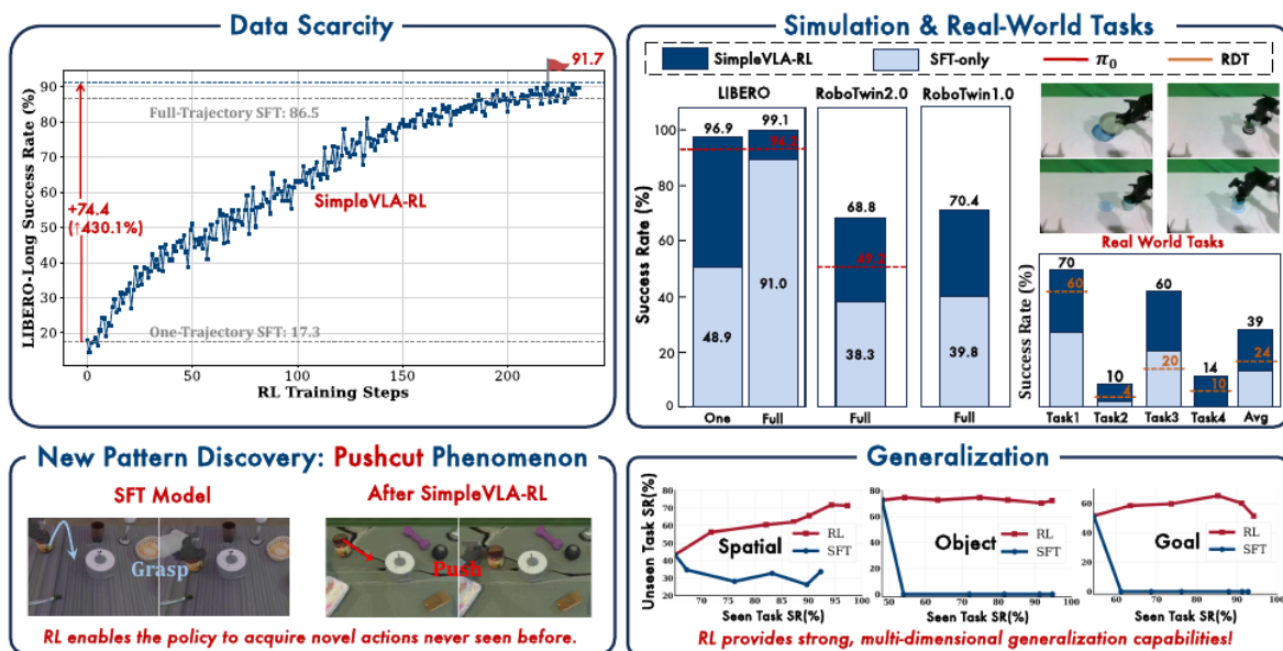
图 6: SimpleVLA-RL 总览：基于 veRL 构建的高效 VLA 在线强化学习框架，通过交互式轨迹采样、结果奖励和探索增强策略，在仿真和真实世界任务中显著提升 VLA 性能
