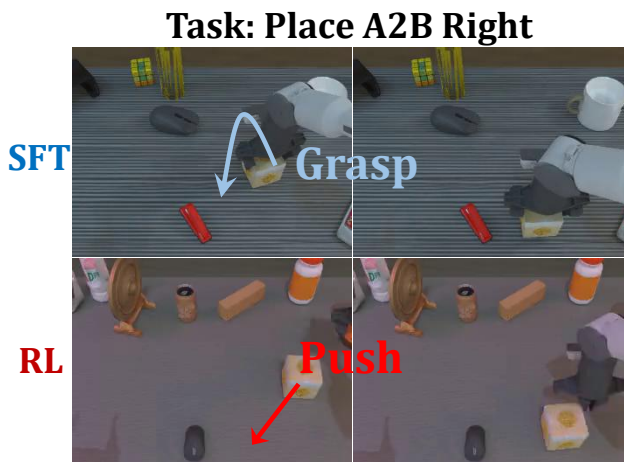
图 10: Pushcut 现象：RL 训练后模型自主发现了推动策略（下），而非示教数据中的抓取-移动-放置策略（上）
