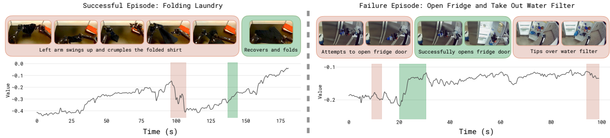
图 16: 价值函数可视化：左侧是成功的叠衣服任务，右侧是失败的操作任务。红色部分表示价值下降（犯错），绿色部分表示价值上升（进展顺利）。价值函数能正确识别 episode 中的错误和进展速度
