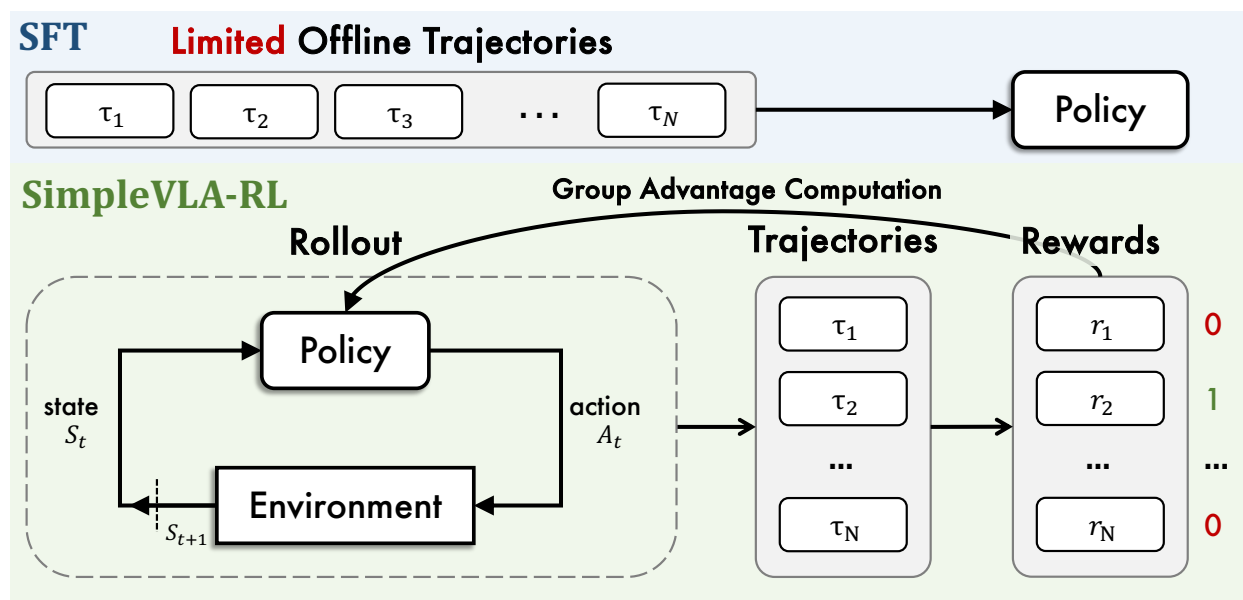
图 7: SimpleVLA-RL 框架总览：从交互式 VLA rollout 到 GRPO 策略更新的完整流程
