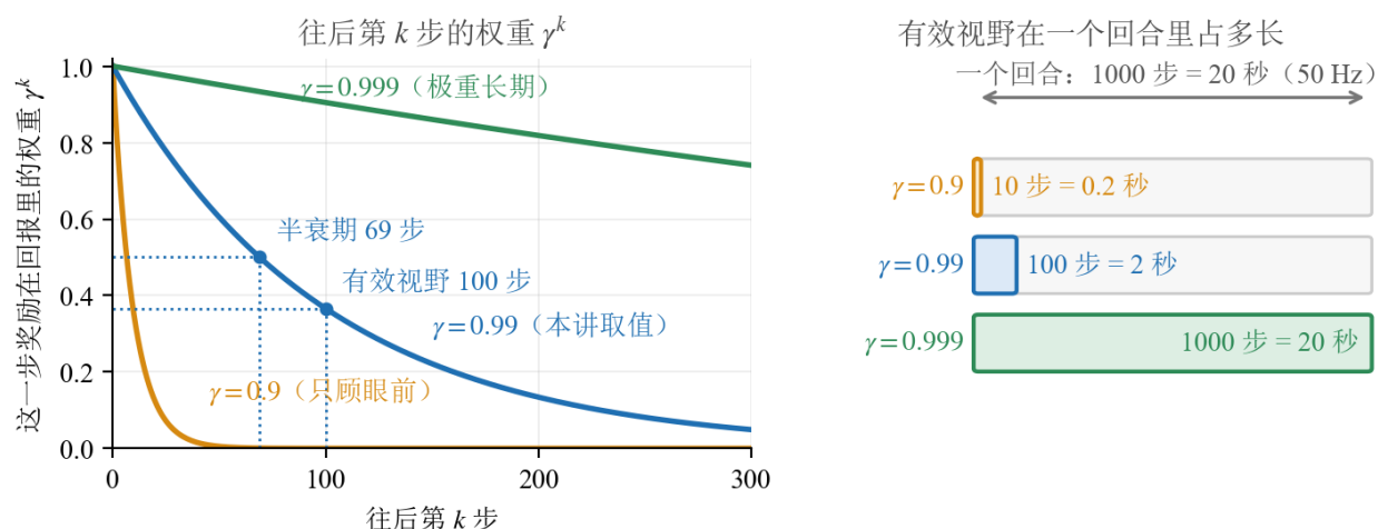
图 3: \gamma 决定未来的奖励还剩多少分量。左: 三个 \gamma 取值下, 往后第 k 步的奖励在回报里还剩多少权重。本讲取 \gamma = 0.99 , 半衰期约 69 步 ( 0.99^{69} \approx 0.5 ), 有效视野 1/(1-\gamma) = 100 步 (此处权重已降到 0.99^{100} \approx 0.37 )。右: 同样三个 \gamma 的有效视野贴到一整个回合上——mjlab 的 G1 速度跟随环境仿真步长 0.005 秒、每 4 步出一次动作, 即 50 Hz, 回合上限 20 秒 [7], 一个回合正好 1000 步
