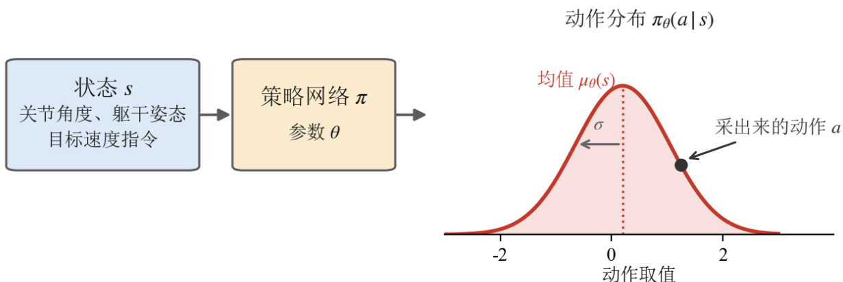
图 4: 策略把状态映射成的是一个 动作分布 , 不是一个定值: 左边是输入 (关节角度、躯干姿态、目标速度指令), 中间是参数为 \theta 的网络, 右边是它吐出来的高斯密度——峰值处的均值 \mu_{\theta}(s) 是“最想做的动作”, 从均值往外量出去的那一段 \sigma 就是探索强度, 黑点是这一步真正采出来去执行的那个 a 。 \sigma 越宽, 采到离均值远的动作的机会越大
