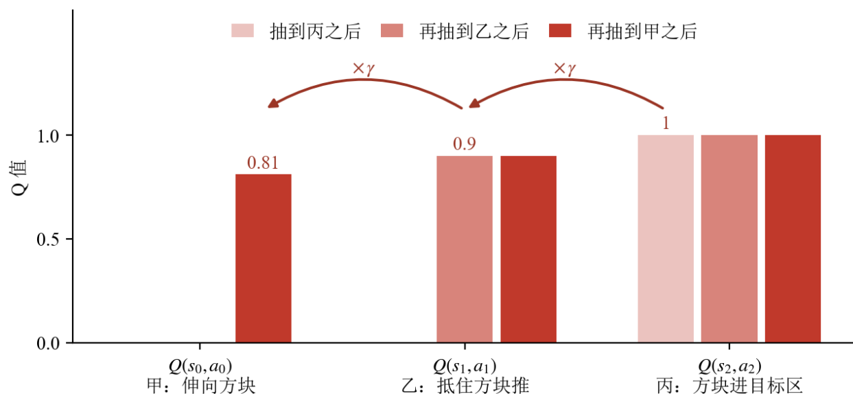
图 2: 一个终点奖励沿转移链回传成价值坡道：抽到丙记住成功，再抽到乙、甲时价值按 \gamma 折扣逐格子起点传播。 \gamma = 0.9 ，起点三个 Q 全为 0
