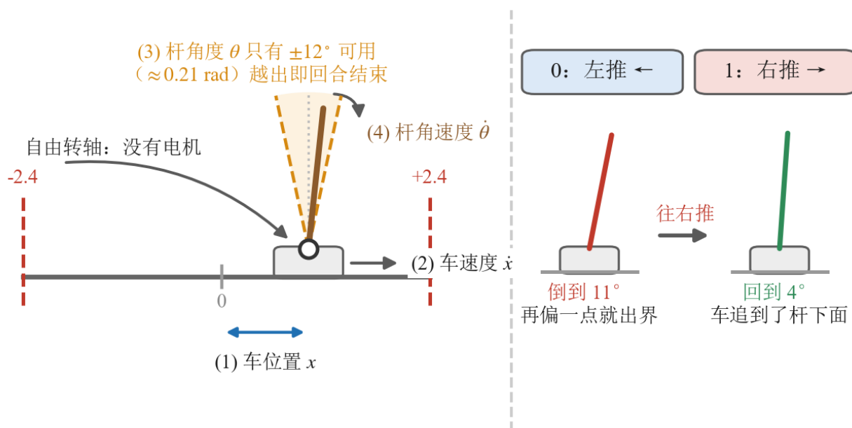
图 4: CartPole 的两道终止线与那个反直觉的动作方向。左半把上面四条要素画进同一个场景：红色虚线是轨道两端的 \pm 2.4 ，越过就出界；橙色扇形是竖直方向左右各 12^\circ ( 0.21 \text{ rad} ) 的可用范围，杆尖越出扇形回合当场结束——两道线卡的不是同一件事，一道管车能滑多远、一道管杆能歪多少。车顶那个白心圆是 自由转轴 ，没有电机，杆只受重力和车身加速度摆布。(1)(2)(3)(4) 分别标出四个观测各自对应的物理量。右半是那一下反直觉的动作：杆已经倒到 11^\circ ，正确的做法是把车也 往右推 ，让车追到杆的正下方，杆才回正；往左“顶回去”只会让它倒得更快。动作只有 0 / 1 两档，没有“不动”这一档
