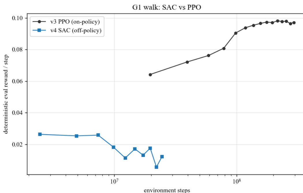
图 9: 按环境步数对齐的 reward 曲线（横轴对数刻度）：SAC 整段曲线都落在图的左侧，最高点就在最早的存档点（246 万步、0.026），此后逐级下滑；PPO 的第一个存档点要到 2000 万步，此后一路爬到 0.098 的平台。数据来源是 G1 行走模块 result 目录下的 compare.json
