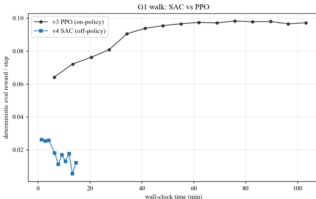
图 10: 按墙钟时间对齐的 reward 曲线，横轴换成训练用掉的分钟数，两条线仍是 SAC 与 PPO：跑满 3000 次迭代，SAC 约 15 分钟、PPO 约 103 分钟；SAC 那条在头 4 分钟里就走完了全部涨幅，剩下的 11 分钟一路往下走
