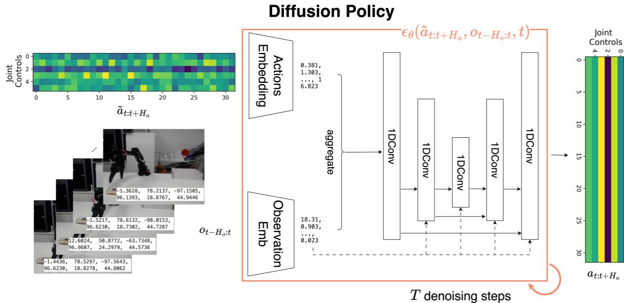
图 13: Diffusion Policy 的条件去噪架构示意
