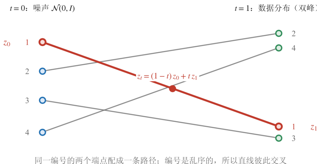
图 15: 左列是从噪声里采到的 4 个样本，右列是数据集里的 4 个样本（画成双峰）。 编号相同的两个端点配成一条条件路径 ，一共 4 条：每个噪声点各自连向一个数据点。编号是乱序的，所以这些直线彼此交叉，交叉正是「端点各自独立采样、随机配对」的后果。红色那条（编号 1）被高亮出来，标出 z_0 、 z_1 与它们之间的插值点 z_t
