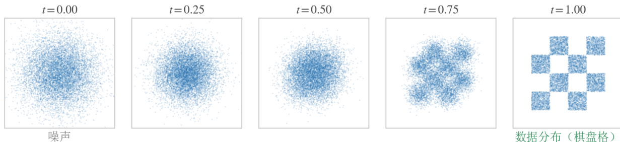
图 14: 五格从左到右是 t = 0, 0.25, 0.5, 0.75, 1 。 t = 0 是标准正态噪声， t = 1 是棋盘格数据分布，中间三格是 z_t = (1-t)z_0 + tz_1 的边际分布，注意结构不是最后一步突然出现的， t = 0.75 时格子的轮廓已经显形（直接按插值式采样画出解析的概率路径，未训练模型）
