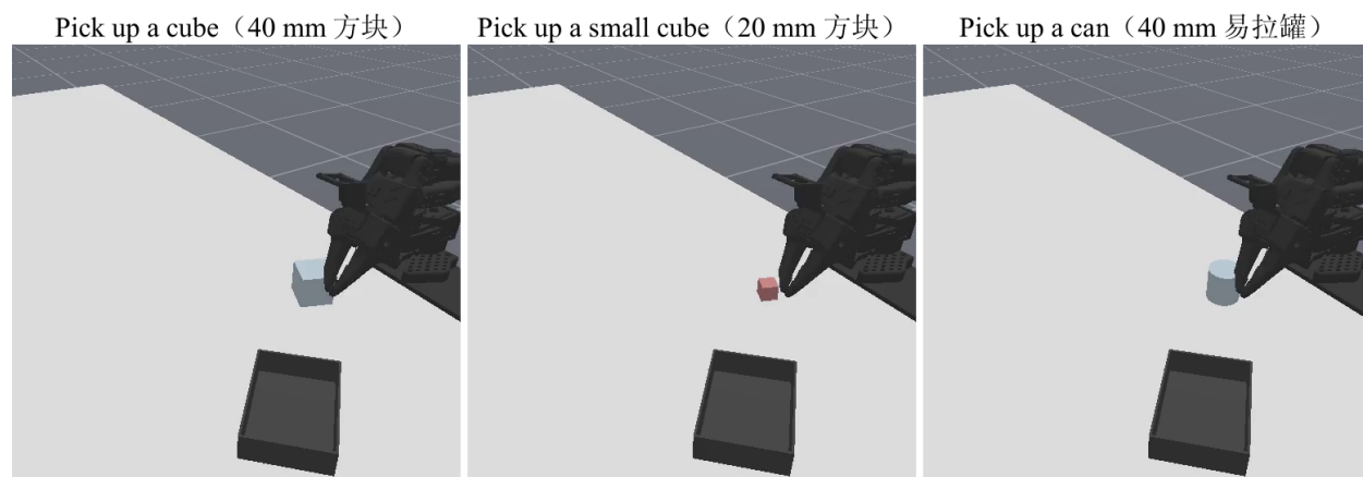
图 11: 三个仿真场景的初始画面并排, 自左向右分别是 40 mm 方块、20 mm 方块、40 mm 易拉罐; 每格里机械臂在右侧起始位姿, 物体在爪前, 料箱在桌面靠前处
