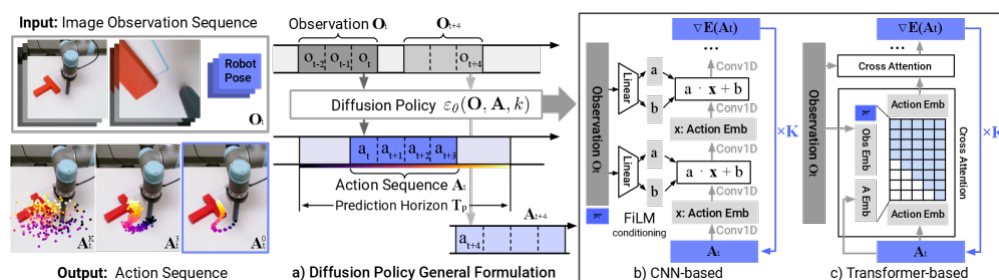
图 32: 图：将动作建模为去噪过程，能够表达多模态动作分布、稳定训练、容易扩展到高维连续动作空间。
