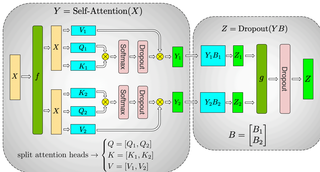
图 27: 图：注意力子层的张量并行：多头注意力按头切到两张卡，卡 1 负责一组头的 Q_1, K_1, V_1 、卡 2 负责另一组 Q_2, K_2, V_2 ，各自独立完成 \text{Softmax} 与加权（图中两条并行支路互不通信），输出投影矩阵 B 按行切，末尾 g 把两路部分和规约成完整输出。和 MLP 一样，整层前向只在出口通信一次
