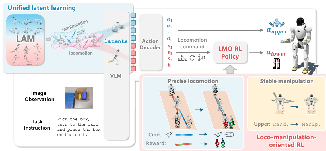
图 16: WholeBodyVLA 总览：从无动作视频里学潜在动作监督，VLA 同时预测操作与移动潜在码，轻量解码器落成上肢动作和下肢指令
