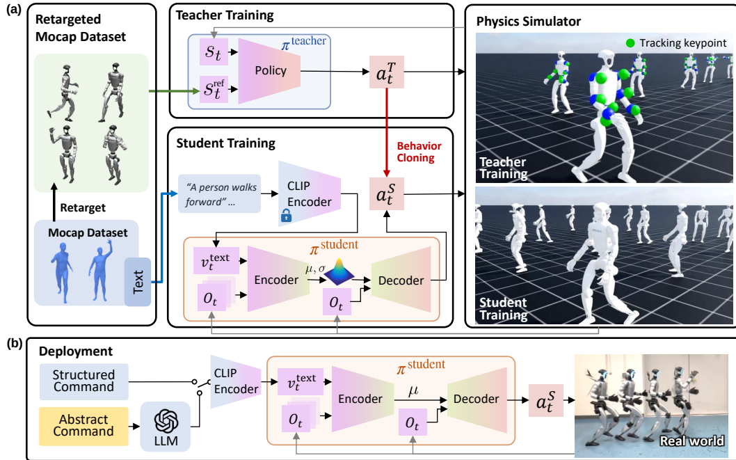
图 10: LangWBC 两阶段框架：先训练只会跟踪的 Teacher，再蒸馏成以语言为条件、只靠本体感知运行的 CVAE Student
