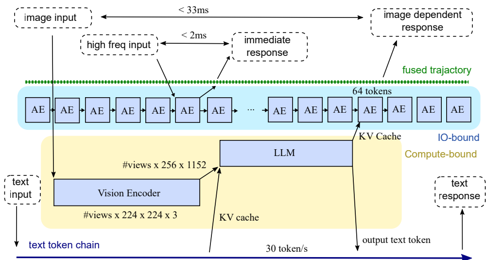
图 5: Full Streaming Inference：大模型慢回路看场景、Action Expert 快回路出轨迹，并发跑出三层不同频率
