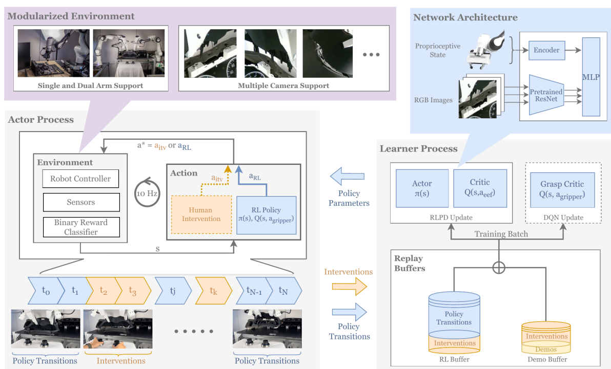
图 12: HIL-SERL 系统架构: actor 进程与环境实时交互并接受人工干预, learner 进程从双 replay buffer 采样更新, 两者异步通信
