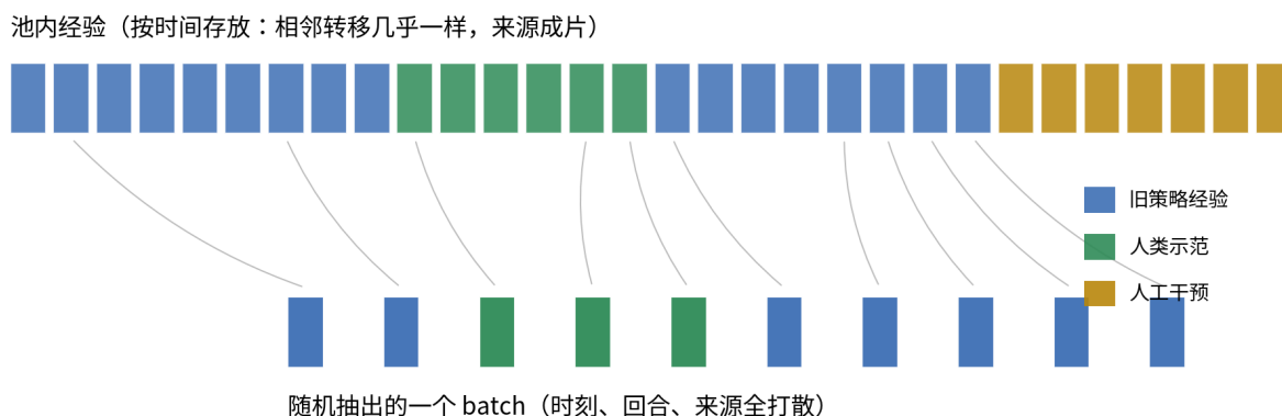
图 2: 经验池的存与取：上排为按时间存放的池内转移（来源成片、相邻相关），下排为随机抽出的一个 batch（时刻与来源全打散）
