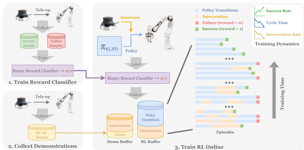
图 14: HIL-SERL 训练流程：先遥操采正负样本训练奖励分类器，再采集示范装入 demo buffer，最后在线训练并逐步减少人工干预
