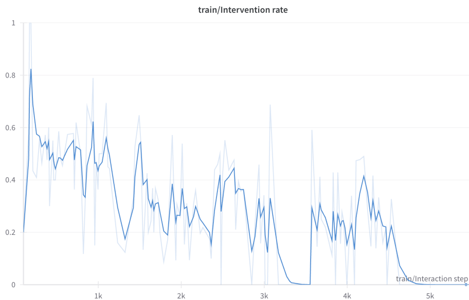
图 18: 一次健康训练的干预率曲线：随策略改善从高位持续下降
