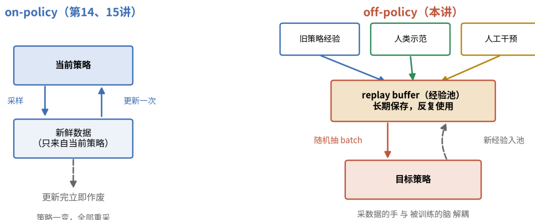
图 1: on-policy 与 off-policy 的数据流对比：左侧数据只来自当前策略、用一次即弃；右侧多来源经验汇入经验池、长期反复使用
