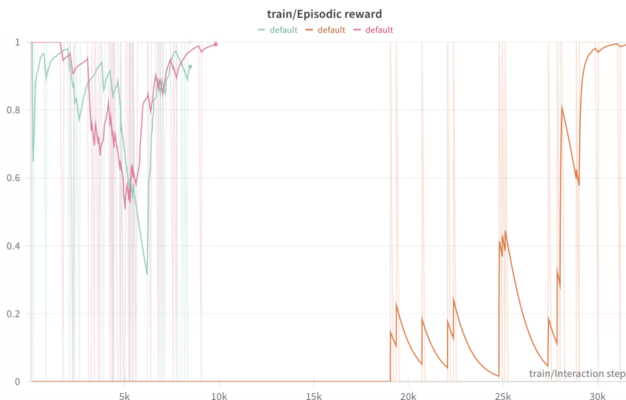
图 17: 人工干预对学习速度的影响：无干预的训练（橙）远迟于有干预的两组（粉、蓝）达到最高回报
