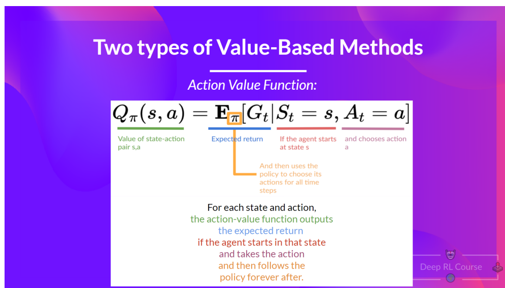
图 3: 动作价值函数 Q_\pi(s, a) 的定义逐段标注：在状态 s 选动作 a 、之后跟随策略 \pi 的期望回报
