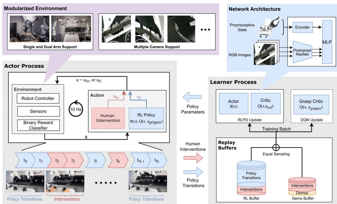
图 13: LeRobot 版 HIL-SERL 工作流：示范与奖励分类器打底，actor 进程在真机上执行并接受干预，learner 进程异步更新策略
