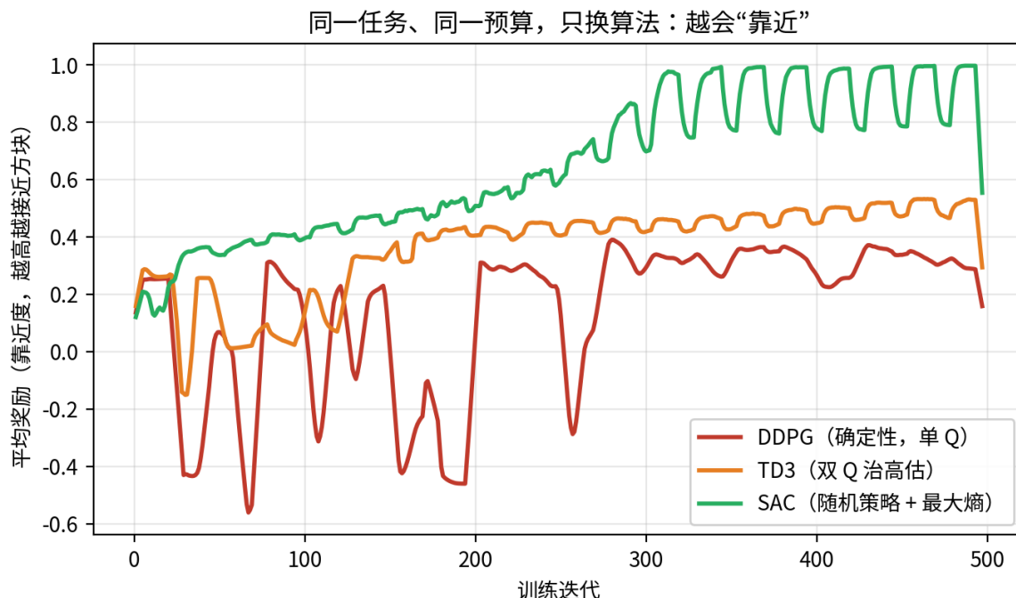
图 8: 同一任务、同一预算 (500 次迭代), 只换算法: DDPG (红) 剧烈震荡卡在低位, TD3 (橙) 稳住并爬到更高, SAC (绿) 稳步登顶。纵轴平均奖励是“靠近度”的代理——越高表示末端越接近方块
