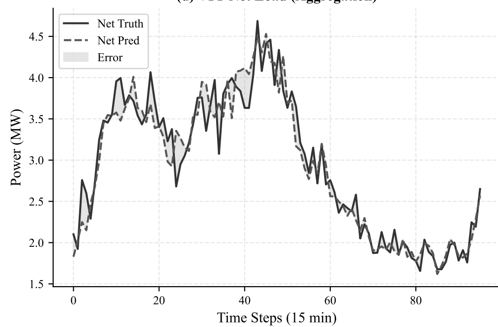
(d) VPP Net Load (Aggregation)
