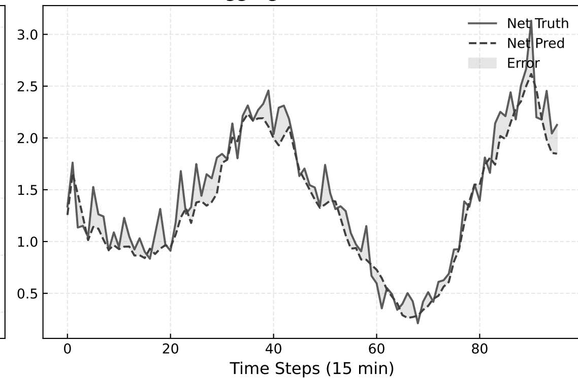
(d) VPP Net Load (Aggregation)
