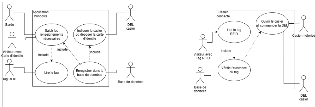
FIGURE 2 – Diagramme de cas d'utilisation
