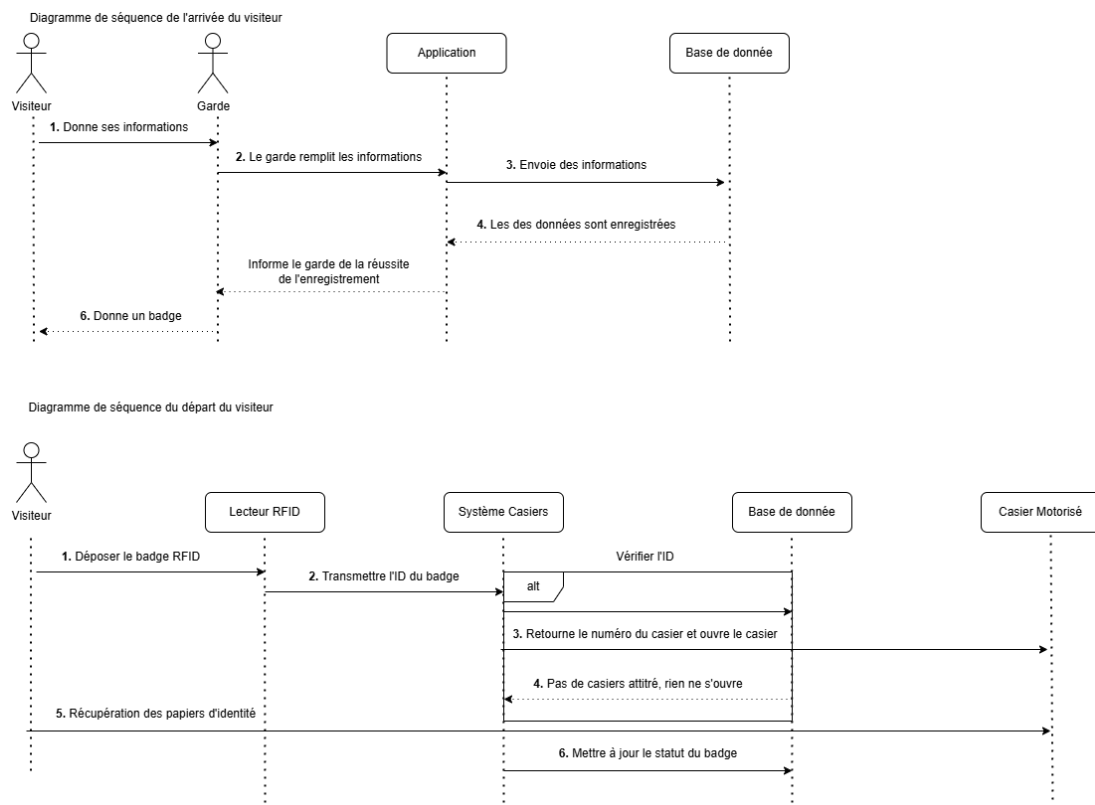
FIGURE 5 – Diagramme de séquences
