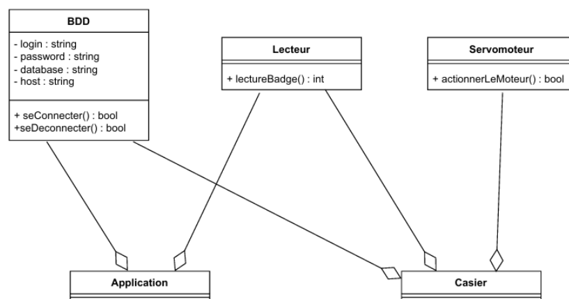
FIGURE 3 – Diagramme de classe
