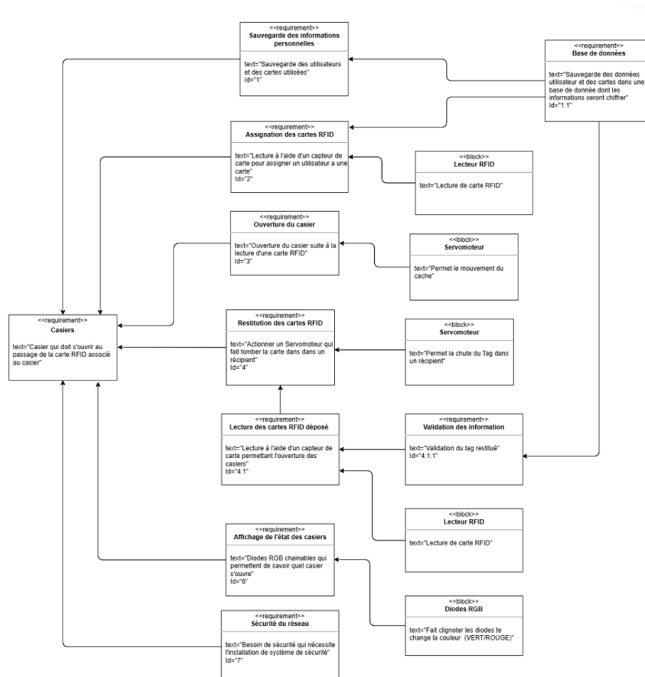
FIGURE 1 – Diagramme d'exigence
