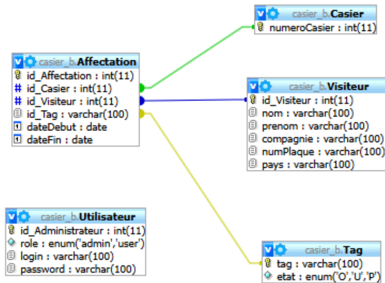
FIGURE 4 – Base de données
