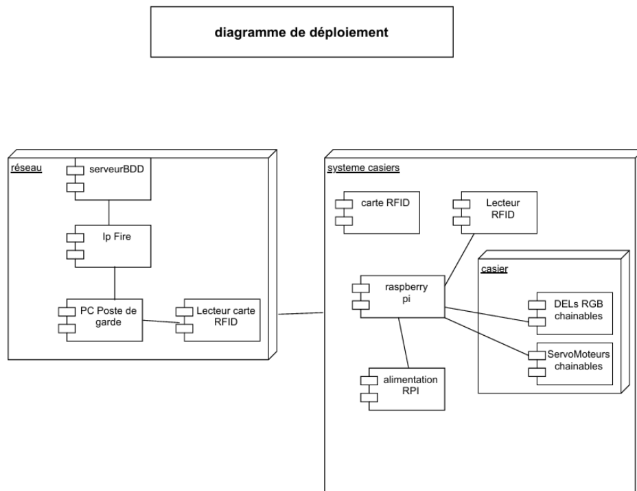
FIGURE 6 – Diagramme de déploiement
