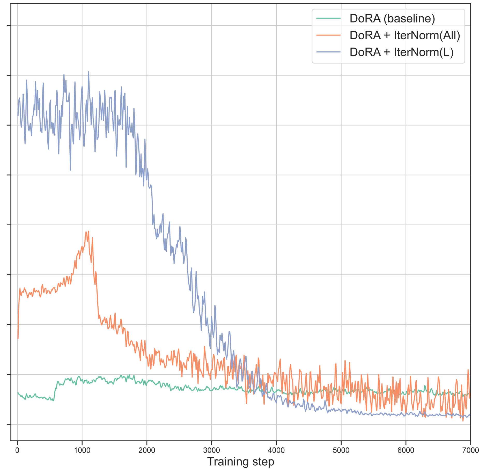
Method: DoRA
