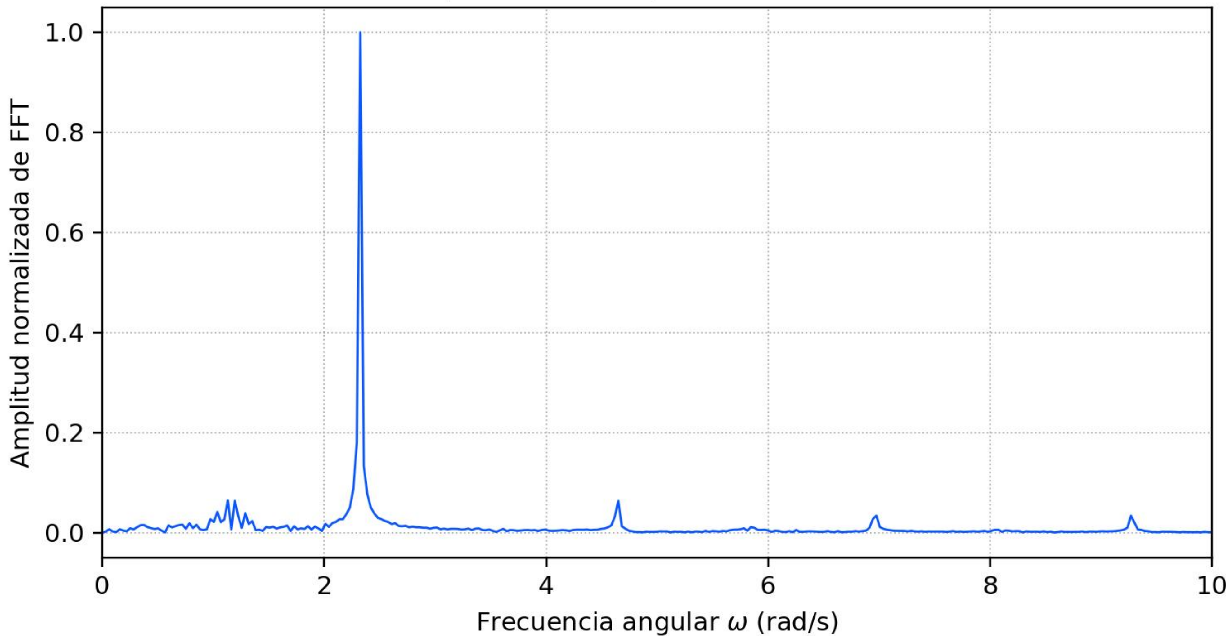
Espectro de Amplitud FFT de x(t)
