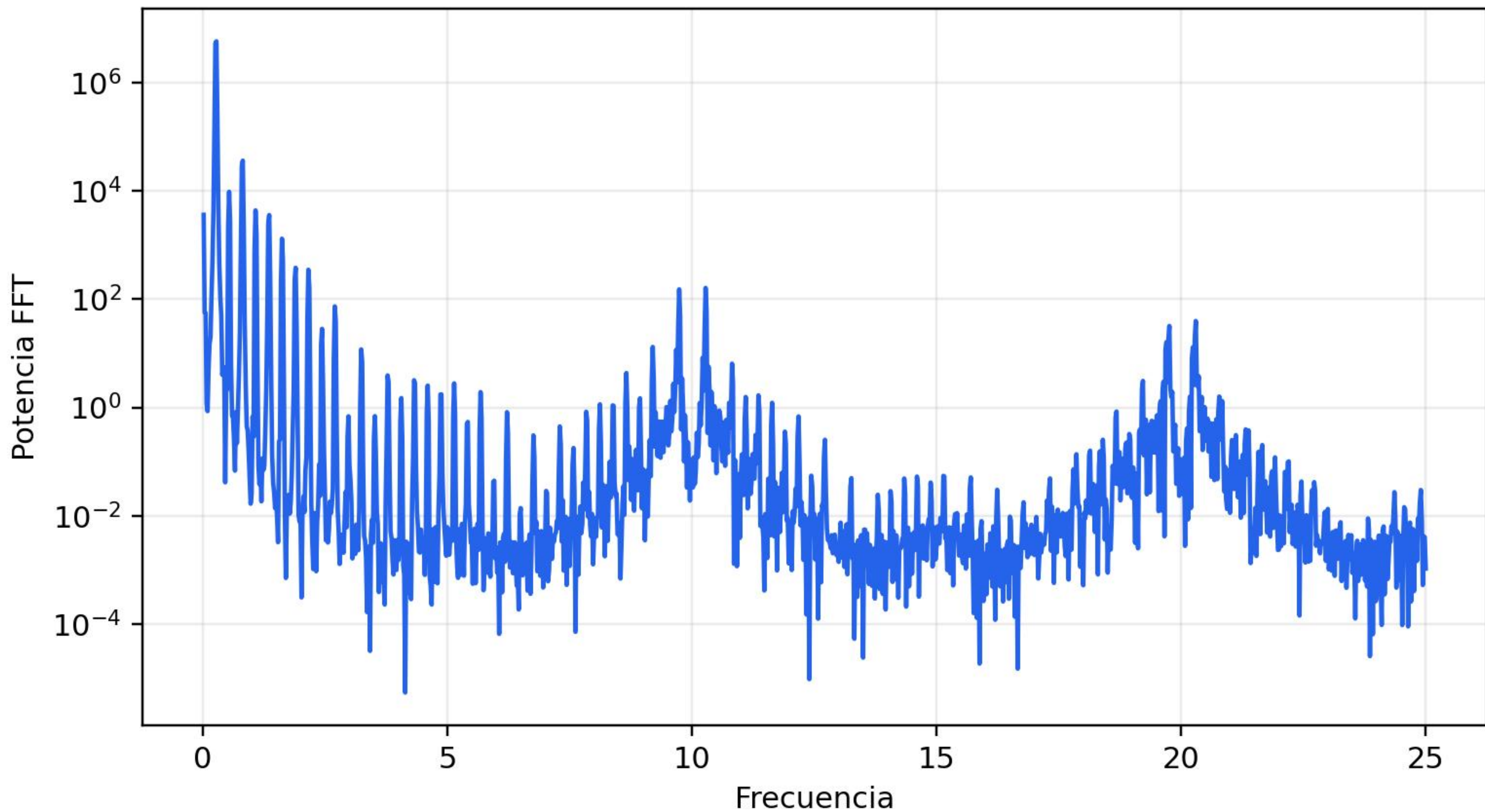
Espectro de x(t) , trayectoria EFORK-3 C
