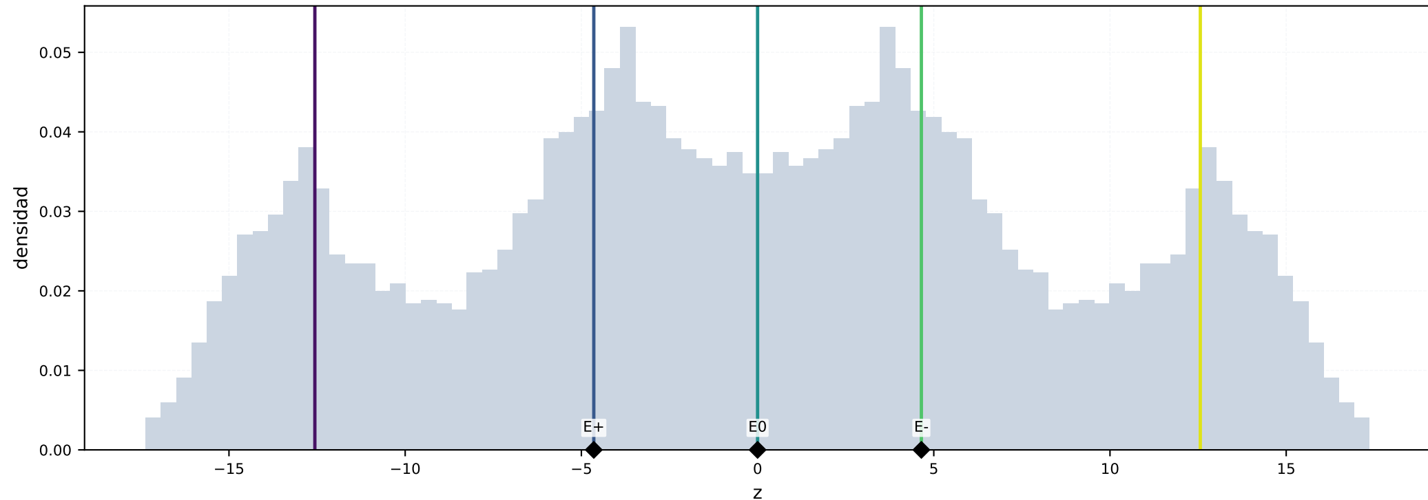
Selección no arbitraria de cortes z — Chua arctangente c590, q=0.9999
