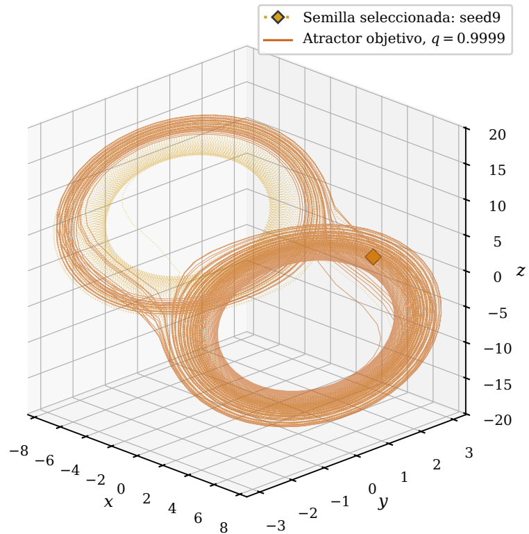
PVI fraccionario desde seed9
