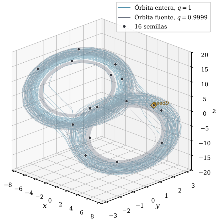
Órbita fuente y selección de semillas
