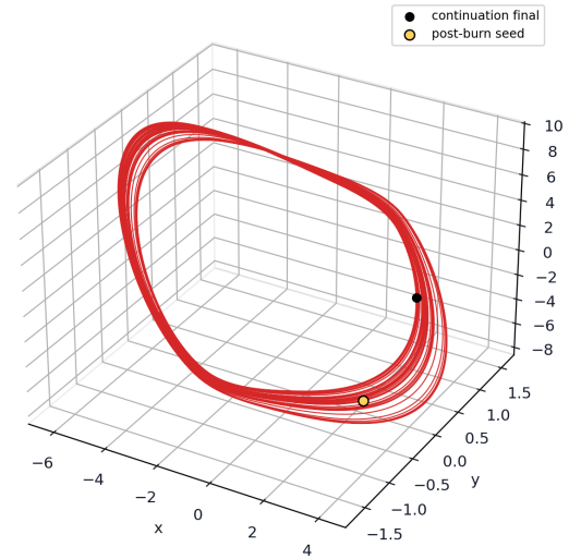
Figura 3. Atractor candidato obtenido al finalizar la continuación y eliminar el transitorio. El punto negro corresponde al estado final de continuación y el punto amarillo a la semilla efectiva X_{target} .
