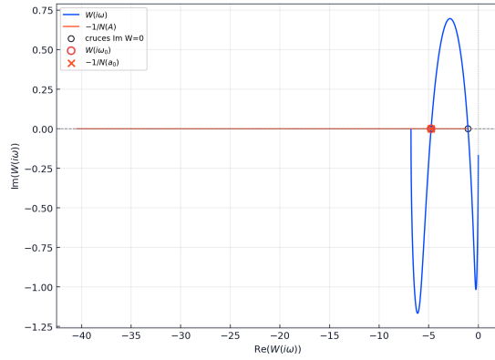
Figura 1. Diagrama de Nyquist del bloque lineal y punto de cierre armónico asociado con la función descriptiva. La coincidencia entre W(i\omega_0) y -1/N(a_0) valida numéricamente la semilla armónica.
