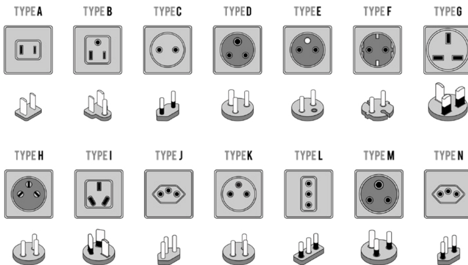
Imagen 2. Types of plugs and sockets
