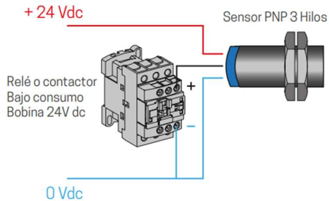
Cableado PNP 3 Hilos
