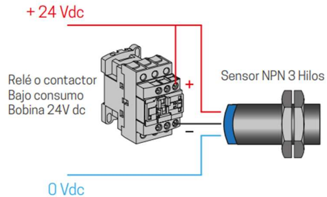
Cableado NPN 3 Hilos
