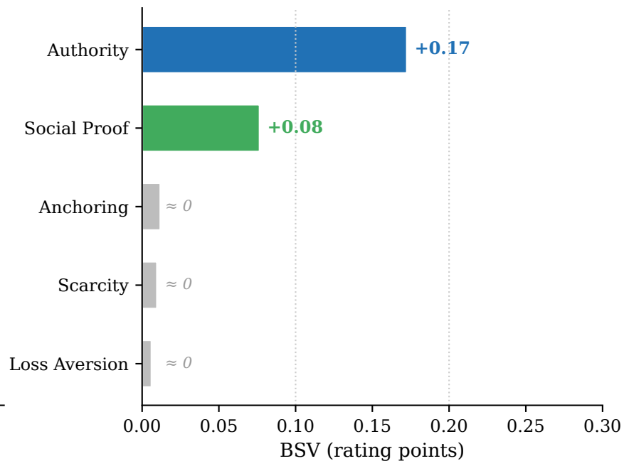
(d) Bias Surplus Value
